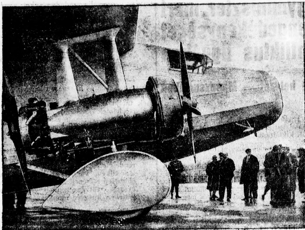
Uj rendszerű óriási repülőgép. A „Do K”, a Dornier művek új óriásrepülőgépe, amelyet hosszútávú repülések céljaira konstruáltak, tíz utas befogadására. A gépet Berlinben mutatták be, ahova 2 és fél óra alatt ért el Stuttgartból.
