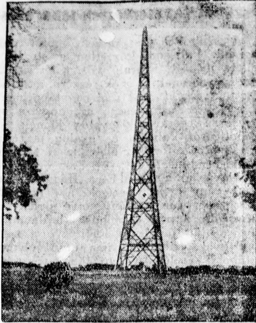
Száznegyven méter magas fatorony. Breslau mellett most készítették el a rothsürbeni leadóállomás nagy tornyát, amely egészen fakonstruktóióból készült. A torony 140 méter magas.
