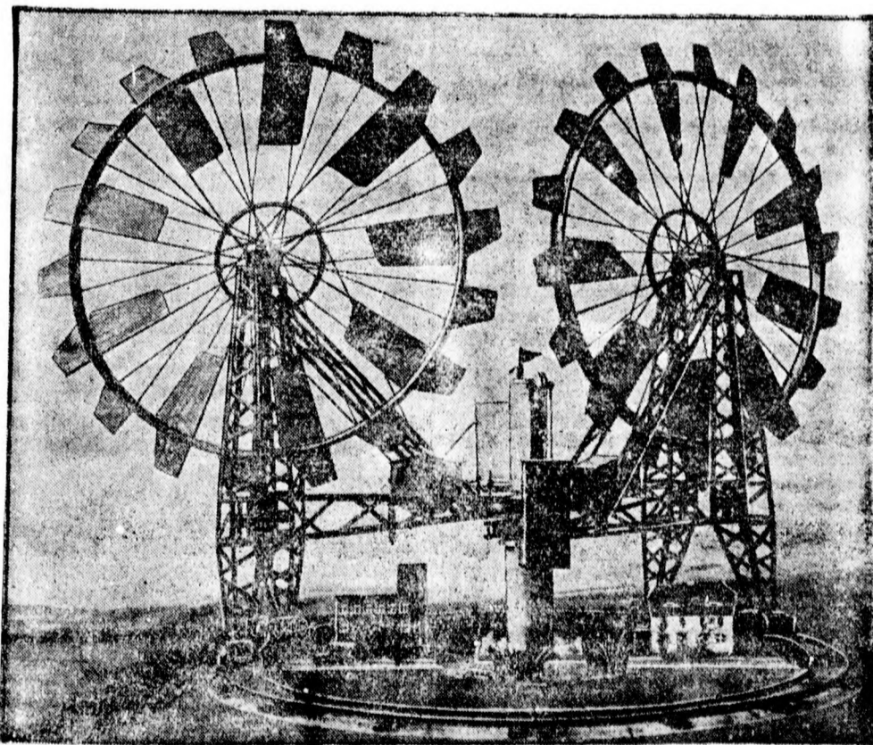
Bendmann Dáca iránklurú mérnök szenzációs találmánya. Bendmann mérnök a képi kőn bemutatott triási légturbinát tervezte, amelynek a hajtóerőt a szél szolgáltatja. A találmány lényege egy 80 méter átmérőjű örsinpálya, amelyen két, egyenként 200 méter magas torony van. A tornyok hatalmas szélfogó kerekekkel vannak ellátva, amelyek automatikusan állnak be a szél lökőereje irányába. A légturbina 2 millió márkába kerül.
