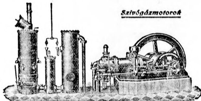
Felfűtéses, generátorral ellátott 30-400 lóerős nagyságu SZŐRGÁZ-MOTORUNK van az Önök részére. - A lassújárati jező-motorok L. LANG legelső, legöregebb gépgyárból valók.
