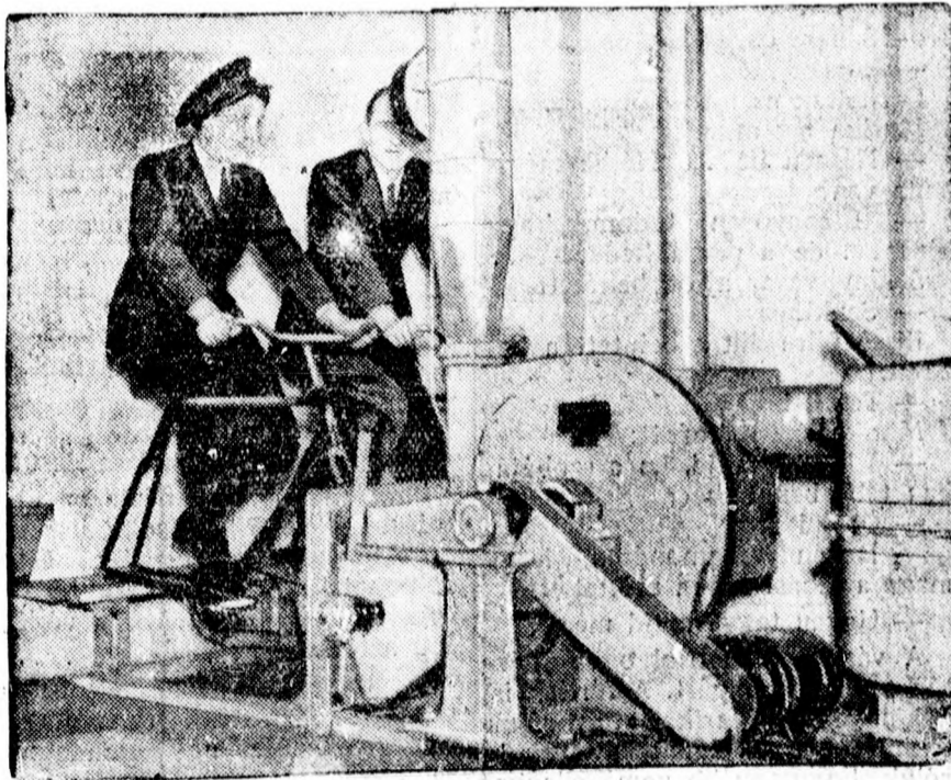
LÁBHAJTÁSOS LEVEGŐ TISZTÍTÁS EGY LÉGVÉDELMI PINCÉBEN. Egy londoni nagybank légvédelmi pincéit építették és ebben újfajta levegő tisztító készülékeket szerelt fel, amelyeket lábhajtással lehet üzemben tartani.
