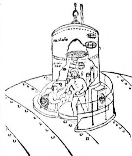
Az elsüllyedt tengeraltjáró csapóajtójához szerített búvárharang keresztmetszetének vázlatos rajza. (Az emberalakok az áttekinthetőség kedvéért aránytalanul nagyok.)
