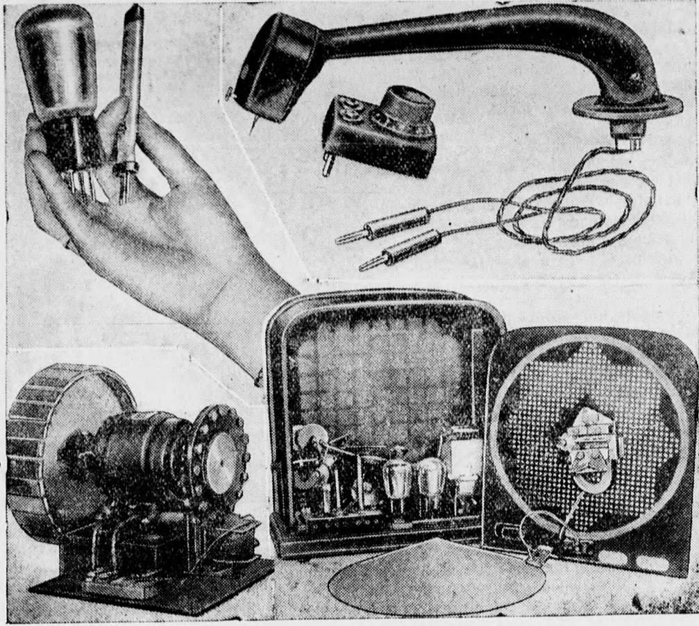
A berlini rádiókiállítás szenzációi: az eddigieknél tízszer kisebb rádiólámpa, érzékeny rádiogramofontű, tükrökészülék távolbalátóhoz és kis dobozba épített hangszórós hálózati rádió.
