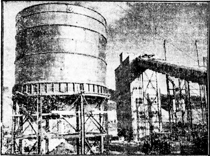
A kujbisevi vízierőmű építkezése télen sem szünetel. Hatalmas mértékben segíti a téli építési munkálatokat az újonnan épült automatizált betongyár, amely naponta több ezer köbméter betonnal segíti a világ legnagyobb vízierőművének határidőelőlti elkészülését.
