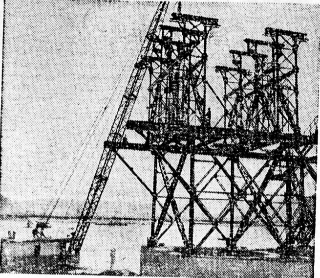
A képen: vázak szerelése a Volga partján, a kujbisevi vízerőmű építkezésén. (Foto: Sz. Kropivnyockij.)
