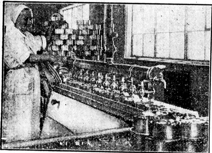
A képen: automata olajtöltőgép a ventspili halfeldolgozó kombinátuban. (Lett SZSZK). Foto: A. Agapov.
