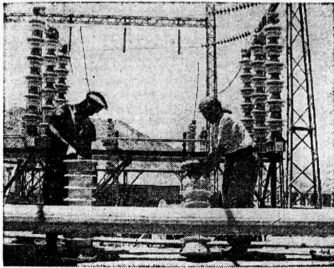
A mingecsaurei vízierőmű építkezése. A mingecsaurei vízierőmű építkezésén megkezdődött a turbinák szerelése. A szerelőmunkásokkal együtt a villanszerelők is mintaszerűen teljesítik vállalásukat. A képen: E. Mamulin (baloldalt) és T. Kuszlova transzformátor-szerelők. (Fotó: E. Sevcov.)
