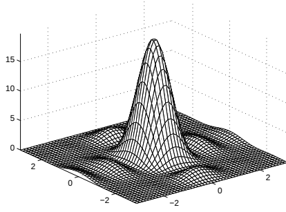
(a) The trigonometric Fejér kernel
