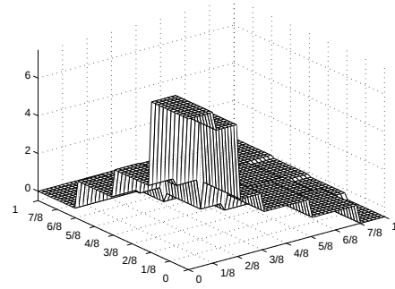
(b) The Walsh-Fejér kernel
