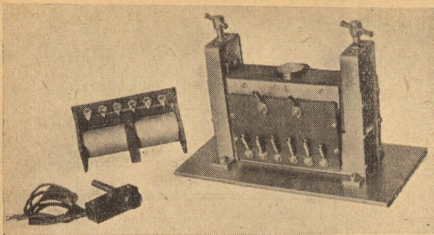
5. ábra. A nagy íga fényképe. Az íga felső részén az iránytű látható. Középen egy hozzátartozó tekercs van, melynek középső válaszfalában látható a furat a baloldali, csőbeszerelt iránytű részére.
