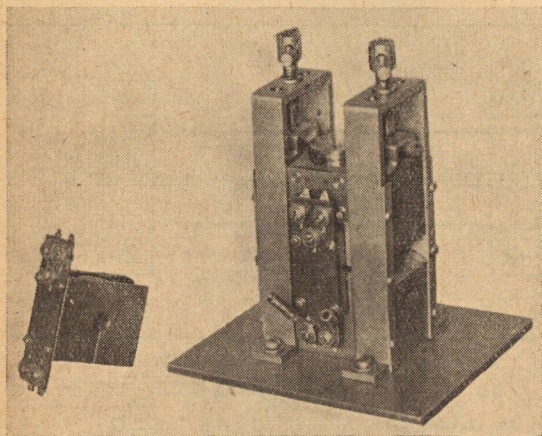
6. ábra. A kis íga fényképe. Jobboldalt az íga, baloldalt egy hozzátartozó tekercs van.
