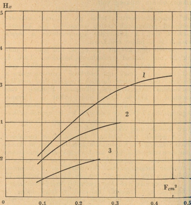
7. ábra. Bemért igakorrekciók a próbakeresztmetszet és az anyag függvényében a nagy ígára. 1 = svédvas; 2 = Si-vas; 3 = permalloy.
