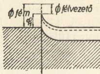
EGYENSÚLYI ÁLLAPOT A FÉM ÉS FÉLVEZETŐ ÉRINTKEZÉSE UTÁN.
