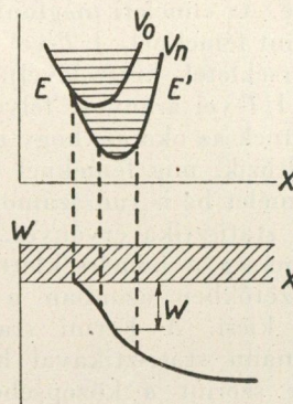
V_0 energia szabad elektronnál. V_n energia megfoglott elektronnál. W az elektron energia változása.
