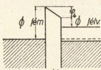
P-TÍPUSÚ FÉLVEZETŐ \varphi < 0 .
