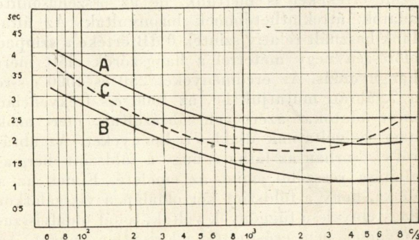
6. ábra. Az utószögési idő frekvenciagörbéi az átépítés előtt. Az A görbe az üres teremben végzett mérések eredménye, a B görbe a telt teremre átszámított érték, a C görbe az ideális utószögési időértékeket szemlélteti.
