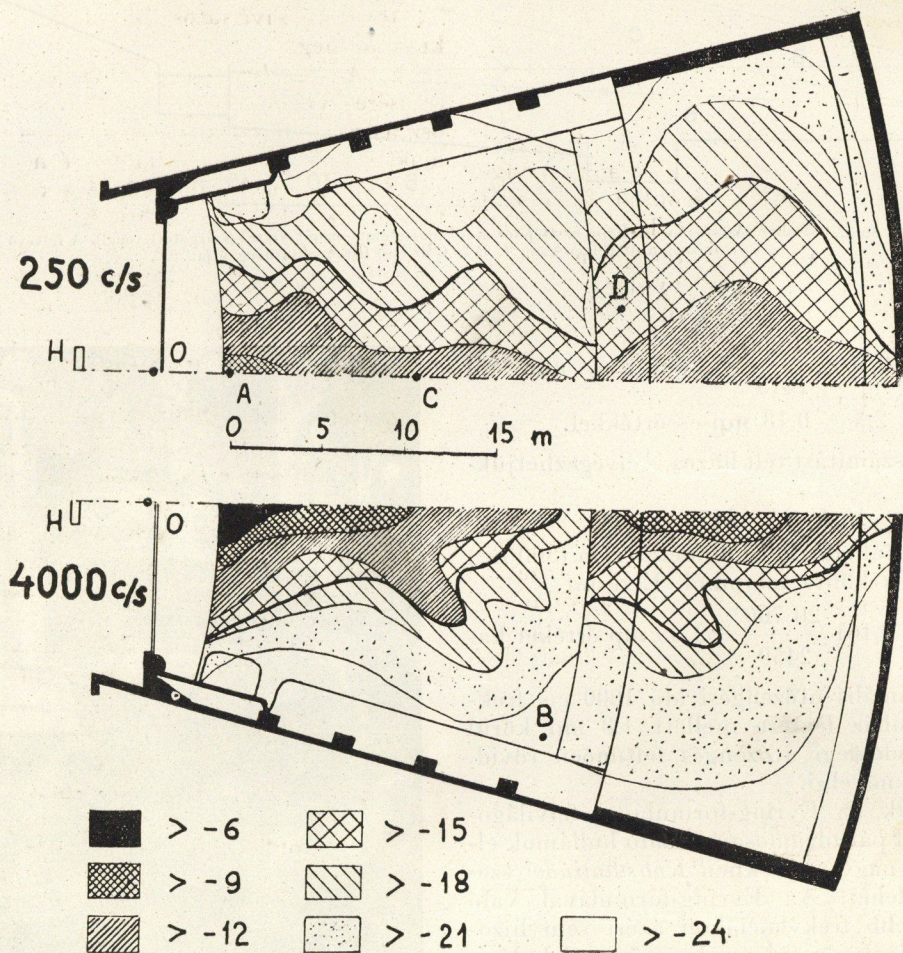
7/a ábra (felső kép) A hangnyomás eloszlása átépítés előtt 250 c/s frekvencián. A hangszórók H helyen állnak, a 0—dB szint O-ban mérhető. A, C és D helyek az utószögési idő mérőhelyei.
