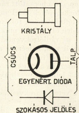
4. ábra. Kristályegyenirányító szerelvény polaritása
