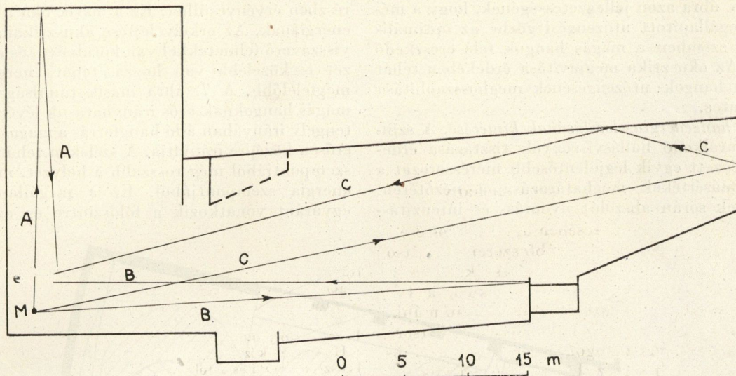
4. ábra. A színház vázlatos metszetraja az átépítés utáni proszcénium-mennyezettel (szaggatott vonal). A felvevő mikrofon M helyen van, A, B és C az első három visszhang útja.
