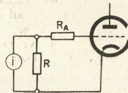
6. ábra. A kristálydetektoros vevő modulálófrekvenciánál működő áramköre
