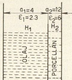
15. ábra Két sorbakapcsolt különmű szigetelő- réteg térintenzitása homogen mezőben
