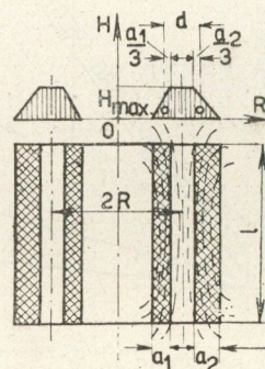
19. ábra Koncentrikus tekercselésű transzformátor szórt mezeje
