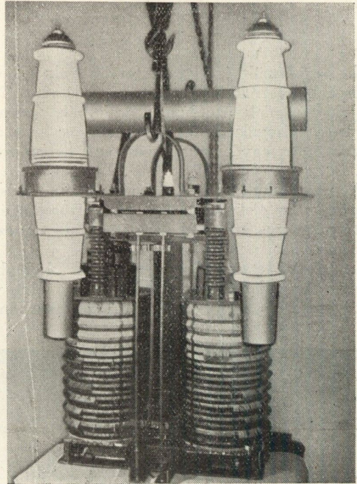
5. ábra 200 kV-os transzformátor. (Szerzőkonstrukciója)
