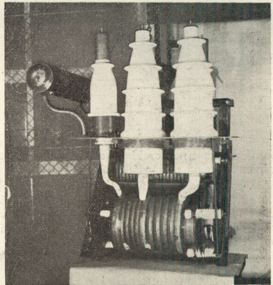
5/a ábra 100 kV-os többkivezetéses transzformátor. A Transzformátor és Mérőműszer Szövetkezet gyártmánya
