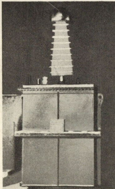
4. ábra 250 kV-os Ganz próbatranszformátor
