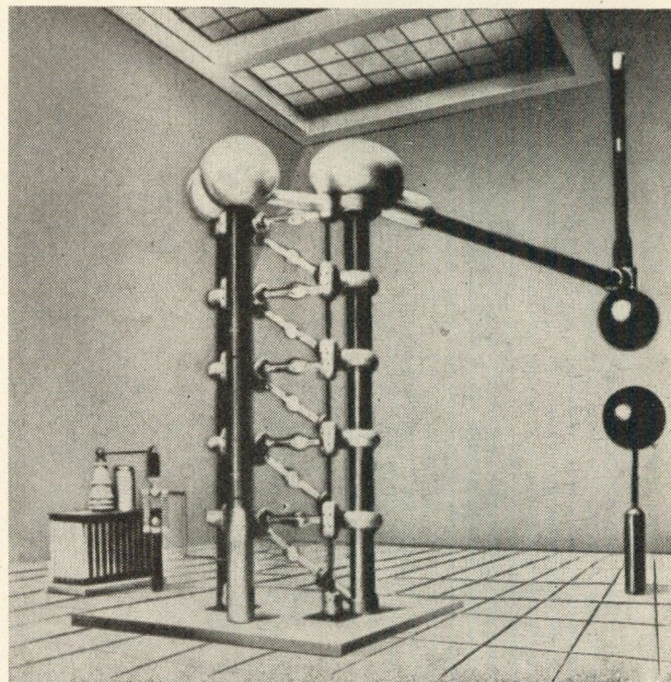
10. ábra 1000 kV-os egyenáramú kaskádgenerátor előlnézeti en (Szerző konstrukciója)
