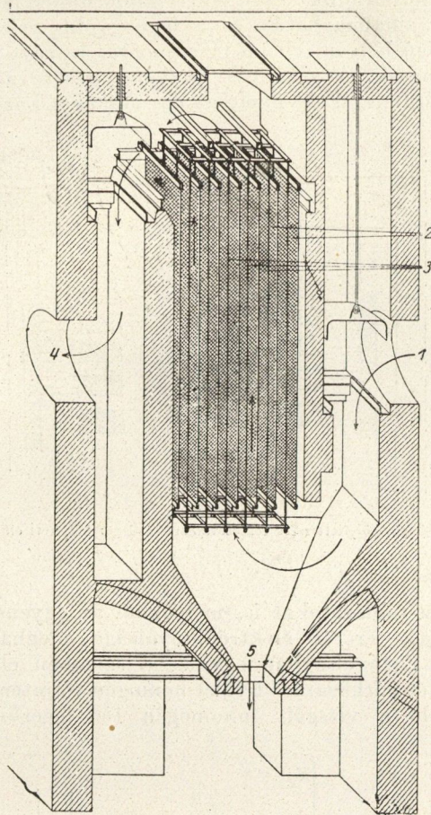
11. ábra Villamos szűrőszűrő elv
