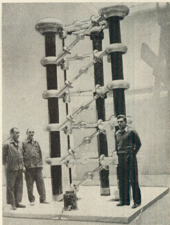
10/a ábra 1000 kV-os egyenáramú kaskádgenerátor
