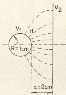
14/a ábra Gömb-síkfelület erőtere
