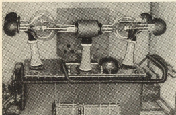
9. ábra 115 kV-os röntgentranszformátor ráépített négy szelepesövel Grütz-kapcsolásban 500 mA pillanatnyi terhelésre
