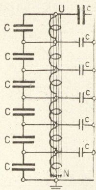
18. ábra. Egyik végén földelt tekercselés kapacitás- eloszlása
