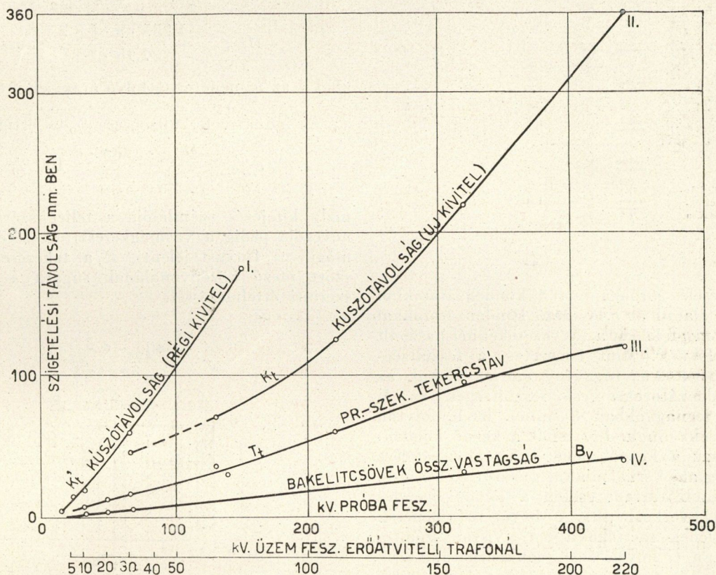
17. ábra, Szigetelési távolságok a próbafeszültség függvényében. (Az abszcissa alsó számsora az üzemi feszültséget jelenti az erőátviteli transzformátorokra vonatkozó szabvány szerint.)
