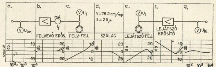
17. ábra Teljes magnetofon-berendezés frekvencia-karakterisztikái
