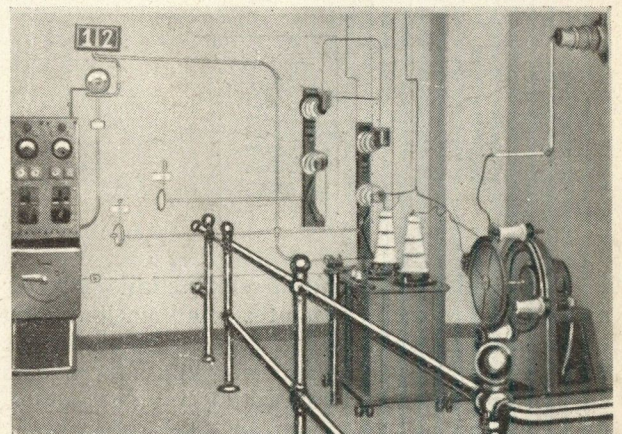
11/a ábra Villamos szűrő táplálására épült forgó egyenirányító: a áramforrás
