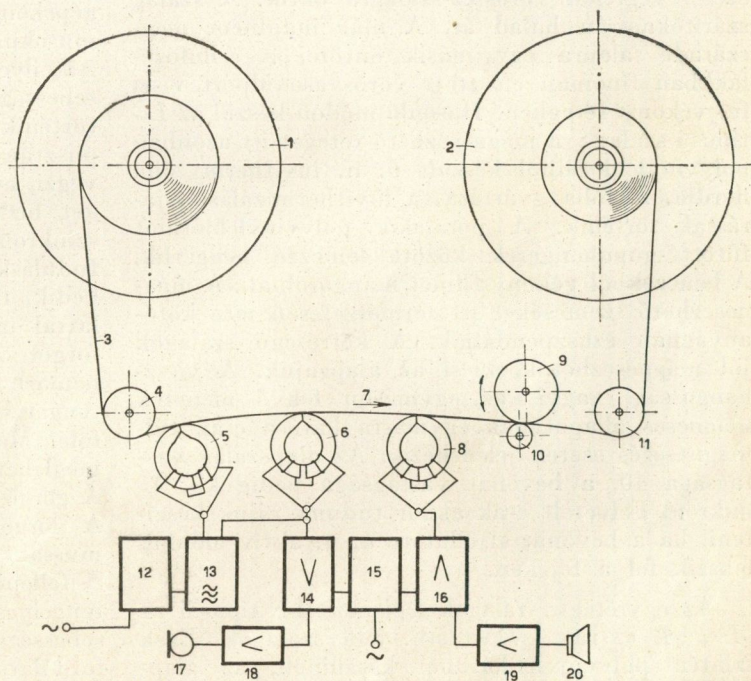
1. ábra. A mágneses hangrögzítő berendezés elvi felépítése
