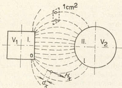
12. ábra Erőtér egyenlőtlen erővonalasűrűséggel
