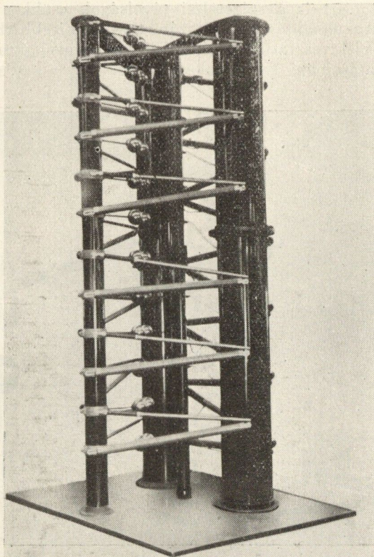
6. ábra 1500 kV-os lökésgeneresztő. Häfeld-gyártmány
