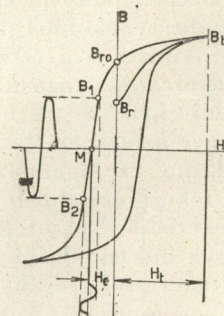
5. ábra. Egyenáramú törlés és előmágnesezés
