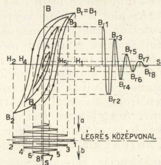
7. ábra. A nagyfrekvenciás törlés folyamata
