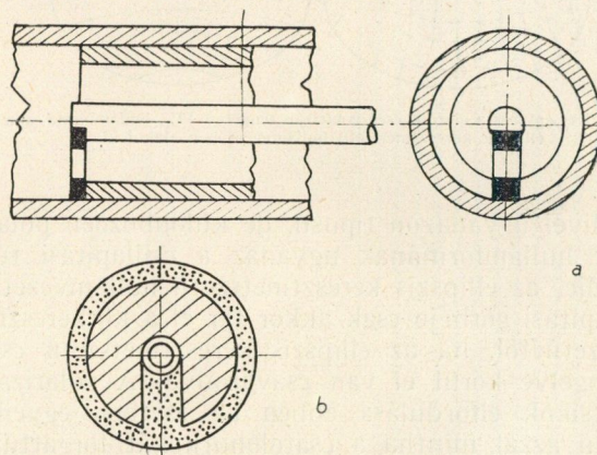
7/a ábra. TE 11 hullámformát használó határfrekvencia alatti csillapító illesztése ellenállásból készült csatoló hurokkal
