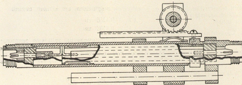
8. ábra. TE_{11} hullámformájú határfrekvencia alatti csillapító
