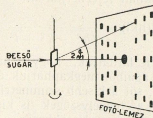
5. ábra. Röntgenfelvétel elrendezése síklemez esetén
