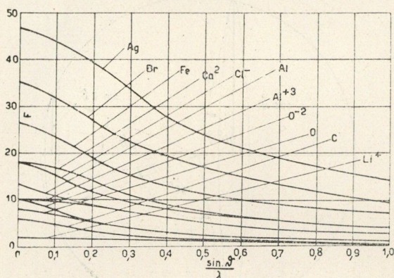
7. ábra. Néhány atom és ion atomtényezője
