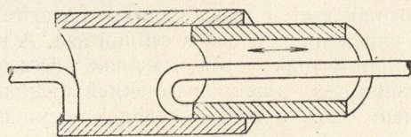
a) TE hullámformával működő határfrekvencia alatti csillapító
