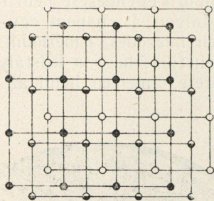
3. ábra. Síkrácsok egymáshatolt rendszere
