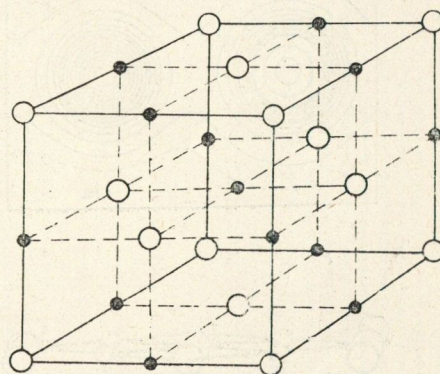
9/d ábra. Komplex lapcentrált rács elemi cellája (NaCl)
