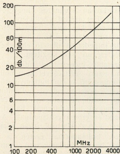
6. ábra. Kábelek csillapításának változása a frekvencia függvényében
