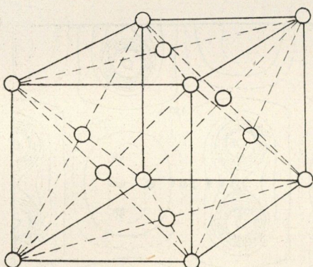
9/b ábra. Lapcentrált rács elemi cellája (Réz)
