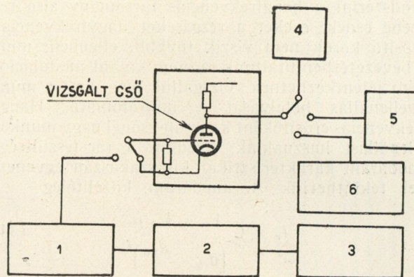
4. ábra. Méri elrendezés.
