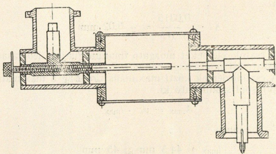
9. ábra. TM_{01} hullámformájú határfrekvencia alatti csillapító
