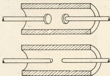
b) TM hullámformával működő határfrekvencia alatti csillapító
