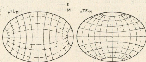
4. ábra. Két egymásra merőlegesen polarizált tengelyű TE_{11} hullámforma, amely ellipszis keresztmetszetű hullámvezetőben alakul ki.
