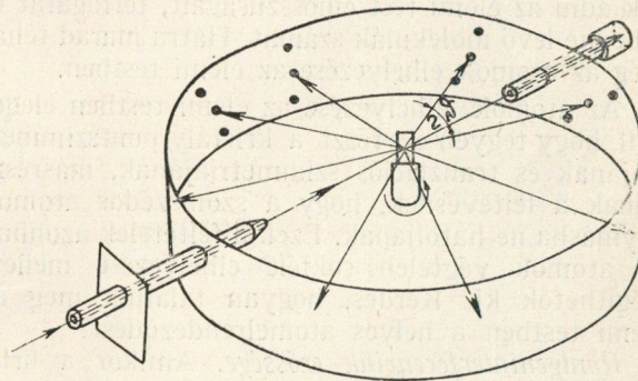
6. ábra. Debye-Scherrer-féle röntgenkamera vázlatos rajza
