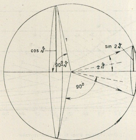
8. ábra. A Debye–Scherrer-féle porfölvételek interferenciáinak erősségéhez tartozó geometriai tényező levezetése
