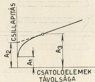
3. ábra. Határfrekvencia alatti csillapító csillapítása a csatoló elemek távolságának a függvényében
