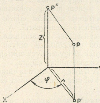
1. ábra. Henger koordináta rendszer
