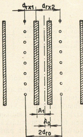
2. ábra. Katódmozgás esete.
