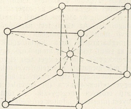
9/a ábra. Tércentrált rács elemi cellája (Wolfram)
