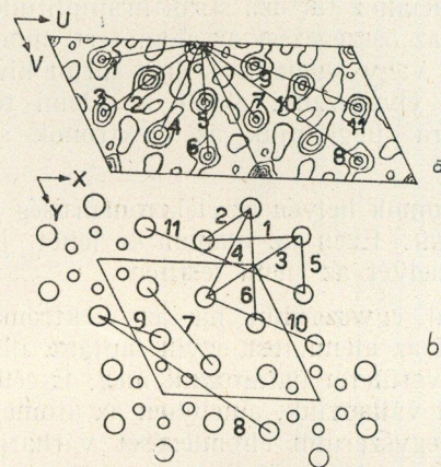
12. ábra. a) \text{C}_6\text{Cl}_6 kétdimenziós Patterson elemzésének ábrázolása az (u,v) koordináta-rendszerben. A számozott egyenesek a fontosabb maximumok rádiuszvektorait jelölik ki
