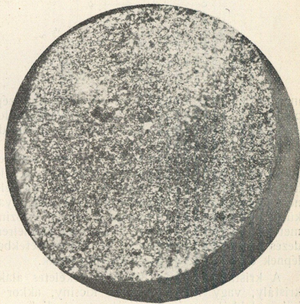
2. ábra. W drót törési felülete 15-szörös nagyításban
