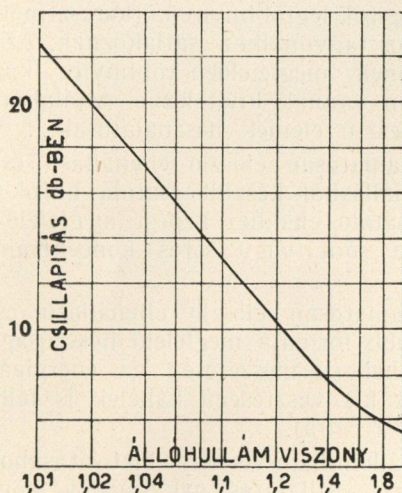
5. ábra. Adott állóhullám-viszony biztosításához szükséges illesztőelem csillapítása
