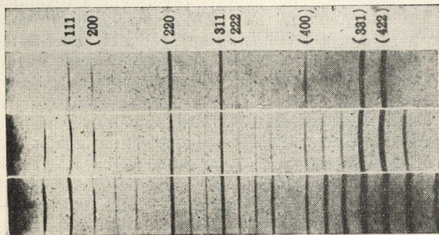
13. ábra. AuCu 3 röntgenfölvétel; a felső (a) rendezetlen, a középső (b) részben és az alsó (c) egészben rendezett rács esetén
