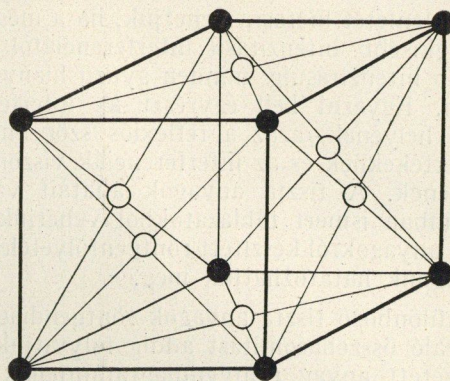
12/b. ábra. \text{AuCu}_3 rendezett rácsa
