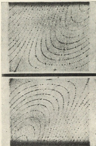
3. ábra. Egyenlőszögű Weissenberg-féle röntgenfölvétel \text{AsS} -ről: a c tengely körüli forgatás első rétegvonal
