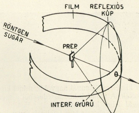
5. ábra. Debye—Scherrer-féle porfölvétel egy reflexiós kúpja
