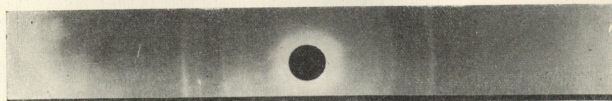
10/e ábra \gamma\text{-Al}_2\text{O}_3 + 0,2\% \text{MoO}_3
