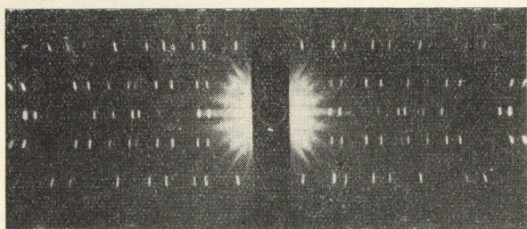
1. ábra. Bragg-féle forgókristályfőlvételek hengerkamrában, kvarckristályról (001) tengely körüli forgatással
