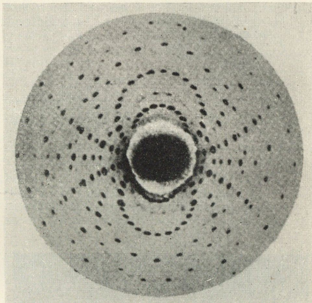
4. ábra. Laue-fölvétel cerussitról
