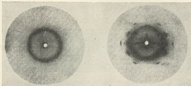
8. ábra. Kaucsuk röntgendiagrammja.
