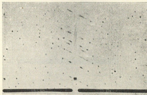
2. ábra. A Weissenberg és forgókristályfőlvételek közti összefüggés. A rétegvonal széthúzása a nyíl irányában történt
