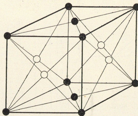
14. ábra. Rendezett AuCu rács
