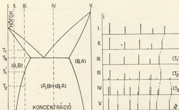
15. ábra. Részlegesen oldódó kristályos anyag fázisdiagramja és sematikus röntgendiagramja különböző összetételnél és hőkezelésnél.
