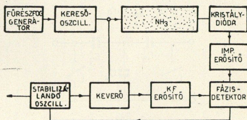
26. ábra. Kereső-rendszerű stabilizálás gáz abszorpciójával
