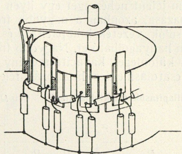
14. ábra. Lánccolt műcsillapítás egyik dekádjának kapcsolója
