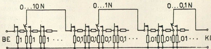
13. ábra. Lánccapcsolású műcsillapítás
