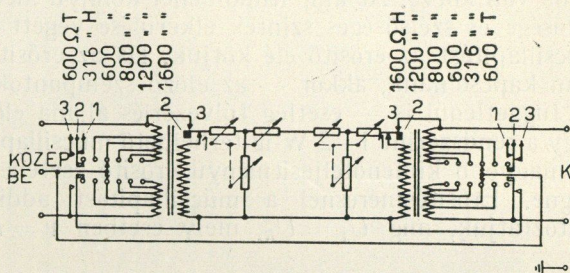
9. ábra. Transzformátor illesztésű műcsillapítás
