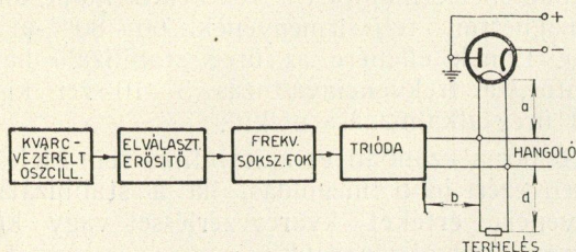
14. ábra. Magnetron kristályvezérlése
