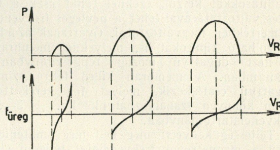
1. ábra. Reflex-klisztron frekvenciájának és teljesítményének változása a reflektorfeszültség függvényében
