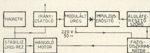
16. ábra. Mikrohullámú diszkriminátor modulált üregrezonátorral
