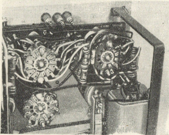
15. ábra. Bifiláris tekercsű műcsillapítás
