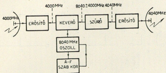
24. ábra. Frekvenciakülönbség stabilizálása A—F rendszerrel
