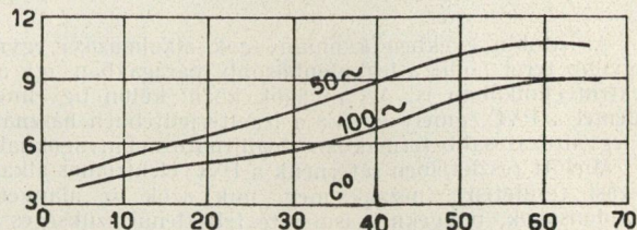
5. ábra. A PVC dielektromos állandójának a változása a hőmérséklet függvényében, különböző frekvenciákon.
