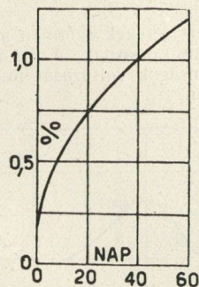
2. ábra. Trikrezilfoszfáttal lágyított, 25 °C hőmérsékletű vízben tartott PVC vízfelvele az idő függvényében.
