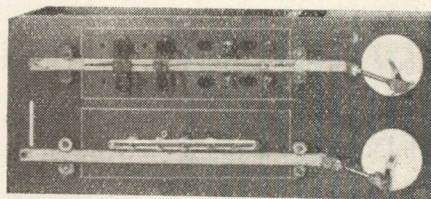
11. ábra. Fárasztókészülék billenős és forgócsapos kapcsolókhoz, valamint hullámváltókhoz
