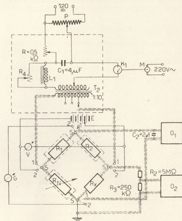
2. ábra. Impulzsmódszerrel működő árnyékolt Wheatstone-híd ellenállások feszültségi tényezőjének mérése.
