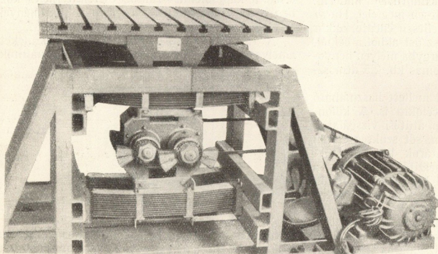
14. ábra. Nagy rázógép
