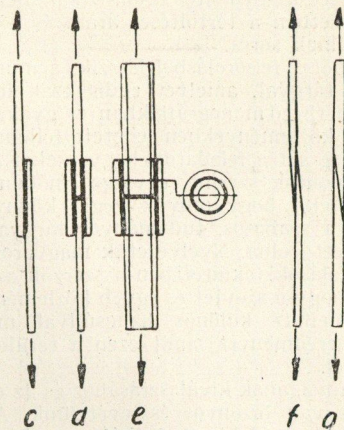
3. ábra. Ragasztástechnológiailag elfogadható kötési formák. c) átlapolt, egynyírási kötés, d) átlapolt, kétnyírási kötés, e) csőkötés, f), g) lelétezett kötések
