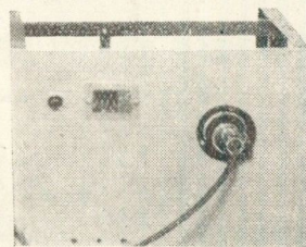
12. ábra. Fárasztókészülék finombeállítókhoz
