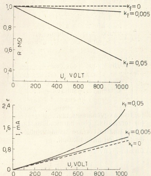
1. ábra. Feszültségfüggetlen feszültségi tényező hatása. Az ellenállás és az áram változása a feszültség függvényében, 1 MΩ ellenállás esetén
