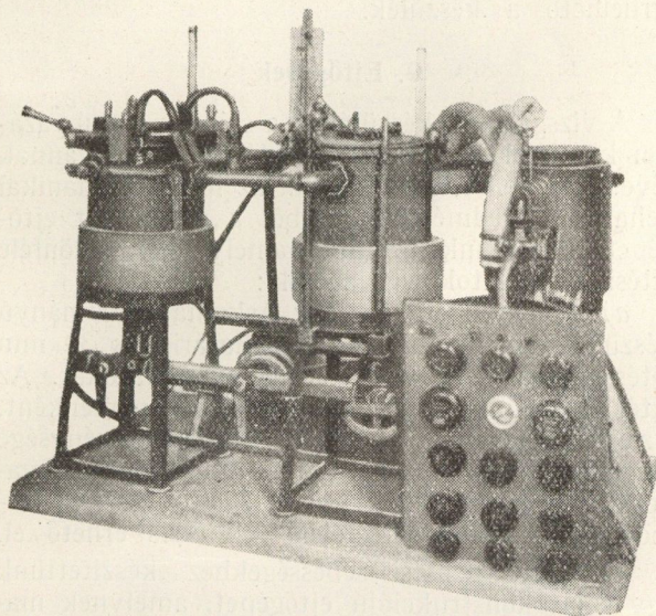
9. ábra. Vacuumberendezés
