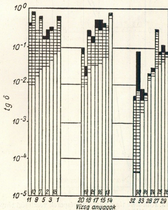
7. ábra. Dielektromos veszteségi tényező változása 1 MHz-en, 100% relatív nedvességtartalmú térben, 25 °C-on
