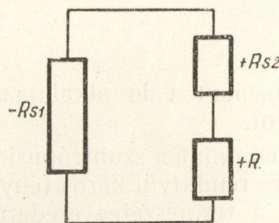
3. ábra. Rezonáns vevőantenna helyettesítő kapcsolása
