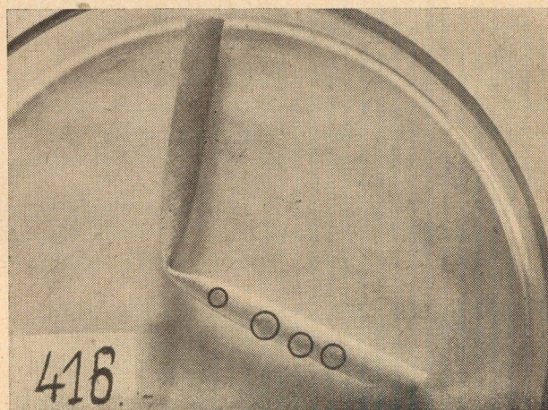
19. ábra. Varnish szigetelőcső; foltokban penészes.
