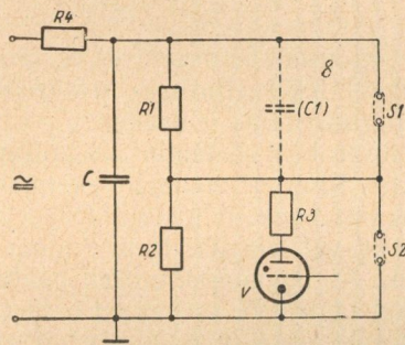
1. ábra. Villanó megvilágító rendszer két szikra vagy villanócső egyidejű működtetéséhez. C = kondenzátor, R1—R4 = ohmos ellenállások, S1—S2 = villanócsővek vagy szikraközök, V = thyatroncső
