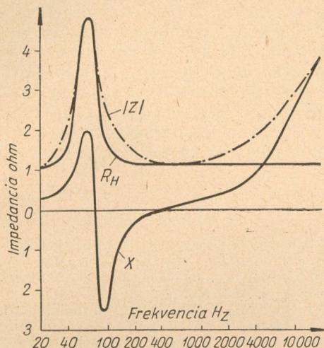
7. ábra. Dinamikus hangszóró impedanciája a frekvencia függvényében. R = a lengőcséve ohmos ellenállása.
