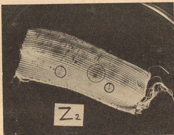
16. ábra. Kezeletlen szalagkábel. Erősen penészes.
