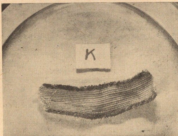
17. ábra. 1% fungicid anyaggal kezelt szalagkábel. Széleken penészesedés.
