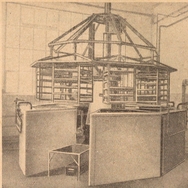
3. ábra. Tárgyelőkészítő (zsirtalanító és pácoló) körautomata
