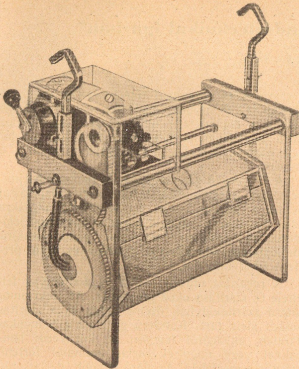
5. ábra. Állófürdőbe meríthető kézi dob
