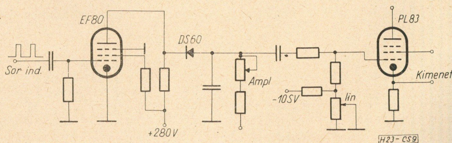
9. ábra. Fűrészelet előállító kapcsolás
