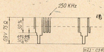
6. ábra. 250 kHz-es négyszög
