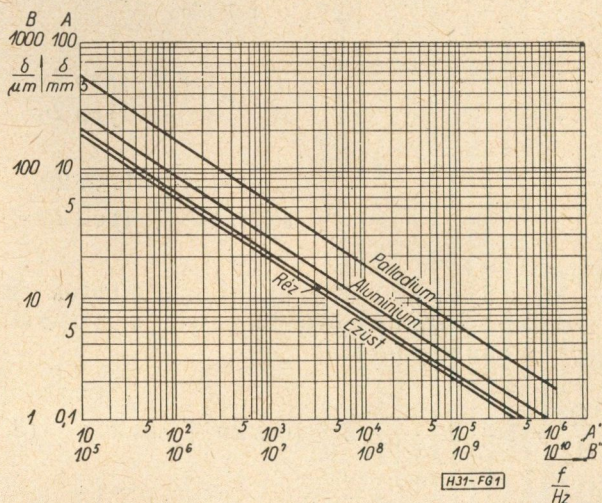
1. ábra. A behatolási mélység függése a frekvenciától „A” skála: 10 \text{ Hz} < f < 10^{10} \text{ Hz} ; 0,1 \text{ mm} < \delta < 100 \text{ mm} „B” skála: 10^5 \text{ Hz} < f < 10^{10} \text{ Hz} ; 1 \mu\text{m} < \delta < 1000 \mu\text{m}
