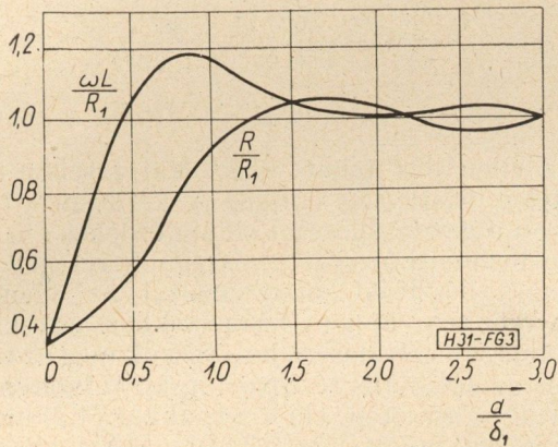
3. ábra. Rétegezett féltér ellenállása és reaktanciája : \alpha = 0,34 [3]
