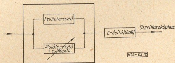
12. ábra. Zajmérő elvi vázlata
