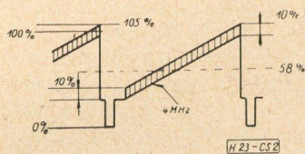
2. ábra. Háromszögjel mérő színusszal
