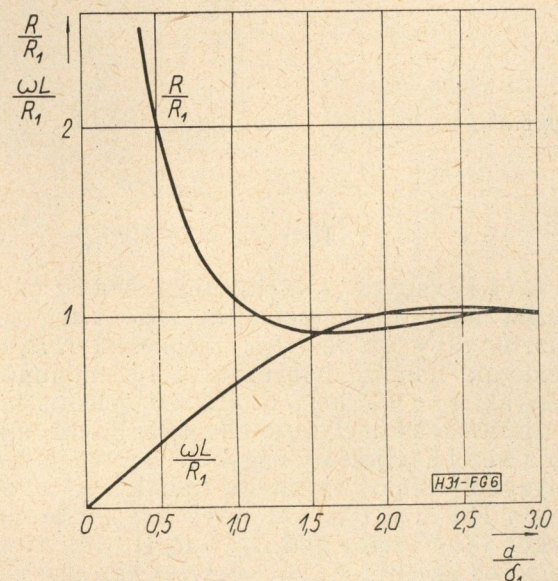
6. ábra. Lemez ellenállása és reaktanciája ( \alpha = \infty )
