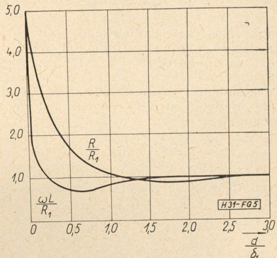
5. ábra. Rétegezett féltér ellenállása és reaktanciája : \alpha = 5 [3]
