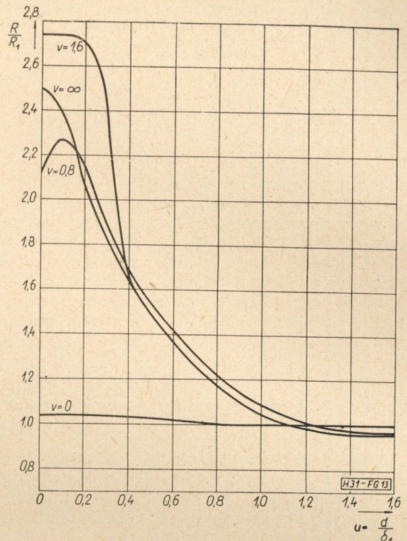
13. ábra. Az ellenállás változása a felső réteg vastagságának függvényében. A második réteg vastagsága az egyes görbékre állandó
