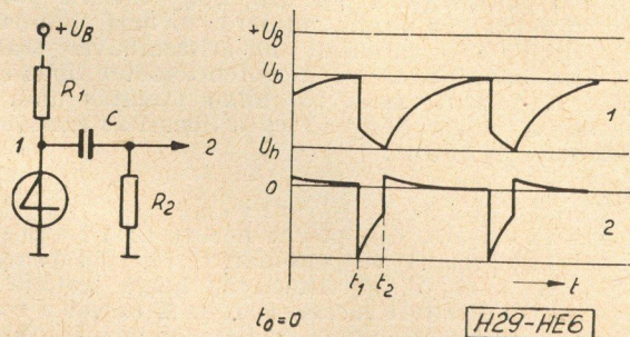
3. ábra. Fűrészfeszítés generátor
