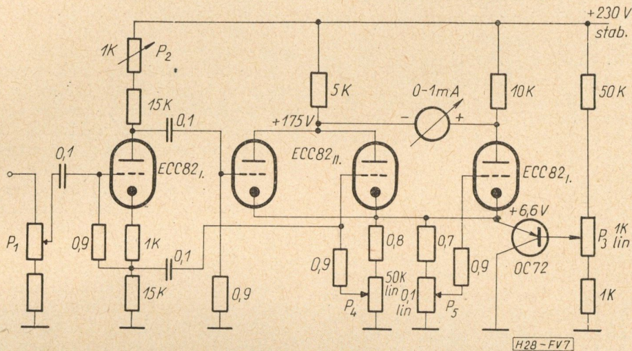
7. ábra A megépített műszer teljes kapcsolása
