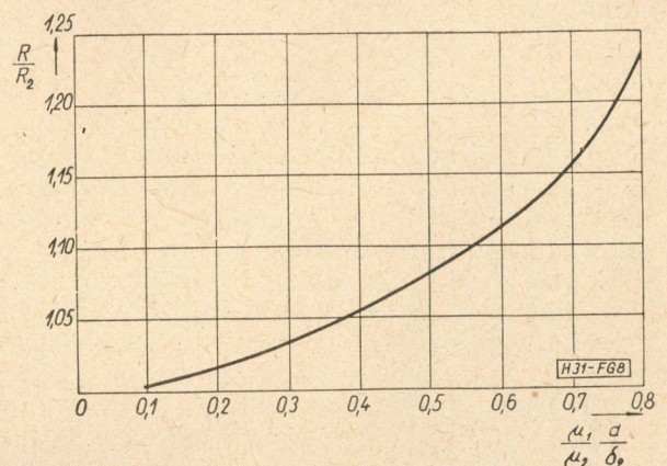
8. ábra. Maximális ellenállás a rétegvastagság függvényében
