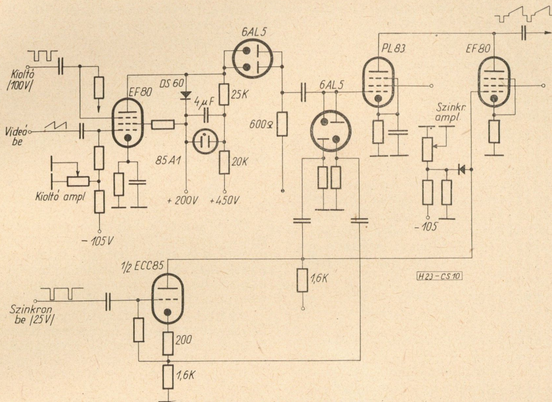
10. ábra. Keverő egység
