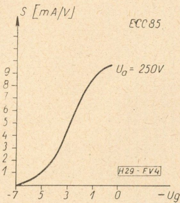
4. ábra. S_1 (U_g) karakterisztikák ECC85
