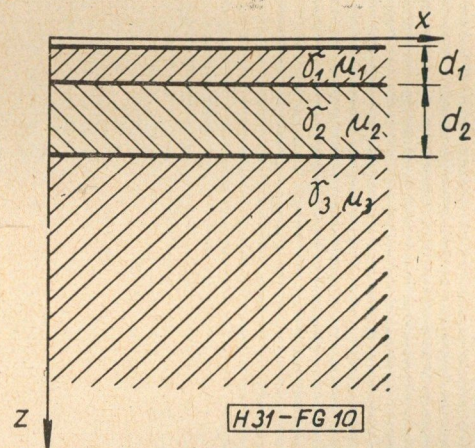
10. ábra. Kettős rétegezésű feltér elrendezése
