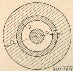
12. ábra. Rétegezett üreges hengeres vezető belső visszavezetéssel
