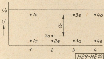
7. ábra. Vezérelt fűrészgénerátor
