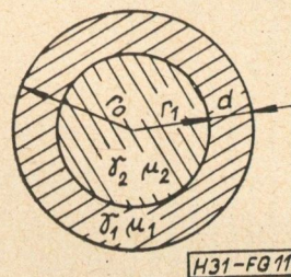
11. ábra. Rétegezett tömör hengeres vezető
