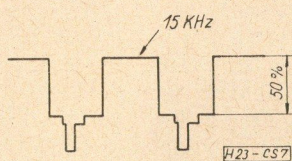
7. ábra. 15 kHz-es négyszög
