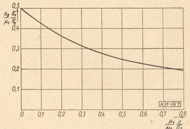
7. ábra. A maximális ellenálláshoz tartozó \gamma_1 vezetőképeség a rétegvastagság függvényében
