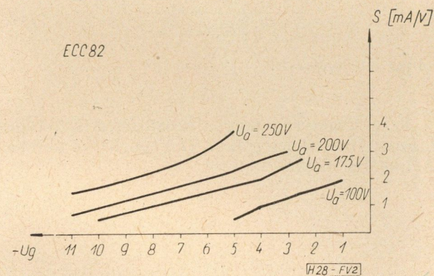
2. ábra. S_1 (U_g) karakterisztikák ECC82
