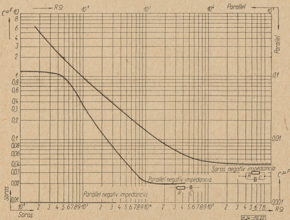
27. ábra. Komplex vonalutánszat alkalmazása esetében a stabilitást biztosító vonalutánszat-kombinációk
