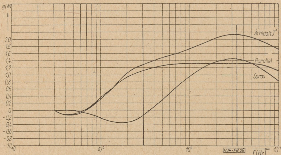
26. ábra. Az erősítés (g) 600 Ohmos rendszerben a frekvencia függvényében. A vonalutánszat a soros negatív impedanciájú erősítő esetében 900 Ohm, a párhuzamos típusnál 400 Ohm
