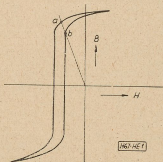
1. ábra. Báriumferrit mágnes
