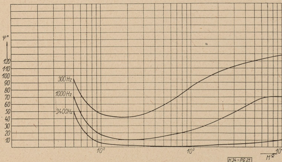
21. ábra. A valós vonalutánszimpedancia transzformálásának fázisszöge a vonalutánszimpedancia értékek függvényében, soros jellegű negatív impedanciájú erősítő esetében
