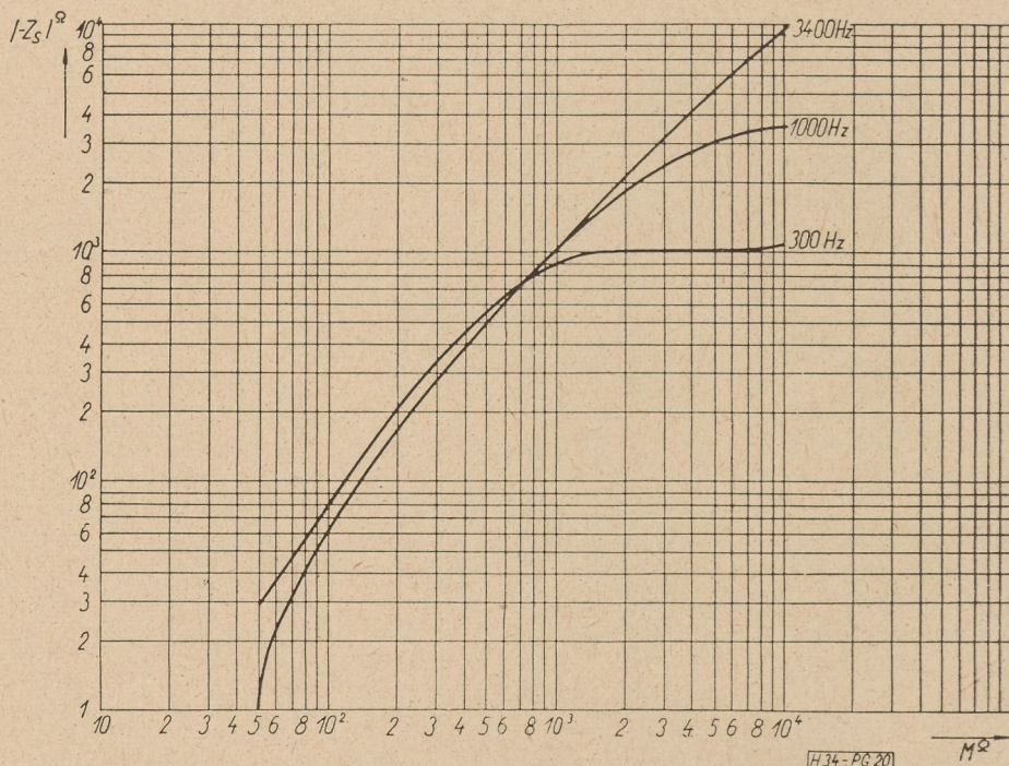
20. ábra. A valós vonalutánszimpedancia transzformálása a vonalutánszimpedancia értékek függvényében soros jellegű negatív impedanciájú erősítő esetében
