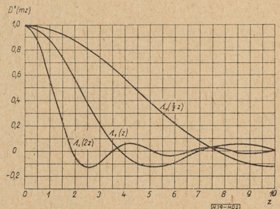
2. ábra. A D^*(z) = \Lambda_1(z) ; D^*(m_e z) = \Lambda_1(z) ; D^*(m_g z) = \Lambda_1\left(\frac{1}{2}z\right) , természetes és módosított irányítási tényezők
