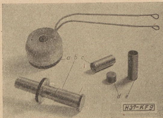
9. ábra. Magnéziumból folytatott fiolák a) szerszám alsórész; b) tűske; c), e) kész munkadarabok; d) előgyártmány
