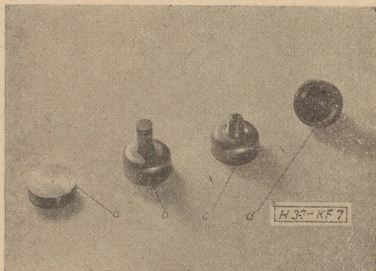
7. ábra. Sárgarézből hidegfolytatott regulátor csésze a) előgyártmány; b) hidegfolytatott munkadarab; c) kész munkadarabok
