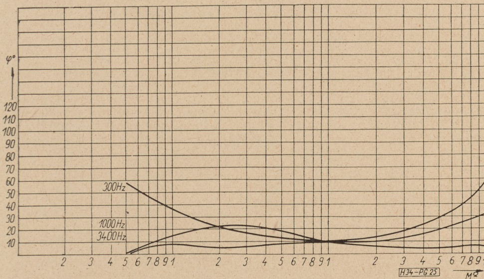
25. ábra. A valós vonalutánnal transzformálásának fázisszöge a vonalutánnal értékeinek függvényében, párhuzamos jellegű negatív impedanciájú erősítő esetében
