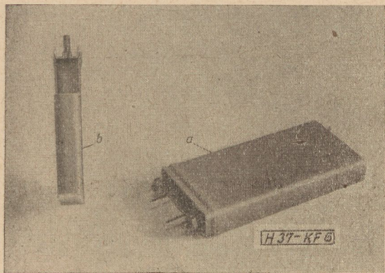
6. ábra. Kondenzátor hidegen folytatott dobozban, hideghegesztéssel lezárva a) kész kondenzátor; b) metszet.
