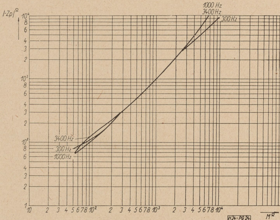
24. ábra. A valós vonalutánnal transzformálása a vonalutánnal értékeinek függvényében, párhuzamos jellegű negatív impedanciájú erősítő esetében
