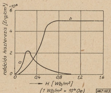
3. ábra. Pólusborítás
