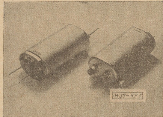
1. ábra. Telefon egységdoboz kondenzátorok hidegen folyatott dobozban, hideghegesztéssel lezárva
