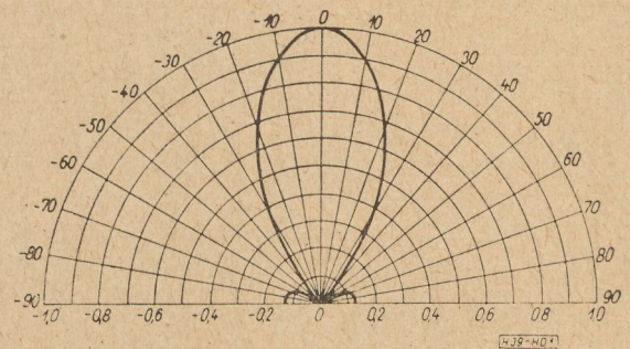
1. ábra. A sugárzó irányjelleggörbéje kr = 5 esetében. Az irányítási tényező D^*(z) = \Lambda_1(z)
