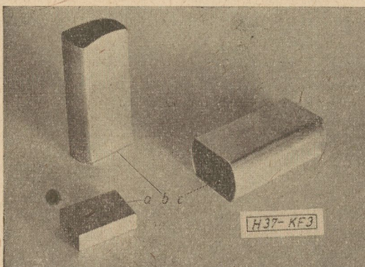
3. ábra. Kondenzátor doboz a) előgyártmány; b) hidegfolyatott doboz; c) méretre vágott doboz
