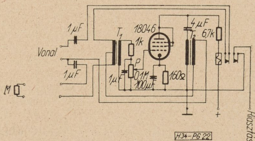
22. ábra. Párhuzamos jellegű negatív impedanciájú erősítő
