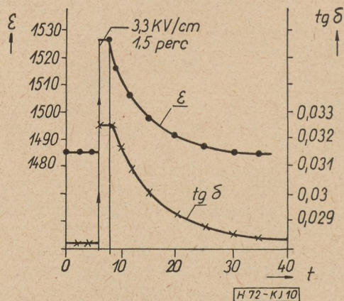
10. ábra. \text{BaTiO}_3 dielektromos állandójának ( \epsilon ) veszteségtényezőjének ( \text{tg } \delta ) időbeli esése, 3,3\text{ kV/cm} térerősséggel rövid ideig tartó (1,5 perc) terhelés után; t = perc
