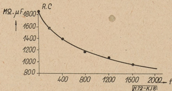
8. ábra. Polietiléntereftálsavészter fólia szigetelési ellenállásának változása az üzemeltetési idő ( t , óra) függvényében. T = 70\text{ }^{\circ}\text{C} ; U_{\text{név}} = 100\text{ V} ; fólia vastagság = 3\mu
