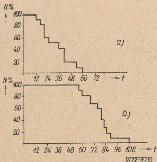
6. ábra. Klórozott naftalinnal impregnált papírkondenzátorok forszírozott élettartam vizsgálata; a) stabilizálatlan sorozat; b) 1,1 % antrachinonnal stabilizált sorozat; U_{n\acute{e}vl} = 500 \text{ V} ; U_{vizsg} = 900 \text{ V} ; T = 90 \text{ }^\circ\text{C} ; t = \text{óra} ; N = a \text{ } t időben megmaradt darabok százaléka
