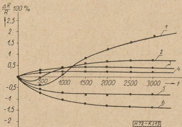
15. ábra. Különböző kristályszenréteg ellenállások változása az üzemeltetési idő függvényében ( 0,5\text{ watt} , 100\text{ Kohm} ); t = üzemeltetési idő órákban; 1 — a krakkolás vákuuma 0,5\text{--}0,8\text{ Hgmm} ; 2 — 2 osztályú ellenállás; 3 és 4 — 0,5 oszt. ellenállás; krakkolási sebesség 0,5\text{ cm}^3 heptán/óra; 5 és 6 — 2. osztályú ellenállások
