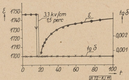
11. ábra. (Ba, Sr) \text{TiO}_3 dielektromos állandójának ( \epsilon ) és veszteségi tényezőjének ( \text{tg } \delta ) időbeli lefolyása a Curie hőmérséklet felett, 1,5 percig 3,3 KV/cm télerősséggel való terhelés után; t = perc
