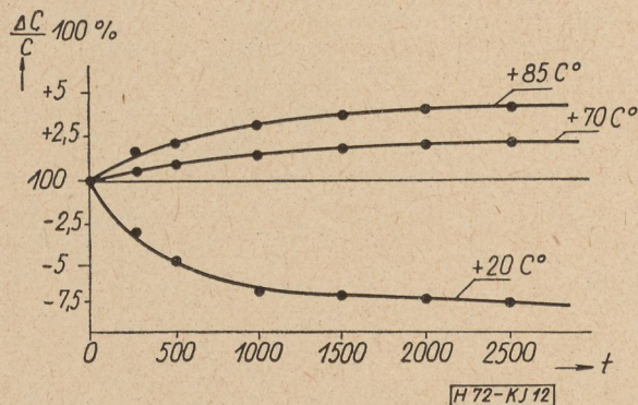
12. ábra. Elektrolitos kondenzátorok kapacitásának változása az üzemeltetési idő függvényében különböző környezeti hőmérsékletek esetében; C = 2 \times 50 \mu\text{F} ; U = 350/385 \text{ V} ; t = üzemeltetési idő órákban
