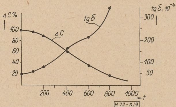
9. ábra. Fémezett papirkondenzátorok kapacitásának és veszteségi tényezőjének változása az üzemeltetési idő függvényében, 90\text{ }^{\circ}\text{C} környezeti hőmérséklet esetén; t = üzemeltetési idő, órákban
