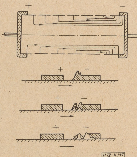
17. ábra. A kristályszenréteg elektrokémiai bomlásának mechanizmusa
