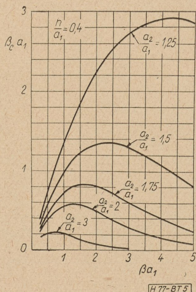
5. ábra. Az energiahullámszórás fázistényezője az egyedülálló helix menti hullámterjedés fázistényezőjének függvényében különböző \frac{a_2}{a_1} értékekre, ha \frac{h}{a_1} = 0,4
