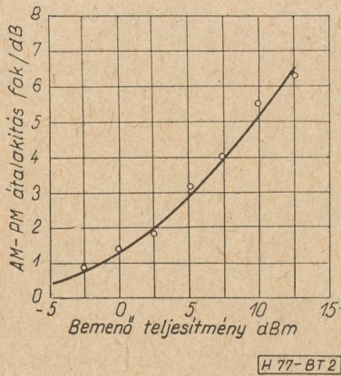
2. ábra. AM-PM átalakítás a bemenő teljesítmény függvényében
