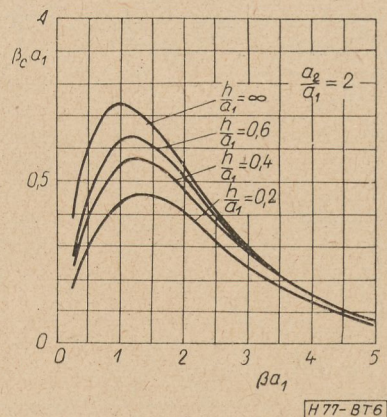
6. ábra. Az energiahullámszórás fázistényezője az egyedülálló helix menti hullámterjedés fázistényezőjének függvényében különböző \frac{h}{a_1} értékekre, ha \frac{a_2}{a_1} = 2
