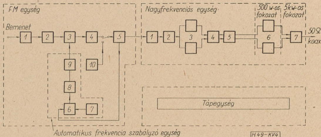
4. ábra. A hangadó tömbvázlata
