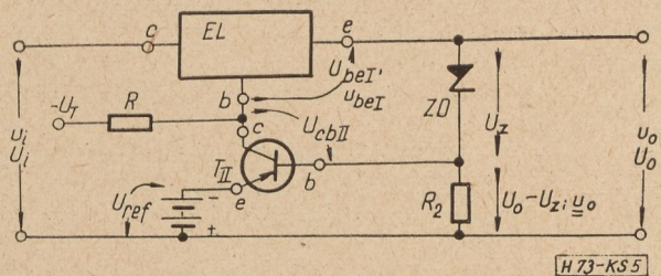
5. ábra. Zenerdióda alkalmazása a kimeneti osztóban
