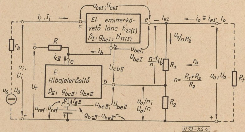
4. ábra. Egyenáramú hibajelerősítő beiktatása
