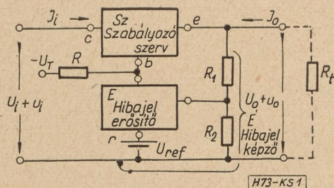
1. ábra. A stabilizátor blokkismérete
