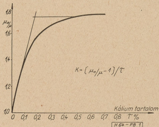
1. ábra. Kálium szennyezés hatása a kezdőpermeabilitásra [1]
