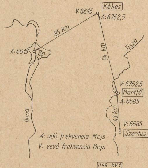
1. ábra. Moduláló összeköttetés nyomvonala és frekvencia-kiosztása
