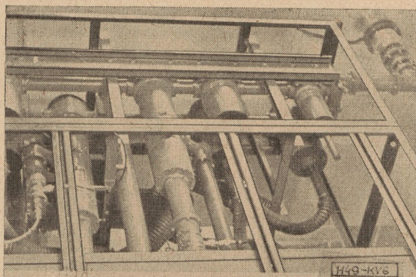
6. ábra. Diplexer és oldalsávszűrő szerkezete
