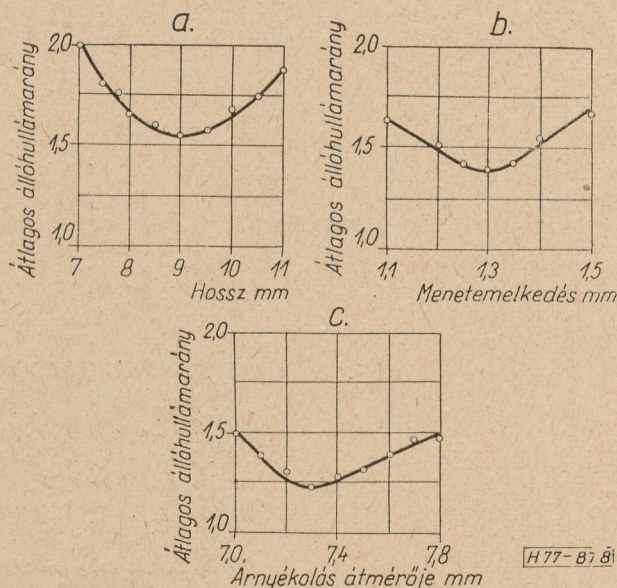
8. ábra. Átlagos állóhullámarány a helixméretek függvényében
