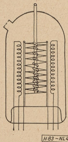
4. ábra. Alpert—Blankfield-féle titán iongetter-szivattyú
