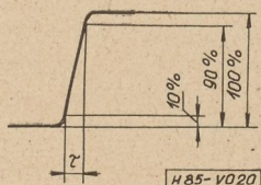
20. ábra. Felfutási idő meghatározása
