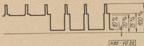
22. ábra. 50 Hz négyszögfeszültséggel modulált adó kimenőjele
