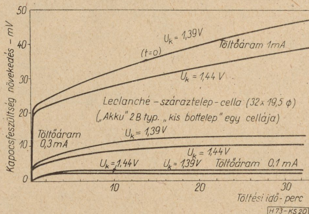
20. ábra. Száraztelep kapacitásváltozása a töltőáramtól
