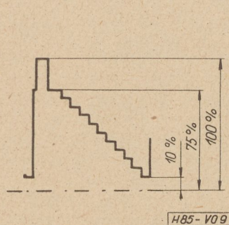
9. ábra. Gradációs skálával modulált adó kijövő jele
