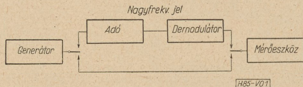
1. ábra. Általános mérési elrendezés
