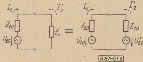
5. ábra. Négypólus szekunder oldalának lezárása helyettesítő reflexiófeszültség-forrással
