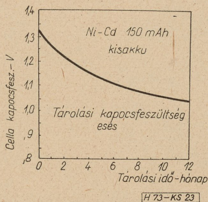
23. ábra. Ni-Cd kisakkumulátor kapcsolófeszültségesése
