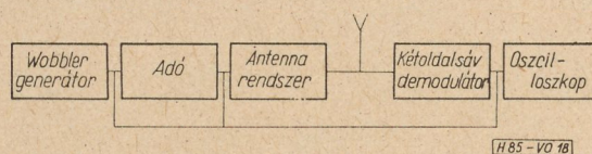
18. ábra. Nagyfrekvenciás frekvencia karakterisztika mérési összeállítása
