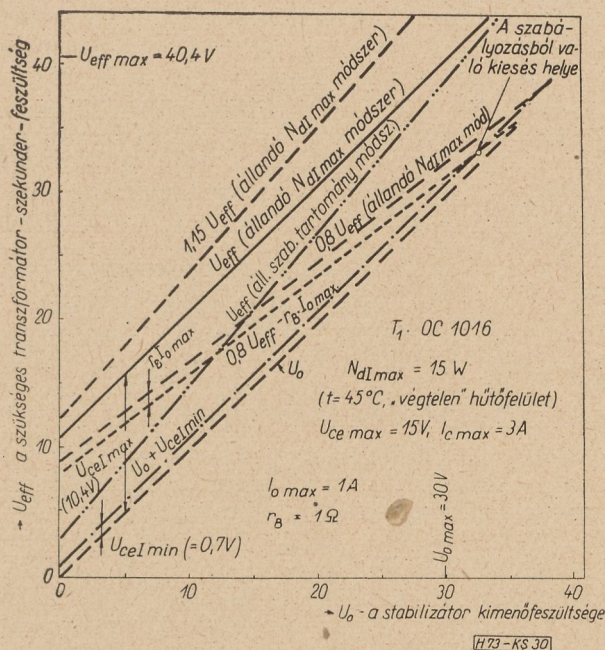
30. ábra. A szükséges transzformátorfeszültség grafikus meghatározásának módszerei
