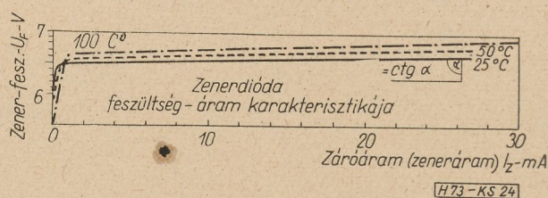
24. ábra. Zener-dióda U-I karakterisztikája
