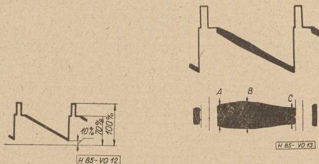
12. ábra. Linearitásméréshez használt jel az adó kimenetén
