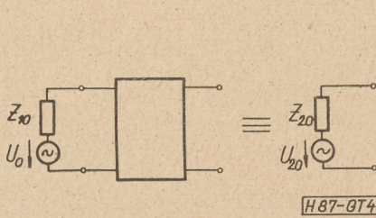
4. ábra. Négypólus szekunder oldalának feszültséghelyettesítő kapcsolása
