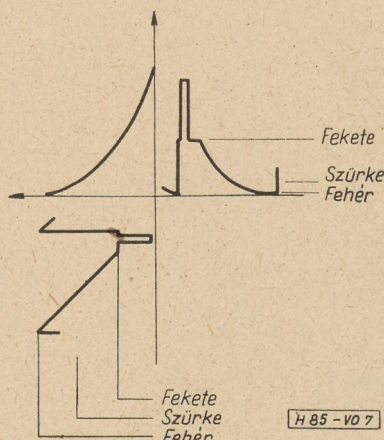
7. ábra. Torzulás keletkezése a fűrészfeszültségnél
