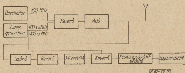
17. ábra. Kétoldalsáv demodulátor tömbvázlata
