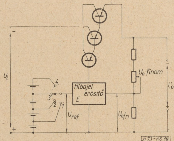
19. ábra. Változó feszültségű telep-referencia stabilizátor
