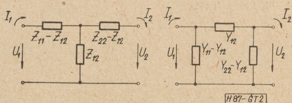
2. ábra. Négypólus helyettesítő kapcsolásai az ellenállás- és vezetéskarakterisztikák szemléltetésére
