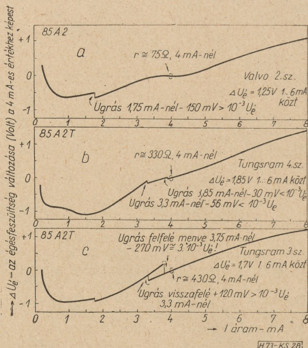
28. ábra. Parázfénystabilizátorcső „finomstruktúrája” U - I karakterisztikája
