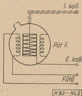
2. ábra. Bayard—Alpert-féle ionizációs manométer
