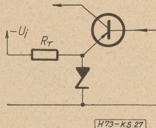
27. ábra. Zener-diódás referencia kisigényű kapcsolásokhoz
