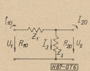
6. ábra. Illesztő L-kapcsolás
