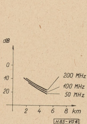
6. ábra. A különböző frekvenciák relatív csillapítása a távolság függvényében
