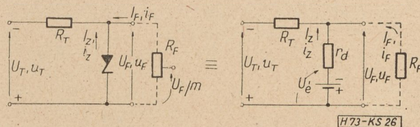
26. ábra. Zener-dióda referenciaforrás és helyettesítő áramkör
