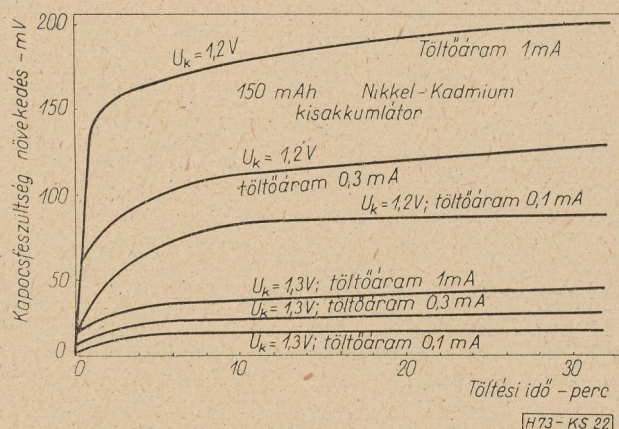
22. ábra. Ni-Cd kisakkumulátor kapcsolófeszültség függése a töltőáramtól
