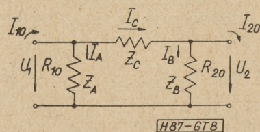
8. ábra. Illesztő \Pi -kapcsolás
