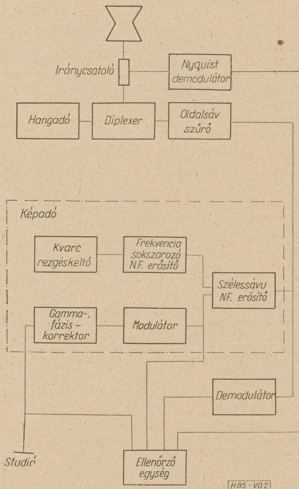
2. ábra. Adó tömbvázlata
