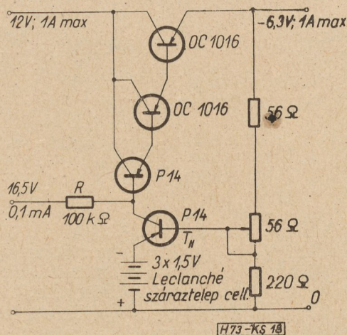
18. ábra. Fix feszültségű telep-referencia stabilizátor
