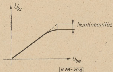
8. ábra. Pontonként felvett modulációs jelleggörbe
