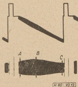
13. ábra. Linearitásméréshez használt jel a felületáteresztő szűrő előtt és után
