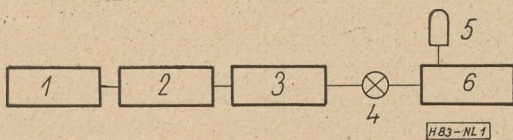
1. ábra. Az ultravákum előállításának tömbvázlata. 1—elővákuum szivattyú; 2—olajdiffúziós szivattyú; 3—speciális kifagyasztó; 4—ultravákumszelep; 5—Bayard—Alpert-féle ionizációs mérő; 6—vákuumrendszer
