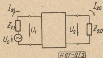
3. ábra. Hullámimpedanciájával lezárt négypólus
