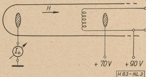
3. ábra. Houston-féle ionizációs mérő
