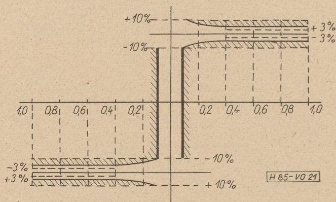
21. ábra. CCIR tűrési diagram négyszögfeszültség átviteléhez
