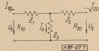
7. ábra. Illesztő T-kapcsolás
