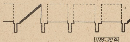
14. ábra. Négy soronkénti periodicitású jel, mely három sorban fekete vagy fehér szintet, a negyedik sorban pedig linearitásméréshez alkalmazott jelet tartalmaz
