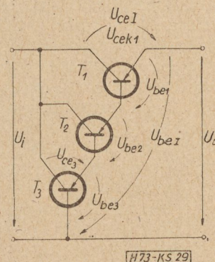
29. ábra. Az emitterkövetőlánc „könyökfeszültsége”
