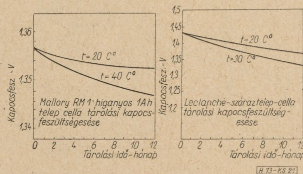
21. ábra. Száraztelepek tárolási kapacitásváltozása
