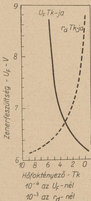
25. ábra. A Zener-feszültség és az r_d hőmérséklet-függése
