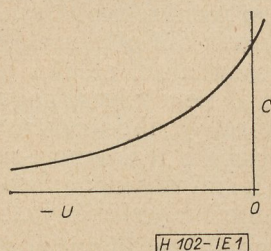
1. ábra. Parametrikus diódák jellegzetes kapacitásváltozása az előfeszültség függvényében
