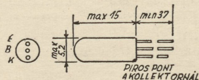
Az OC 1070 OC 1071 OC 1075 tranzisztorok külalakrajza
