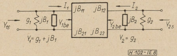
8. ábra. Nonlineáris kapacitás mint 4-pólus a bemeneti és kimeneti áramkörökkel; az Y_2 helyesen = g_2 + jB_2
