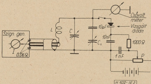
2. ábra. A nemlineáris kapacitás mérésére használt vizsgáló áramkör. (Nagy kapacitású dióda mérésénél a 10 pF kapacitás rövidre volt zárva.)
