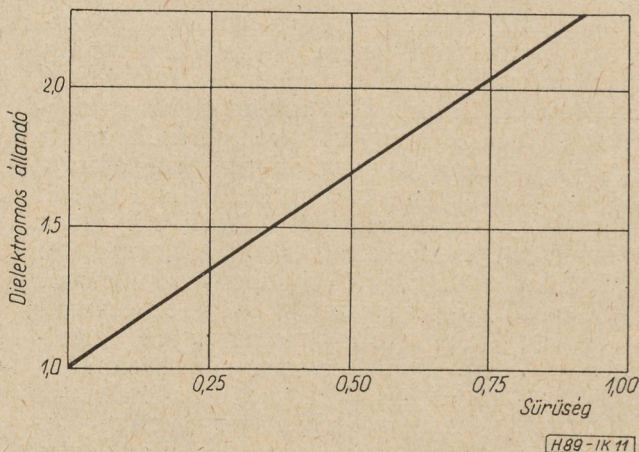
11. ábra. Hab pet dielektromos állandója a sűrűség függvényében
