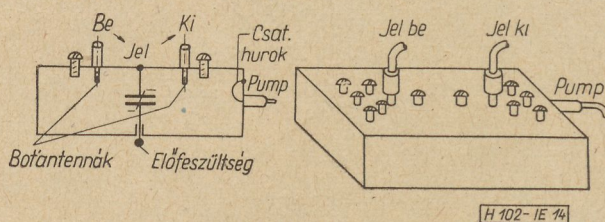
14. ábra. Három frekvenciára hangolt kísérleti üregrezonátor
