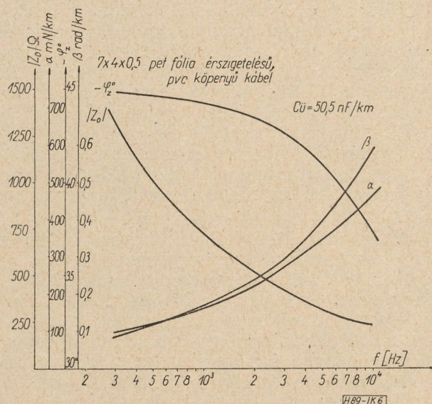
6. ábra. 7 \times 4 \times 0,5 szerkezetű pet fólia érszigetelésű kábel átviteli értékei
