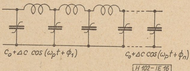
16. ábra. Haladó hullámú vonal megfelelő fáziseltolással gerjesztett nonlinearis kapacitásokkal
