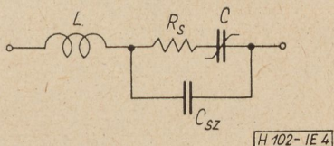
4. ábra. Előfeszített dióda helyettesítő áramkör
