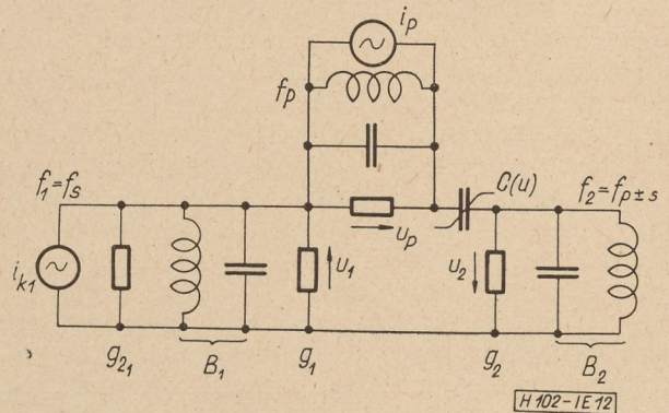
12. ábra. Paralel rezgőkörök soros kapcsolása nemlineáris kapacitás esetén; g_{21} helyesen g_{11}
