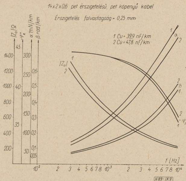
9. ábra. 14x2x0,6 szerkezetű pet érszigetelésű kábel átviteli értékei. Az érszigetelés falvastagsága 0,25 mm
