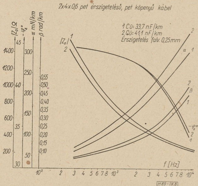
8. ábra. 7 \times 4 \times 0,6 szerkezetű pet érszigetelésű kábel átviteli értékei. Az érszigetelés falvastagsága 0,25 mm
