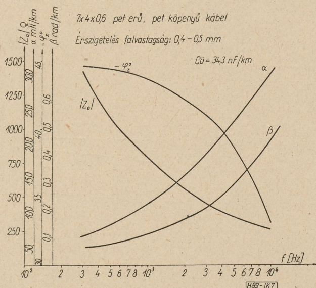
7. ábra. 7 \times 4 \times 0,6 szerkezetű pet érszigetelésű kábel átviteli értékei. Az érszigetelés falvastagsága 0,4–0,5 mm
