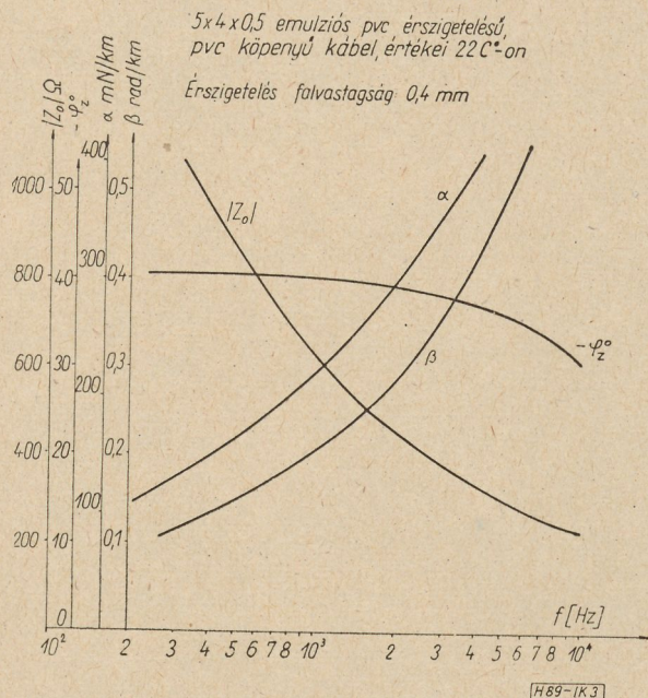
3. ábra. Emulziós polimér pvc-vel készült pvc falikábel átviteli értékei
