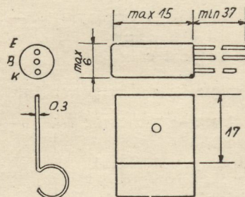
Az OC 1072 OC 1076 OC 1077 tranzisztorok külalakrajza
