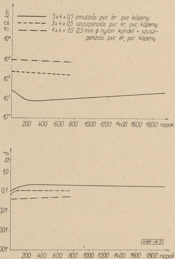
2. ábra. Pvc érszigetelésű és pvc köpenyű kábelek szigetelési ellenállás és \text{tg } \delta értékeinek változása a vízbeáztatási idő függvényében
