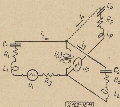
11. ábra. Soros rezgőkörök párhuzamos kapcsolása nemlineáris induktivitás esetén
