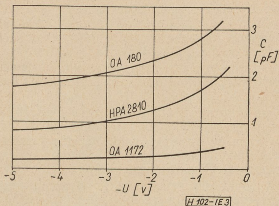
3. ábra. Néhány bemért dióda kapacitás-feszültség karakterisztikája
