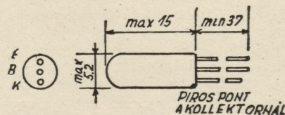
Az OC 1070, OC 1071 és OC 1075 tranzisztorok külalakrajza
