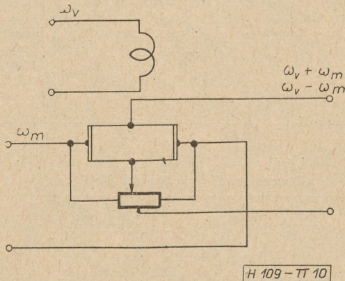
10. ábra. Hall-modulátor
