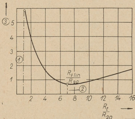
7. ábra. Szorzási hibagörbe. 1 — szorzási hiba teljesítmény illesztésnél; 2 — minimális szorzási hiba ( R_t = R_{tlin} ); 3 — szorzási hiba %
