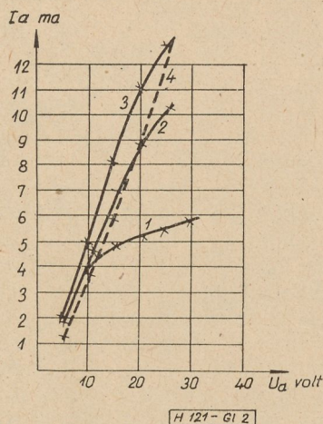
2. ábra. A katód terhelési görbéi különböző hőfokokon. 1 — U_f = 5 V, T_{szines} = 820 °C; 2 — U_f = 6,3 V, T_{szines} = 920 °C; 3 — U_f = 7 V, T_{szines} = 980 °C; 4 — I_a = f(U_a) a 3/2 törvény szerint
