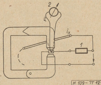
12. ábra. Teljesítménymérés Hall-generátorral. 1 — előtét; 2 — közvetlenül mutató teljesítménymérő
