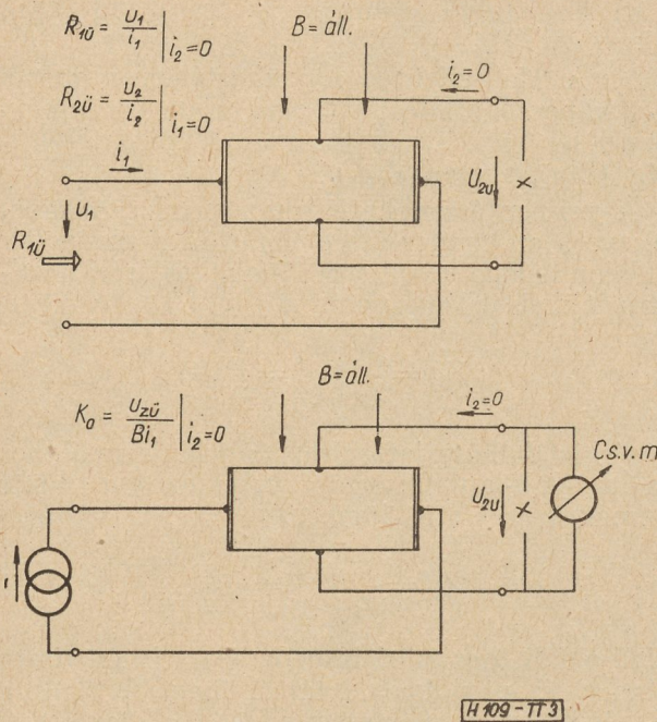
3. ábra. Az üresjárás ellenállások és az üresjárás érzékenység mérése
