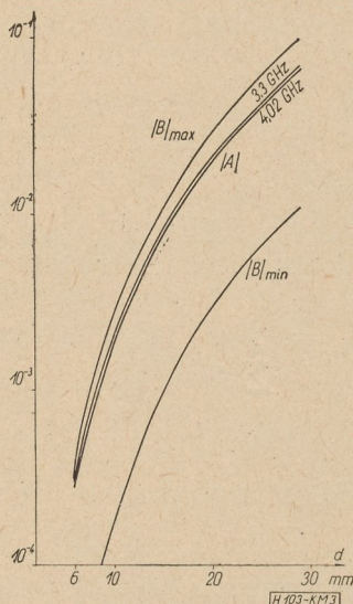
3. ábra. Az A , ill. B csatolási tényezők változása a frekvencia függvényében különböző lyukátmérők esetén
