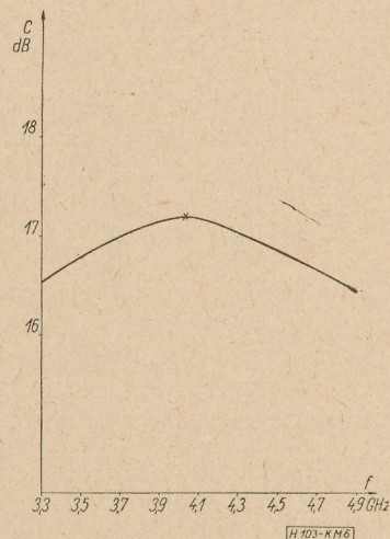
6. ábra. Az optimális csatolású iránycsatoló csatolásának változása a frekvencia függvényében
