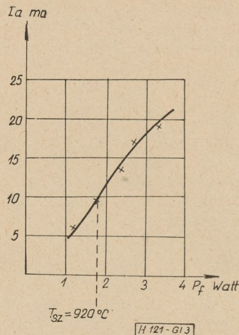
3. ábra. A katód effektivitás-görbéje 20 V anód-feszültségnél
