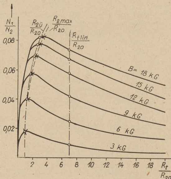
8. ábra. Teljesítményátvitel a relatív terhelés függvényében
