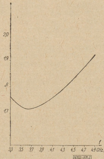
2. ábra. A csatolás változása, ha a lyuk a csőtápvonal széles oldalának egynegyedében helyezkedik el
