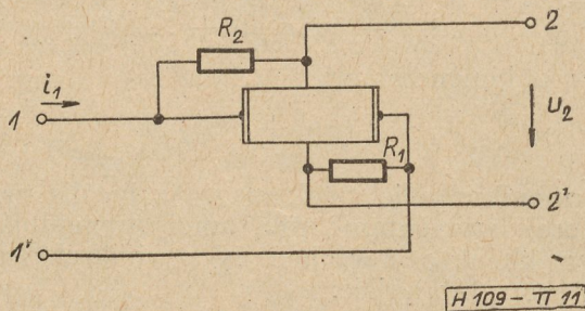
11. ábra. Hall-izolátor
