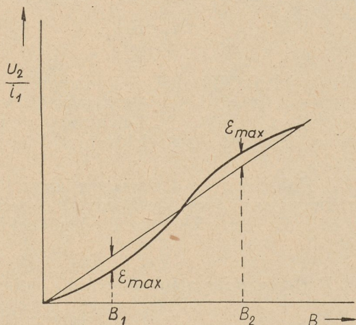
6. ábra. \frac{u_2}{i_1} jelleggörbe és közelítése
