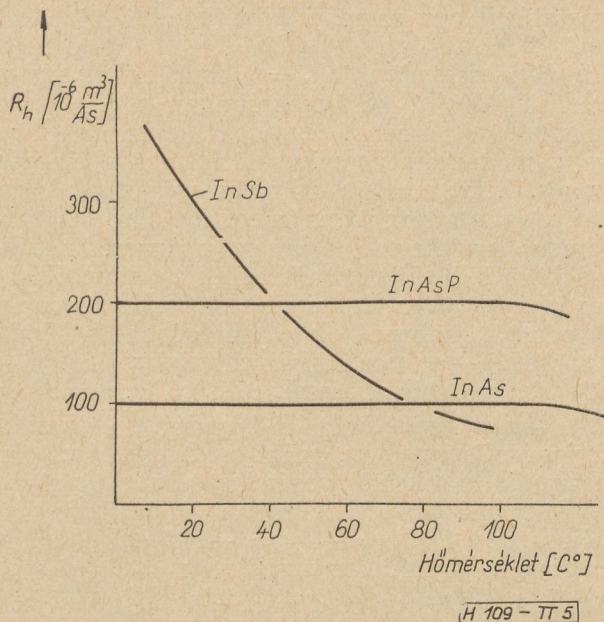
5. ábra. Néhány intermetallikus félvezető Hall-állandójának hőmérsékletfüggése
