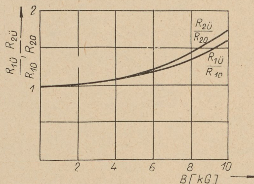
2. ábra. Az üresjárási ellenállások változása a mágneses indukció függvényében
