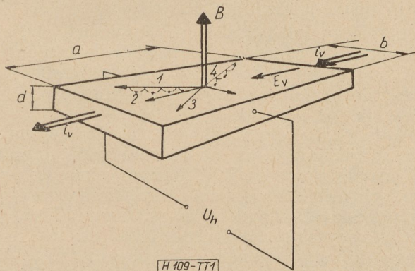
1. ábra. Hall-jelenség; 1 — lyukáram; 2 — lyukpálya; 3 — elektronáram; 4 — elektronpálya
