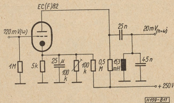
11. ábra. Sokszorozó egység
