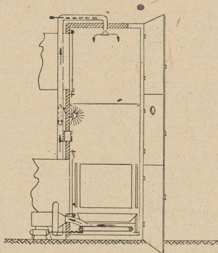
4. ábra. Porvizsgáló szekrény
