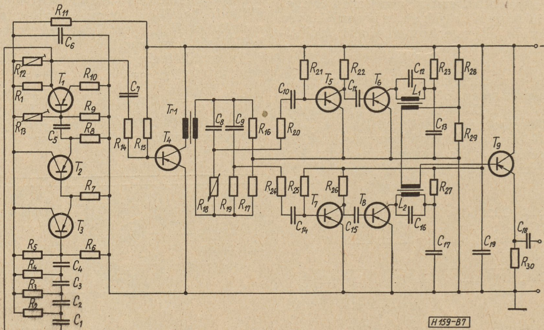
7. ábra. A teljes adó kapcsolási vázlata
