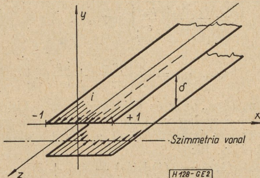
2. ábra. A szimmetrikus vonal és a koordináta rendszer elhelyezése
