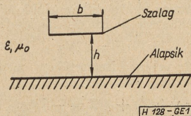
1. ábra. A szalagtápvonal keresztmetszete
