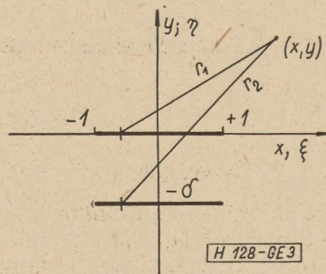
3. ábra. A vizsgált pont és az áramszálak közötti távolság meghatározásához
