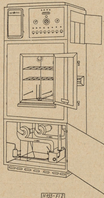
2. ábra. Nedvesmelegvizsgáló-szekrény
