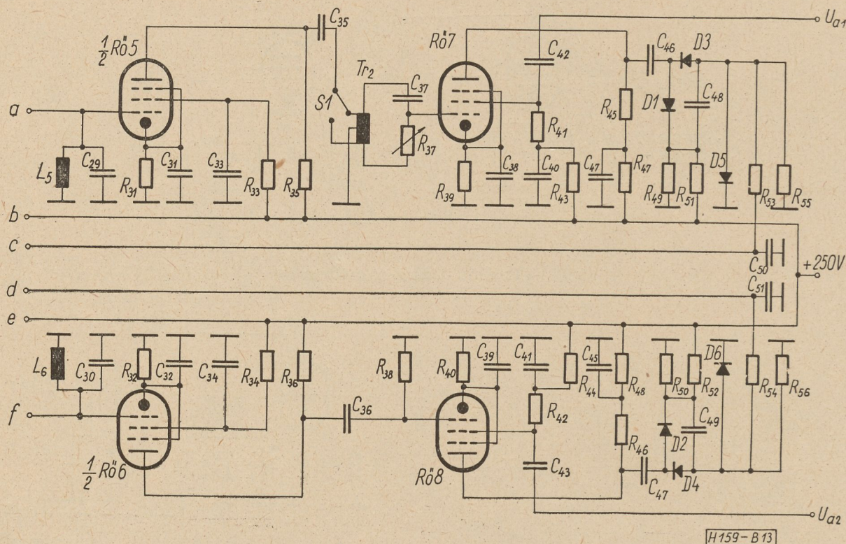
13. ábra. A teljes vevőrészek kapcsolási vázlat. II. rész
