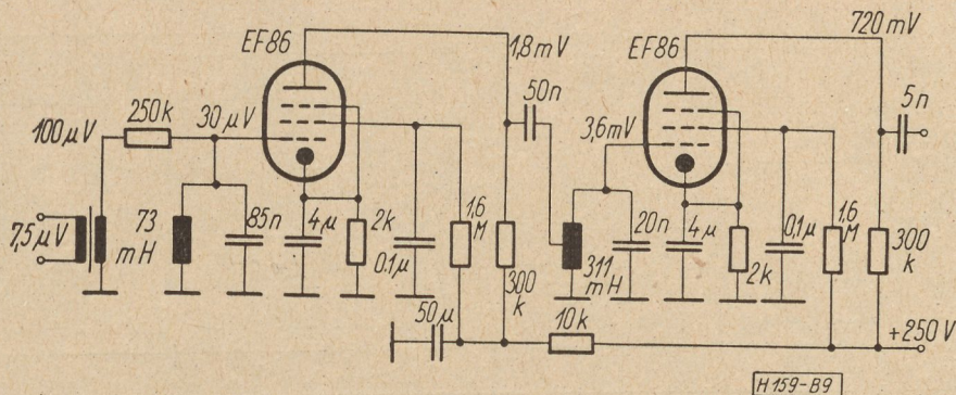
9. ábra. 2 kHz-es csatorna
