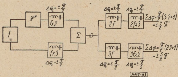
3. ábra. Az átviteli rendszer fázishibája
