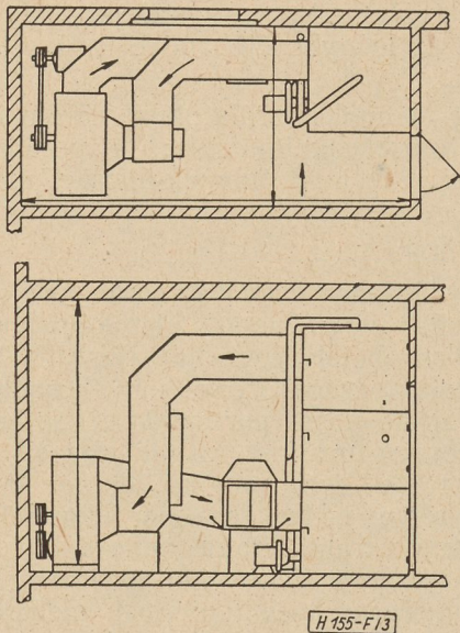
3. ábra. Por-homokvizsgáló berendezés A felső ábra az alaprajzi elrendezést ( 2,2 \times 5,0 m), az alsó az előlnézetet mutatja (magasság 3,2 m)
