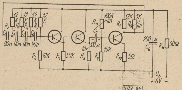
4. ábra. Tranzisztoros oszcillátor
