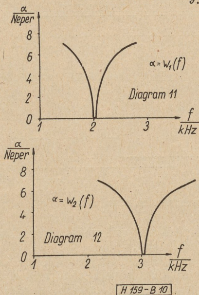
10. ábra. 2 és 3 kHz-es csatornák szelektivitásgörbéi
