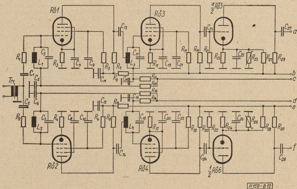
12. ábra. A teljes vevőrész kapcsolási vázlatja I. rész.
