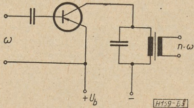
5. ábra. A tranzisztoros frekvenciasokszorozító elve
