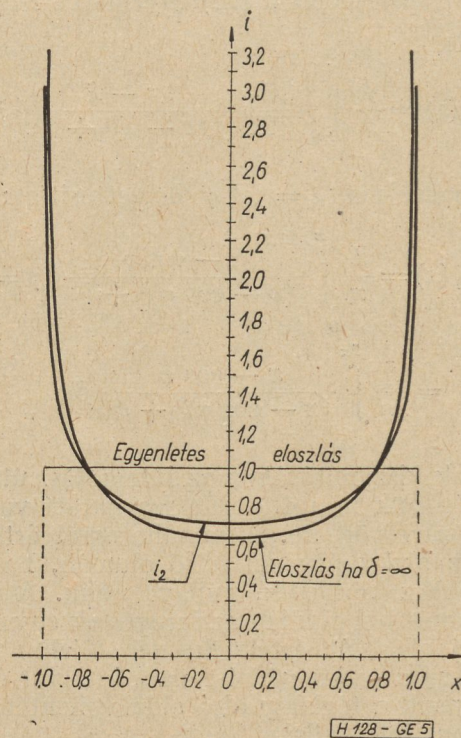
5. ábra. Árameloszlás a szalagon
