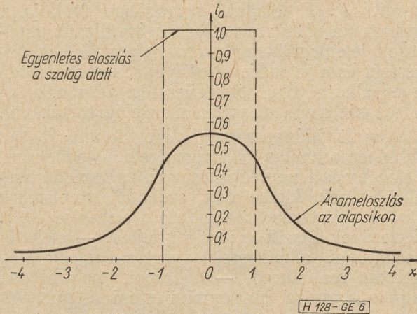
6. ábra. Árameloszlás az alapsíkon
