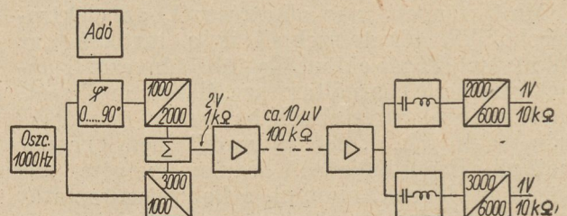
2. ábra. A mérőberendezés tömbvázlata
