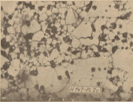
2c ábra. Előégetés 5 órán át, 1000 C°-on, őrlés 24 órán át, végső égetés 5 órán át, 1350 C°-on
