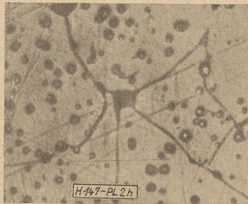
2h ábra. Előégetés 10 órán át 1000 C°-on, őrlés 72 órán át, végső égetés 5 órán át, 1350 C°-on
