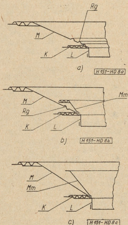
8. ábra. Különböző hangszóró-membrán megoldások
