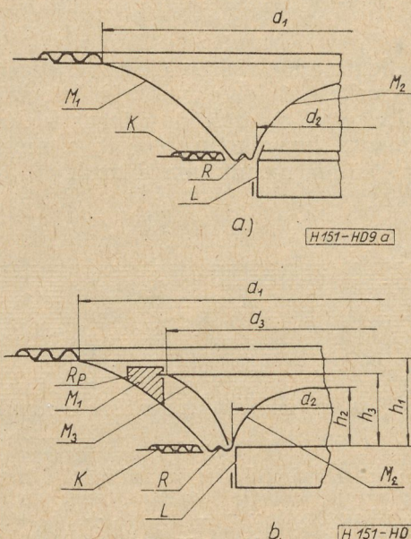
9. ábra. Szélessávú hangszóró-membrán megoldások
