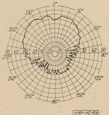
11b ábra. H_c típusú 160 mm átmérőjű hangszóró irányjelleggörbéje f = 4 kHz-en, R_p csillapítógyűrűvel
