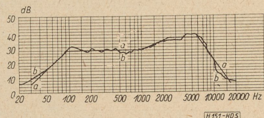
5. ábra. a — H_b típusú, 160 mm átmérőjű hangszóró javasolt tengelybeli hangnyomás jelleggörbéje; b — H_b típusú 160 mm átmérőjű hangszóró tengelybeli hangnyomás jelleggörbéje; U = \text{áll.}
