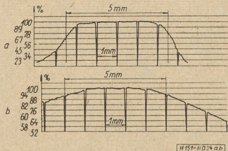
24. ábra. a — a légrésindukció eloszlása egy 5 mm vastag fedőlappal, 20 mm átmérőjű vasmaggal felépített mágneskör légrésében, 1,1 mm légréshossz mellett. B_1 = 0,9 Vsm -2 ; b — egy, a fenti légrésben mozgó 8 mm hosszú lengőtekeresre ható erő csökkenése a lengőtekeres elmozdulásának függvényében
