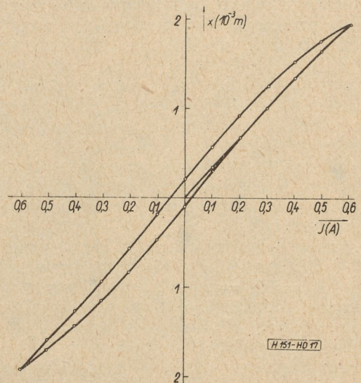
17. ábra. 160 mm átmérőjű hangszóró lengőrendszerének elektromechanikai hiszterézisgörbéje (elmozdulás a lengőtekercsben folyó áram függvényében)
