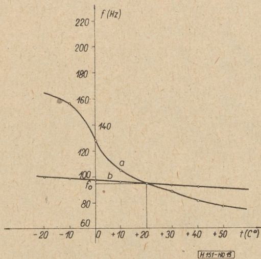
15. ábra. a — 160 mm átmérőjű, Standoplasttal kezelt membránszerű hangszóró rezonanciafrekvenciájának hőfokfüggése; b — ugyanaz, szilikonkaucsuk-polimerizátummal kezelve
