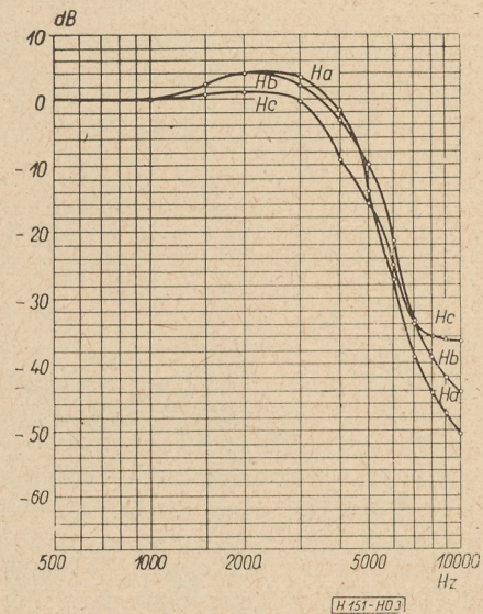
3. ábra. H_a , H_b , H_c típusú hangszórók javasolt tengelybeli hangnyomás jelleggörbéje f \geq 0,5 kHz felett, az 1. ábrán látható a jelleggörbéjű erősítőről táplálva
