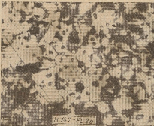
2e ábra. Előégetés 5 órán át, 800 C°-on, őrlés 72 órán át, végső égetés 5 órán át, 1350 C°-on
