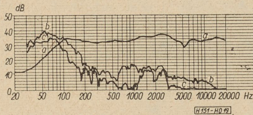
19. ábra. a — 160 mm-es átmérőjű, H_c típusú hangszóró tengelybeli hangnyomás jelleggörbéje U = 4 \text{ V} áll. mellett; b és c — az első és a második felharmonikus jelleggörbéje a ténylegesnél 20 dB-el nagyobb szinten feljegyezve
