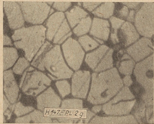
2g ábra. Előégetés 5 órán át, 1000 C°-on, őrlés 72 órán át, végső égetés 5 órán át, 1350 C°-on
