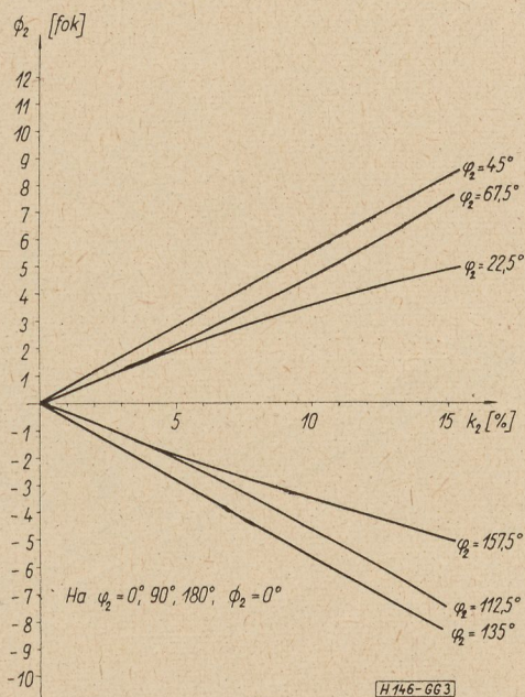
3. ábra. A járulékos fáziseltolást kifejező görbék második harmonikus tartalom esetén
