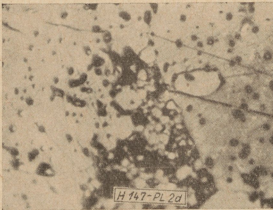
2d ábra. Előégetés 10 órán át 1000 C°-on, őrlés 24 órán át, végső égetés 5 órán át, 1350 C°-on
