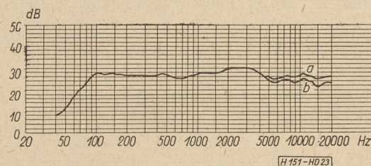
23. ábra. a — Hc típusú, 160 mm átmérőjű r rövidrezáró gyűrűvel ellátott hangszóró tengelybeli hangnyomás jelleggörbéje U = \text{áll. feszültségű generátorról táplálva} ; b — ugyanaz, de rövidrezáró gyűrű nélkül
