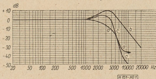
1. ábra. a — két fokozatú KF erősítő jellegzetes átviteli jelleggörbéje; b — keskenysávú hangszóró javasolt tengelybeli hangnyomás jelleggörbéje; c — az előbbi KF erősítőről táplált keskenysávú hangszóró tengelybeli hangnyomás jelleggörbéje
