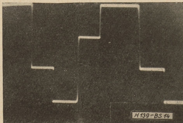
14. ábra A 13. ábrán vázolt kapcsolás kimenő jele
