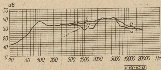
13. ábra. a — Hc típusú, 160 mm átmérőjű hangszóró tengelybeli hangnyomás jelleggörbéje, a membránszél csillapítása nélkül; b — ugyanaz csillapítással
