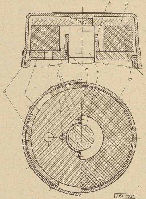
21. ábra. A hangszóró mágneskörének kialakítása. A mágnes báriumferrit gyűrűmágnes
