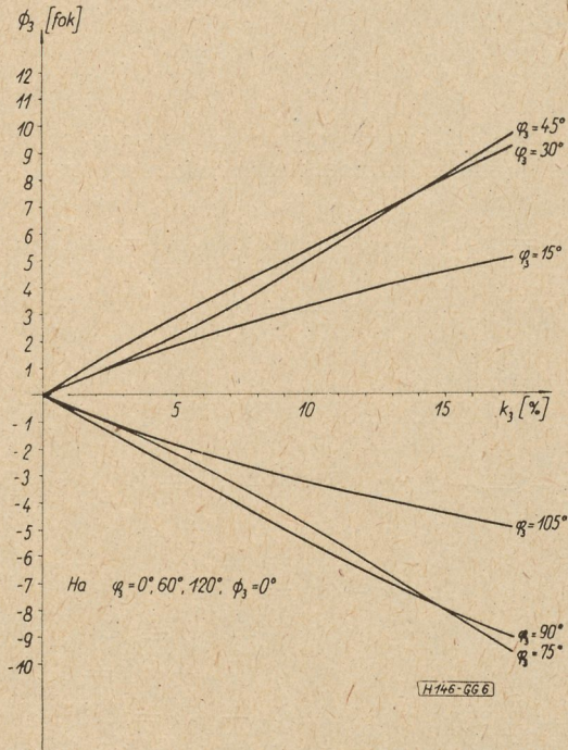
6. ábra. A járulékos fáziseltolást kifejező görbék harmadik harmonikus tartalom esetén
