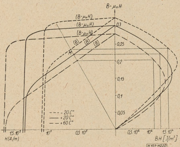
20. ábra. Anizotróp báriumferrit-mágnes jellegzetes mágnesezési görbéi T = -20; +20; +60 \text{ }^\circ\text{C} hőmérsékleten
