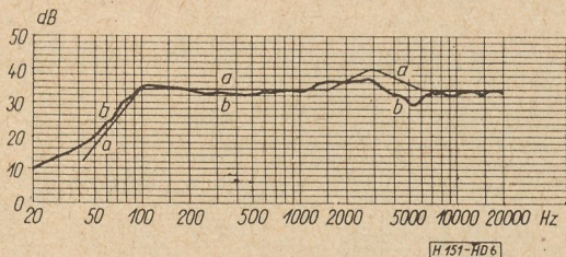
6. ábra. a — Hc típusú, 160 mm átmérőjű hangszóró javasolt tengelybeli hangnyomás jelleggörbéje; b — Hc típusú 160 mm átmérőjű hangszóró tengelybeli hangnyomás jelleggörbéje; U = \text{áll.}
