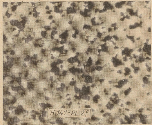
2f ábra. Előégetés 5 órán át, 900 C°-on, őrlés 72 órán át, végső égetés 5 órán át, 1350 C°-on
