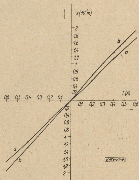
18. ábra. A hangszórók elektromechanikai szűzgörbéje; a — 130 mm-es, hangszóró; b — 160 mm-es hangszóró
