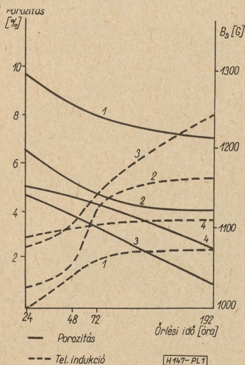
1. ábra. A porozitás és a telítési indukció az őrlési idő függvényében. 1—5 óra, 800 C°; 2—5 óra, 900 C°; 3—5 óra, 1000 C°; 4—10 óra, 1000 C°
