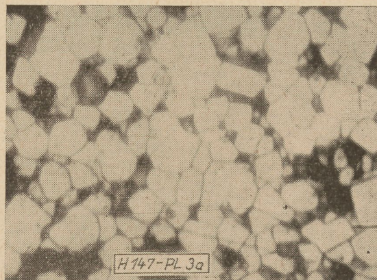
3a ábra. Végső égetés 2 órán át, 1350 C°-on
