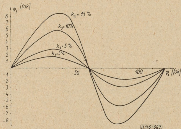
7. ábra. A járulékos fáziseltolást kifejező görbék harmadik harmonikus tartalom esetén
