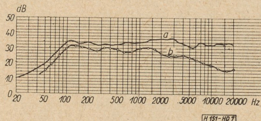
7. ábra. a — Hc típusú, 160 mm átmérőjű hangszóró tengelybeli hangnyomás jelleggörbéje; U = \text{áll.} ; b — a hangszóró elsugárzott teljesítmény-jelleggörbéje; U = \text{áll.}
