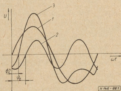
1. ábra. Második harmonikus tartalom által okozott fáziseltolás
