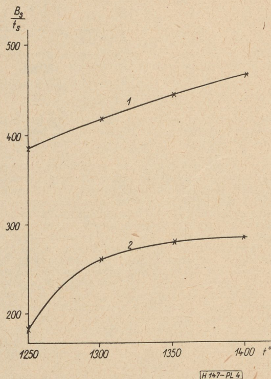
4. ábra. Tömörségre korrigált két ferrit típus telítési indukciója az égetési körülmények függvényében: 1- Mg_{1,4}Mn_{0,2}Fe_{1,4}O_4 ; 2- Mg_1Mn_{0,1}Al_{0,6}Fe_{1,3}O_4
