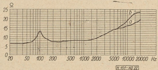
22. ábra. a — Hc típusú, 160 mm átmérőjű hangszóró impedanciája abszolút értékének jelleggörbéje, r rövidrezáró gyűrűvel; b — ugyanaz, de rövidrezáró gyűrű nélkül
