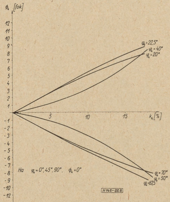
8. ábra. A járulékos fáziseltolást kifejező görbék negyedik harmonikus tartalom esetén
