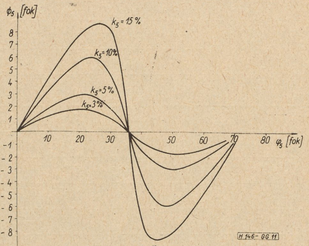
11. ábra. A járulékos fáziseltolást kifejező görbék ötödik harmonikus tartalom esetén
