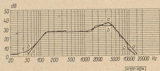
4. ábra. a — H_a típusú 130 mm átmérőjű hangszóró javasolt tengelybeli hangnyomás jelleggörbéje; b — H_a típusú 130 mm-es átmérőjű hangszóró tengelybeli hangnyomás jelleggörbéje; U = \text{áll.}
