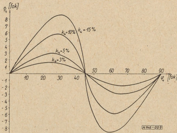
9. ábra. A járulékos fáziseltolást kifejező görbék negyedik harmonikus tartalom esetén
