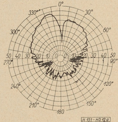
11a ábra. H_c típusú, 160 mm átmérőjű hangszóró irányjelleggörbéje f = 4 kHz-en
