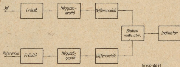
2. ábra. Impulzustechnikai elven működő fázisszögmérési eljárás működési vázlata
