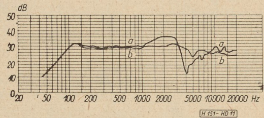
11. ábra. a — H_c típusú, 160 mm átmérőjű hangszóró tengelybeli hangnyomás jelleggörbéje az R_p csillapító gyűrű nélkül; b — ugyanez csillapítógyűrűvel
