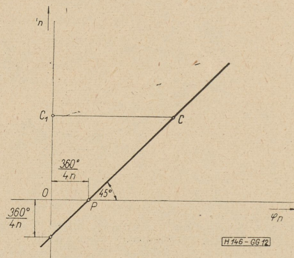
12. ábra. A járulékos fáziseltolást kifejező görbék csúcspontjait összekötő egyenes
