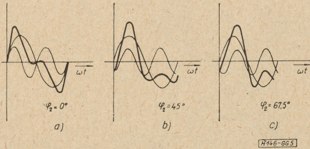
5. ábra. Az eredő görbe megszerkesztése különböző fázishelyzetű második harmonikus tartalom esetén
