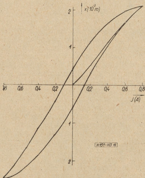
16. ábra. 130 mm átmérőjű hangszóró lengőrendszerének elektro-mechanikai hiszterézisgörbéje (elmozdulás a lengőtekercsben folyó áram függvényében)
