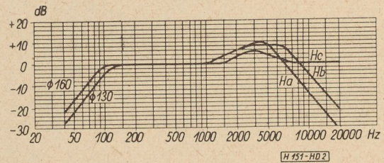
2. ábra. H_a , H_b , H_c keskeny, közepes-, szélessávú hangszóró névleges tengelybeli hangnyomás jelleggörbéje
