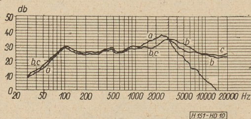
10. ábra. a — Hc típusú, 160 mm átmérőjű hangszóró M_1 membránja keltette sugárzás tengelybeli hangnyomás jelleggörbéje; b — az M_1 + M_3 membrán sugároz; c — az M_1 + M_2 + M_3 membránok sugárzásának eredője
