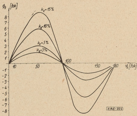
4. ábra. A járulékos fáziseltolást kifejező görbék második harmonikus tartalom esetén
