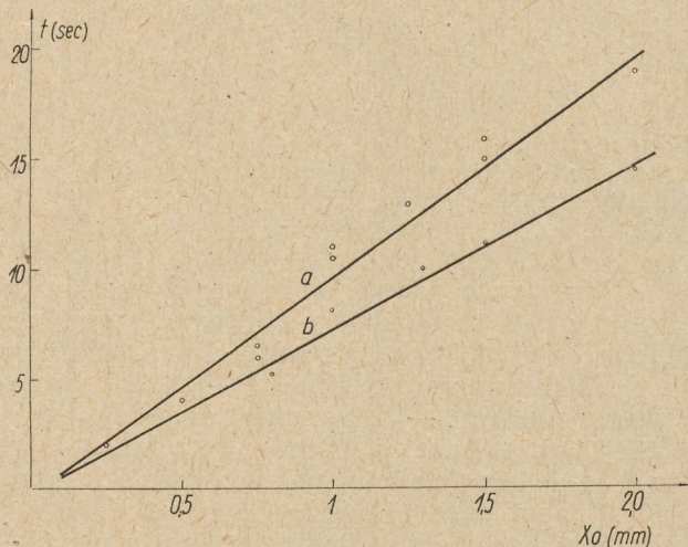
14. ábra. a — 160 mm átmérőjű hangszóró membránjának relaxációs ideje, Standoplasttal kezelt membránszéllel; b — ugyanaz, csak szilikon-kaucsuk polimerizátummal kezelt membránszéllel
