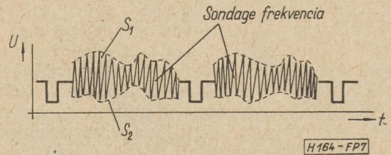
7. ábra. DM rendszer képvívójét moduláló videojel
