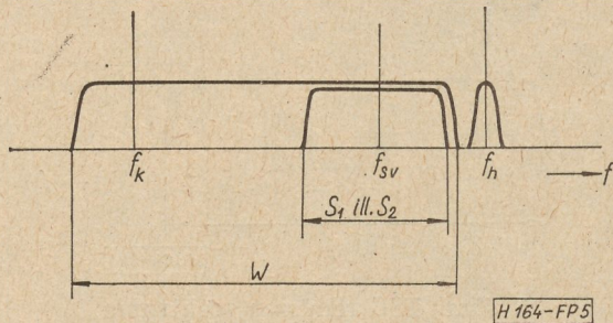
5. ábra. SECAM rendszer spektruma
