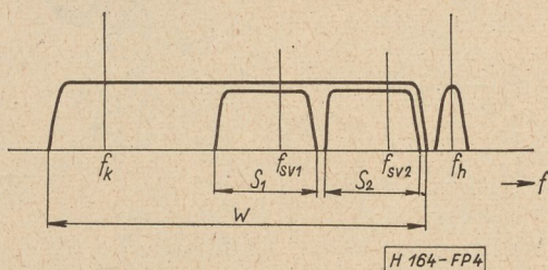
4. ábra. TSC rendszer spektruma
