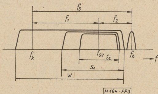
3. ábra. NTSC rendszer spektruma
