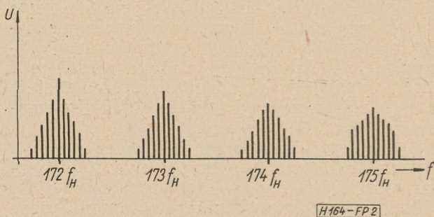
2. ábra. Video-jel spektrumának egy részlete. f_H = vízszintes eltérítő frekvencia
