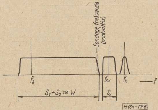
6. ábra. DM rendszer spektruma
