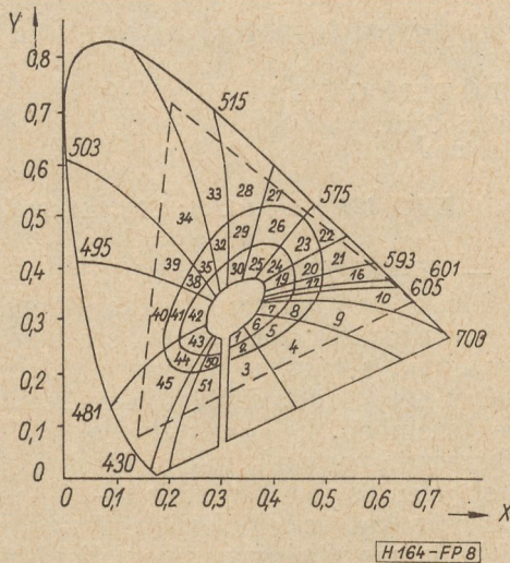
8. ábra. A színszektorok elhelyezkedése a színdiagrammon
