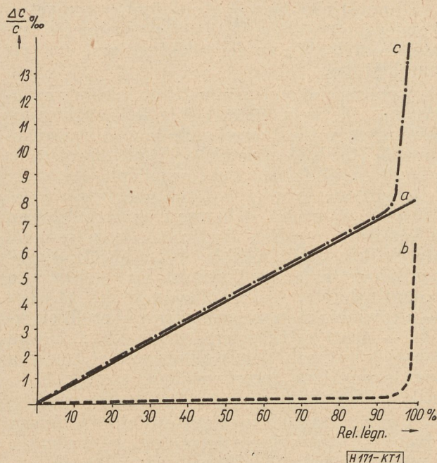
1. ábra. A száraz kondenzátor kapacitásváltozása a relatív légnedvesség függvényében az egyensúlyi állapot elérése után akkor, ha a légrés 0–0,2 \mu között lineárisan változik, és a légrések szennyezettségének hatásától eltekintünk. A térfogati nedvesség hatását az a, a légrésnedvesség hatását a b, a nedvesség következtében fellépő összes kapacitásváltozást a c görbe tünteti fel. E görbék számított értékek alapján készültek
