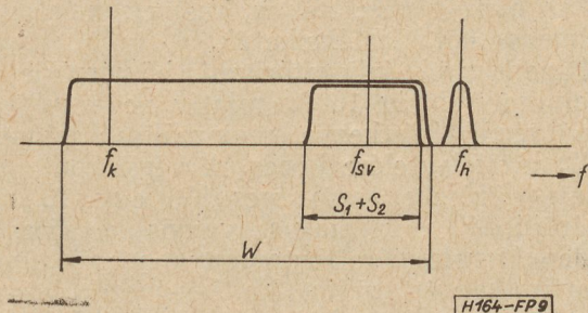
9. ábra. Kód rendszer spektruma
