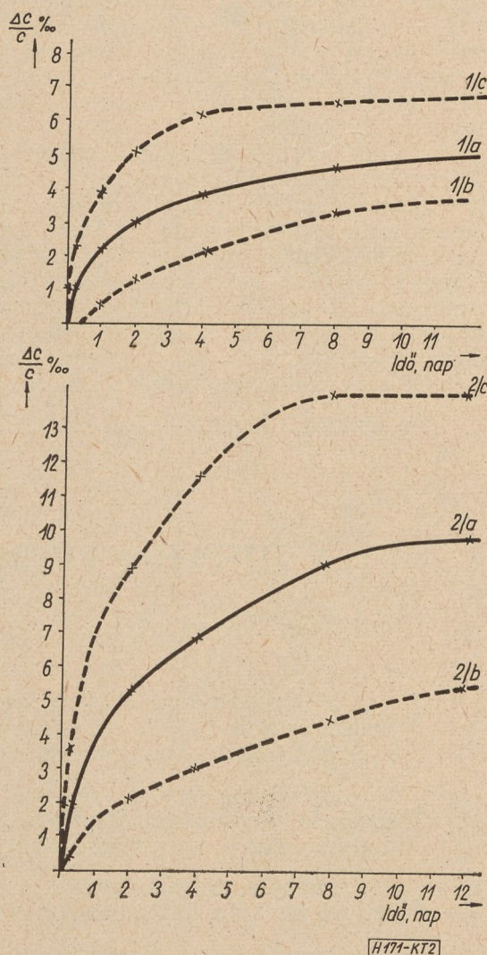
2. ábra. 250 V névleges feszültségű, 1 nF-os, huzalkivezetéses polisztirolkondenzátorok kapacitásváltozása akkor, ha a környezet relatív nedvességtartalma 45%-ról 83%-ra ( 1/a-c görbék), ill. 98,5%-ra ( 2/a-c görbék) nő meg (hőmérséklet 25 \pm 2^\circ\text{C} ). Az átlagértékeknek megfelelő görbéket a -val, a legkisebb, ill. legnagyobb változást mutató kondenzátorok kapacitását megadó görbéket b -vel, ill. c -vel jelöltük
