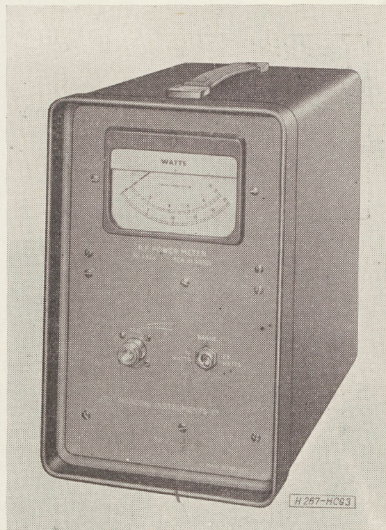
3. ábra. Marconi TF 1152 A-típusú, közvetlenül leolvasható abszorpciós típusú teljesítménymérő. Méréshatár 25 watt, egyenáramtól 500 MHz-ig használható. A bemeneti impedancia 50 ohm vagy 75 ohm
