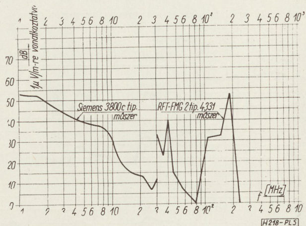
5. ábra. A nagyfrekvenciás zavar spektruma a távvezeték 290. sz. oszlopának tövében, 1962. IX. 4-én 11.15–12.00 időben. Az oszlopon egy szigetelőlánc 4 tagja mesterségesen roncolt. Ezen ábra a 4. ábra karakterisztikájának folytatása a nagyobb frekvenciák felé
