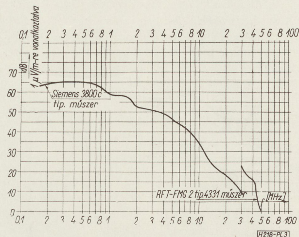
3. ábra. A nagyfrekvenciás zavar spektruma a távvezeték 288. sz. oszlopának tövében. 1962. IX. 4. 15.00–17.30 időben. Valamennyi szigetelőtag ép
