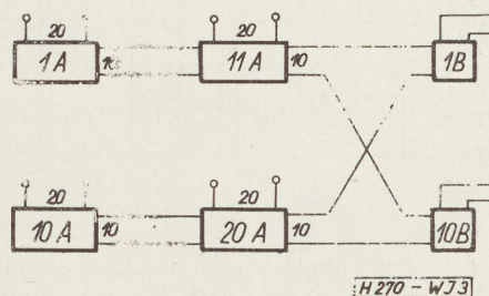
3. ábra. 4 \times 10 -es kapcsológépek
