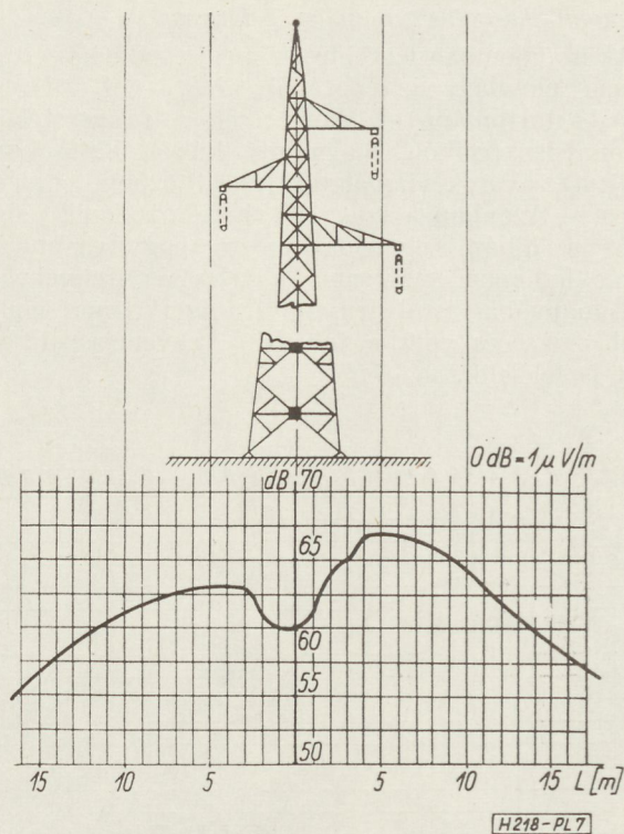
7. ábra. Zavar szint változás a nyomvonalra merőlegesen, a 289. és 290. sz. oszlopok között, 1962. IX. 5-én 11.00—11.30 időben. Mérési frekvencia: 0,245 MHz
