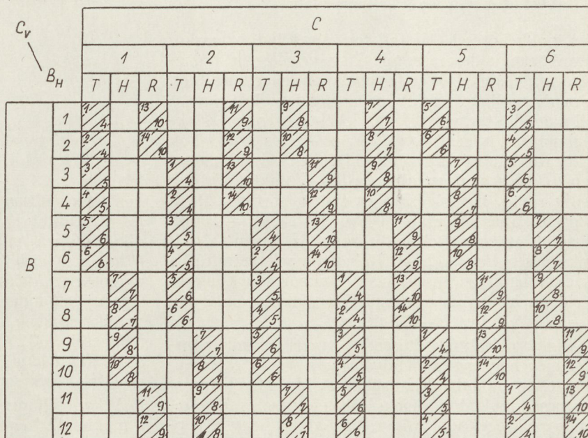
8. ábra. B—C linkbekötés
