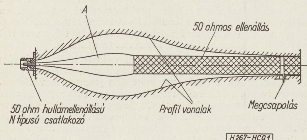
1. ábra. Rádiófrekvenciás rezisztív terhelés, amelynél a belső vezető két szimmetrikusan elhelyezett, megfelelően kialakított felület fogja közre
