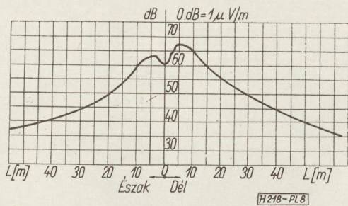
8. ábra. Zavar szint változás a nyomvonalra merőlegesen, a 289. és 290. sz. oszlopok között, 1962. IX. 5-én 11.00—11.30 időben
