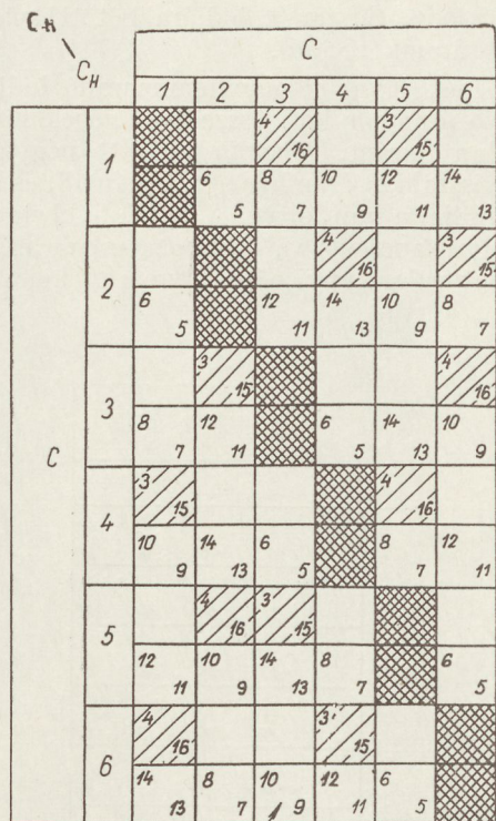
9. ábra. C—C linkbekötés
