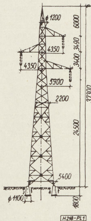
1. ábra. Sajószöged—Zugló II. távvezetéken alkalmazott oszlop méretvázlata
