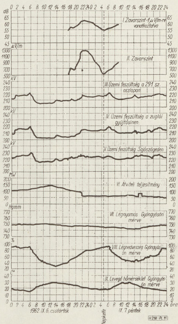
11. ábra. Zavarsszint mérés a távvezeték 291—292. sz. oszlopai között, 350 kHz frekvencián, a legközelebbi fázisvezetőtől 20 m távolságban. Alatta a vezeték feszültség és terhelési viszonyai és a környezet meteorológiai adatai
