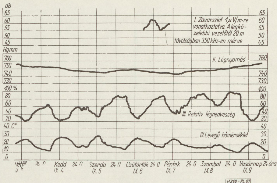
10. ábra. A távvezeték 291. és 292. sz. oszlopai között 1962. IX. 6—7-én mért zavarsszint és az 1962. IX. 3—9 közötti hét Gyöngyösön felvett meteorológiai adatai
