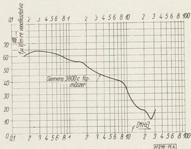
4. ábra. A nagyfrekvenciás zavar spektruma a távvezeték 290. sz. oszlopának tövében, 1962. IX. 4-én 11.15–12.10 időben. Az oszlopon egy szigetelőlánc 4 tagja mesterségesen roncolt
