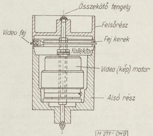
9. ábra. Videódob felépítése (Loewe Opta után)
