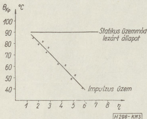
3. ábra. A \theta_{kv} — kritikus tok-hőmérséklet ábrázolása az \eta -tényező függvényében
