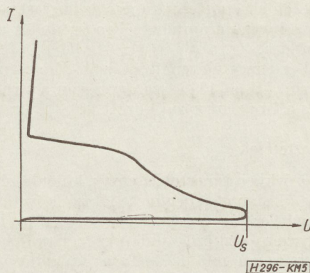
5. ábra. A négyrétegű dióda áram-feszültség karakterisztikája
