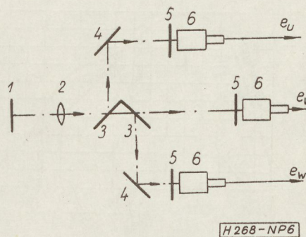
6. ábra. Háromfelvevőcsöves kamara; 1 — tárgy, 2 — objektív, 3 — színválasztó féligáteresztő tükrök, 4 — tükrök, 5 — korrekciós színszűrők, 6 — képfelvevő csövek
