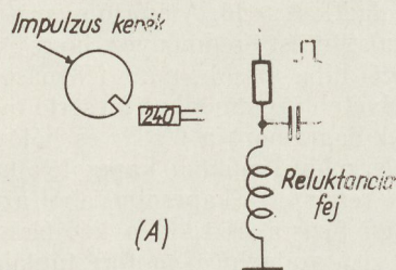
6. ábra. Az RCA impulzuskerék működése
