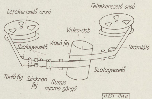
8. ábra. Loewe Opta videódob mechanizmusa (Loewe Opta után)
