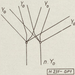
1. ábra. Illesztett elágazás
