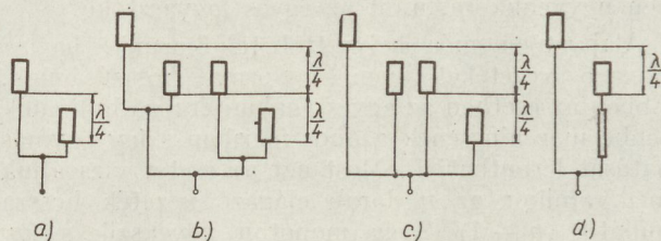
3. ábra. A fázistáplálás különböző módjainak áttekintése: a) egyszerű fázistáplálás, b) többszörös fázistáplálás, c) egyszerű, szélessávú fázistáplálás, d) fázistáplálás szélessávú fázistoló vonallal
