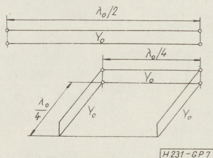
7. ábra. Szélessávú fázistoló áramkör
