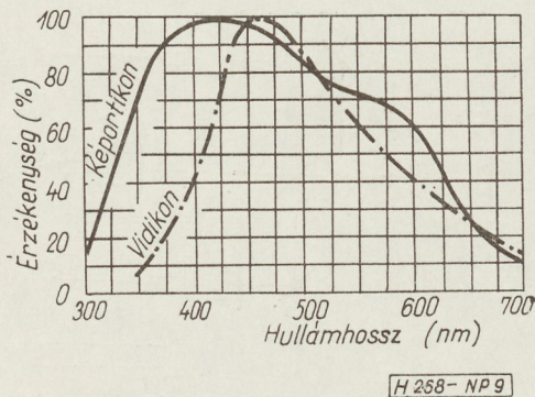
9. ábra. Képortikon és vidikon spektrális érzékenység karakterisztikái
