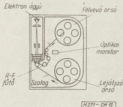
12. ábra. Egy kísérleti termoplasztikus rekorder. A film elhalad az elektronsugár alatt, hogy megkapja a töltését, majd áthalad az R-F fűtőn, ahol deformálódik (Gen. El. Co. után).
