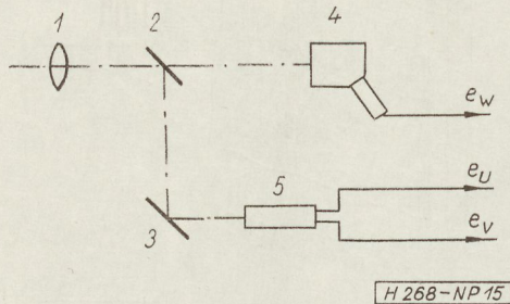
15. ábra. Kétsöves kamera; 1 — objektív, 2 — féligáteresztő tükör, 3 — tükör, 4 — képortikon 5 — kétraszteres vidikon
