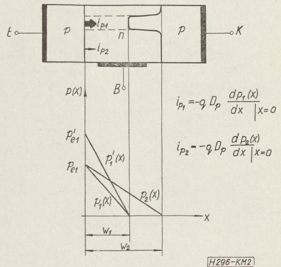
2. ábra. Lyuksűrűség-eloszlás az ötvözött tranzisztor bázisrétegének w_1 és w_2 szélességű tartományaiban
