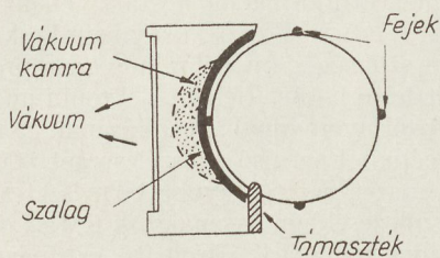
5. ábra. A vákuumvezető és videódob keresztmetszete (Ampex után)
