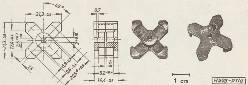
1. ábra. X-fazésmag és a hozzátartozó csévetest
