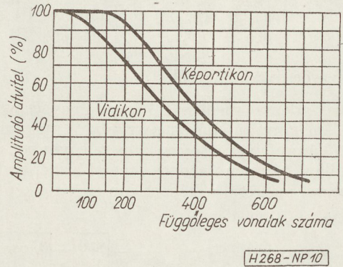
10. ábra. Képtikon és vidikon felbontása appertúrakorrektio nélkül
