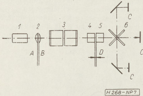
7. ábra. Háromfelvéves csöves kamara optikai rendszere; 1 — objektív készlet, 2 — juszitírozó lencserendszer, 3 — sík-párhuzamos kompenzáló lemezek, 4 — leképző lencserendszer, 5 — leképző lencserendszer, 6 — színválasztó féligáteresztő tükrök
