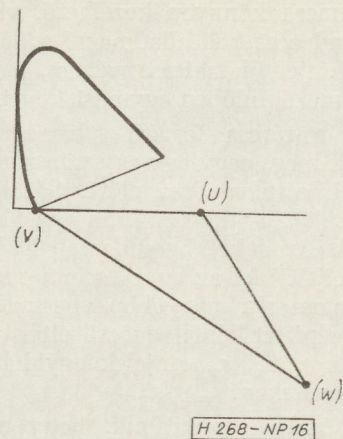
16. ábra. Kétsöves kamera alapszínpontjainak elhelyezkedése
