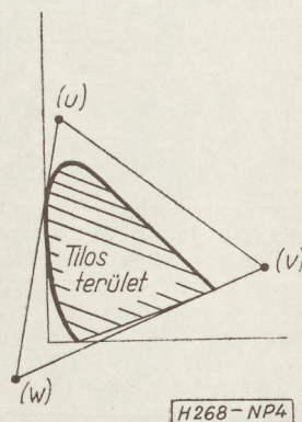
4. ábra. Képfelvételi oldal alapszíneinek elhelyezkedése
