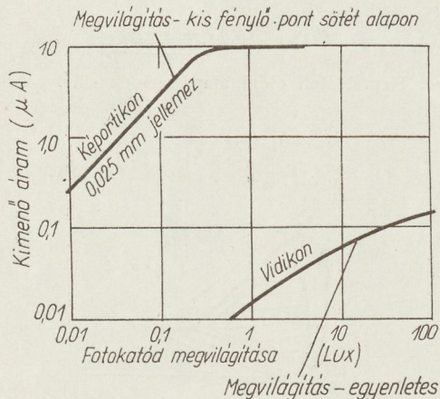
8. ábra. Képortikon és vidikon amplitúdó átviteli jelleggörbéi
