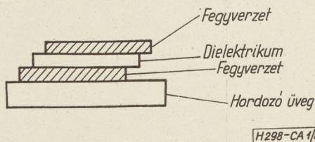
1b ábra. Gőzölt dielektrikumú kondenzátor keresztmetszetének elvi vázlata
