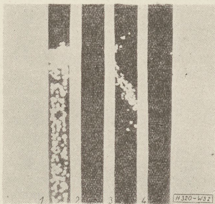
2. ábra. Gőzölt alumínium-réteg korróziója anodikus oxidációkor különböző elektrolitokban. 1 — kloridionnal szennyezett nátriumborátos elektrolitban; 2 — kloridionnal szennyezett nátriumtartarátos elektrolitban; 3 — szennyezetlen nátriumborátos elektrolitban; 4 — szennyezetlen nátriumtartarátos elektrolitban
