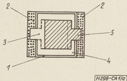
1a ábra. Gőzölt dielektrikumú kondenzátor felépítése (felülnézet). 1 — üvegbázis 2 — beégetett kontaktus; 3 — alsó fegyverzet; 4 — dielektrikum; 5 — felső fegyverzet
