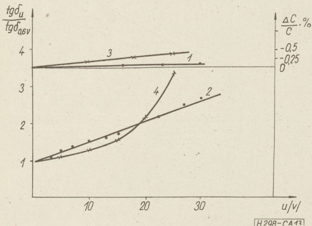
13. ábra. Gőzölt dielektrikumú kondenzátorok kapacitásának és veszteségi tényezőjének feszültségfüggése. 1 — SiO 2 dielektrikumú kondenzátorok kapacitásának feszültség függése; 2 — SiO 2 dielektrikumú kondenzátorok veszteségi tényezőjének feszültség függése; 3 — MgF 2 dielektrikumú kondenzátorok kapacitásának feszültség függése; 4 — MgF 2 dielektrikumú kondenzátorok veszteségi tényezőjének feszültség függése
