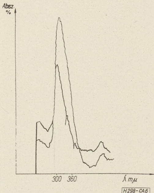
6. ábra. Üveglapra felhordott SiO ultraibolya abszorpciós spektruma. 1 — hőkezelés nélkül; 2 — 1 óra, 400 °C-os hőkezelés után
