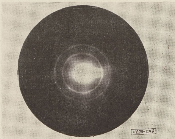
9. ábra. Párolgatott MgF 2 réteg elektrondiffrakciós felvétele 30 perc 400 °C-os hőkezelés után
