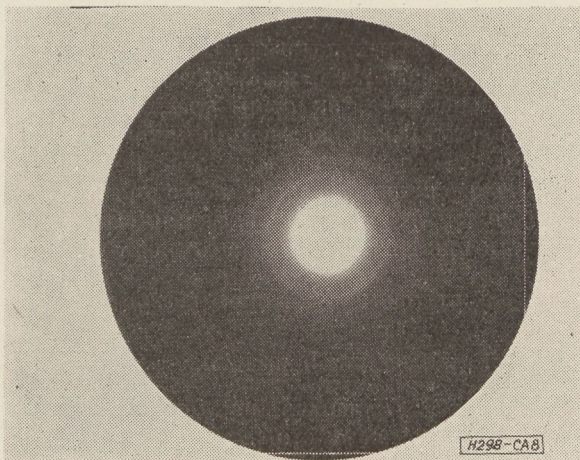
8. ábra. Párolgatott MgF 2 réteg elektrondiffrakciós felvétele közvetlenül párolgatás után
