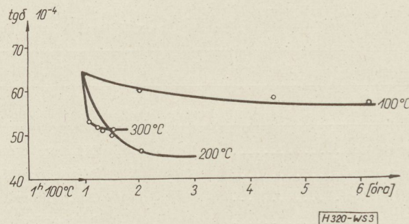
3. ábra. A kondenzátorok kapacitásának és veszteségi tényezőjének változása 100°C, 200°C és 300°C-on történő hőkezelés során a hőkezelési idő függvényében
