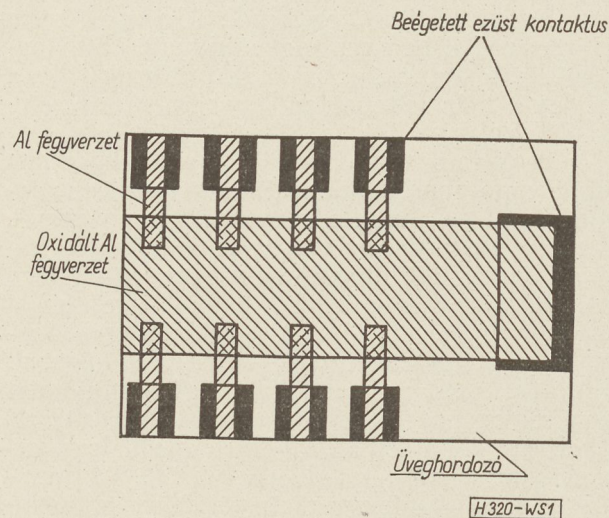
1. ábra. A kondenzátor szerkezeti felépítése, kísérleti elrendezése
