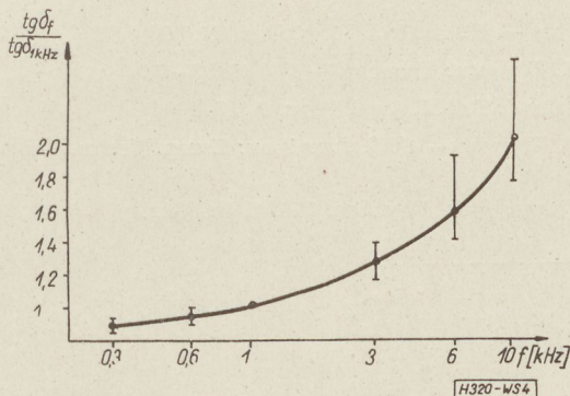
4. ábra. A kondenzátorok kapacitásának és veszteségi tényezőjének frekvenciafüggése
