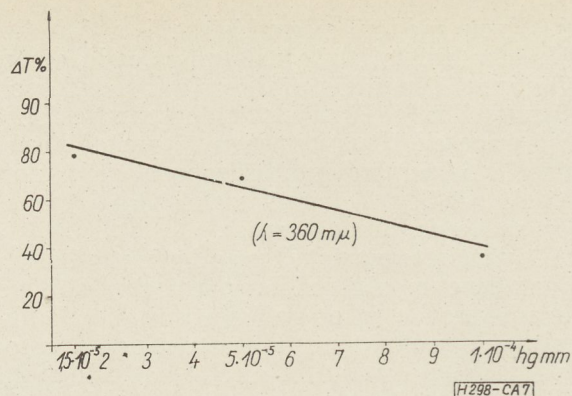
7. ábra. A fényelnyelés különbsége a párolgatásnál alkalmazott vákuum függvényében
