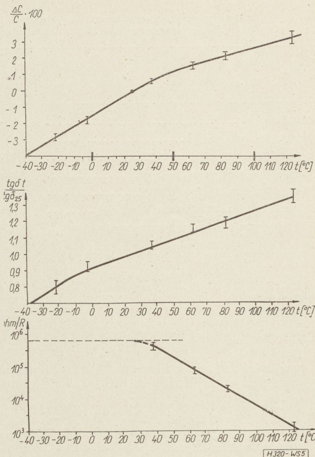
5. ábra. A kondenzátorok kapacitásának, veszteségi tényezőjének és szigetelési ellenállásának hőmérsékletfüggése
