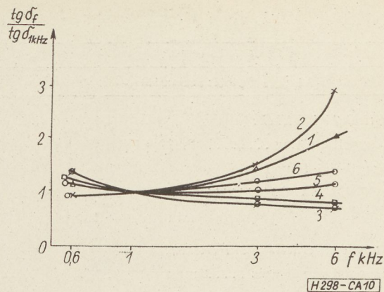
10. ábra. Gőzölt dielektrikumú kondenzátorok veszteségi tényezőjének frekvencia függése. 1–2–3 – SiO dielektrikumú kondenzátorok; 4–5–6 – MgF 2 dielektrikumú kondenzátorok
