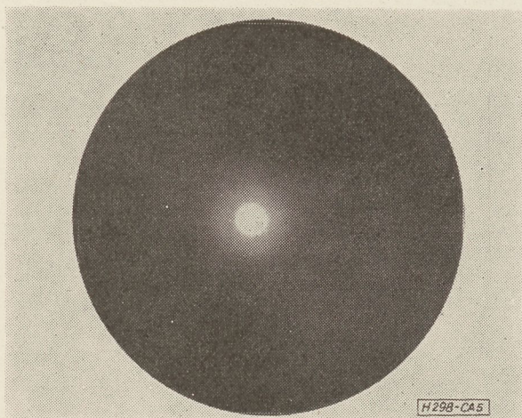
5. ábra. Párolgatott SiO réteg elektrondiffrakciós felvétele 1 óra 400 °C-os hőkezelés után
