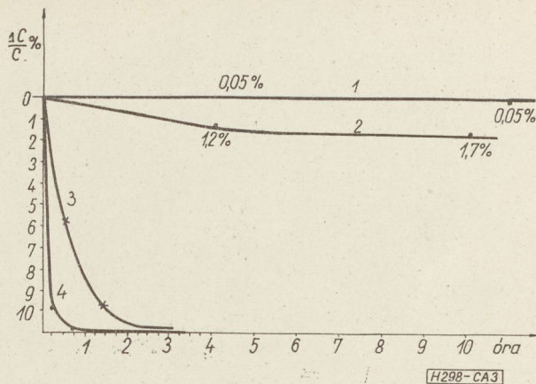
3. ábra. Százalékos kapacitás csökkenés a hőkezelési idő függvényében különböző hőkezelési hőfokokon \left(-\frac{\Delta C}{C}\right) \cdot 100 – 120 °C; 2 – 200 °C; 3 – 300 °C; 4 – 400 °C
