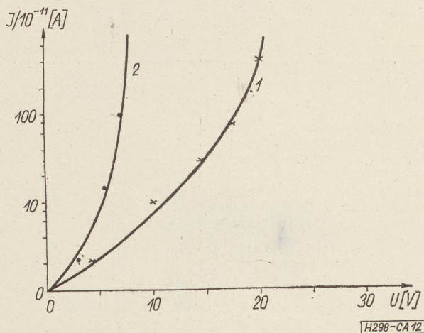
12. ábra Gőzölt dielektrikumú kondenzátorok áram-feszültség karakterisztikája. 1 – SiO dielektrikumú (1000 Å); 2 – MgF 2 dielektrikumú (1500 Å)
