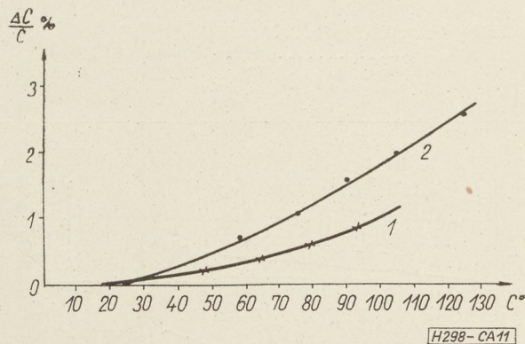
11. ábra. Gőzölt dielektrikumú kondenzátorok kapacitásának hőfokfüggése. 1 – SiO dielektrikumú kondenzátorok; 2 – MgF 2 dielektrikumú kondenzátorok
