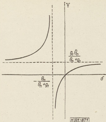
1. ábra. Az ideális klisztron-modulátor feltételezett terhelő áramkörének fáziskarakterisztikája
