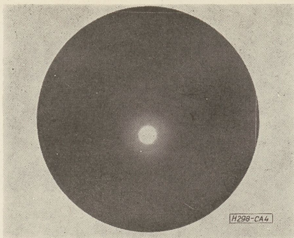
4. ábra. Párolgatott SiO réteg elektrondiffrakciós felvétele közvetlenül párolgatás után
