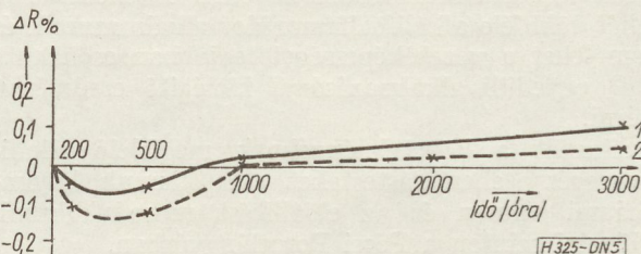
5. ábra. Az alkáliionszegény és közönséges porcelántestekre készült kristályosszén ellenállás váltóáramú terhelési stabilitása az idő függvényében (0,25 W, 1/400 KΩ). 1 — alkáliionszegény porcelán, 2 — közönséges porcelán
