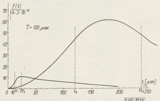
4. ábra. A (4) összefüggés ábrázolása. A kisebbik jelel a felfutási idő t_1 = 12 \mu s , míg a nagyobbik jelel t_2 = 120 \mu s . a) \tau = 6 \mu s ; b) \tau = 120 \mu s
