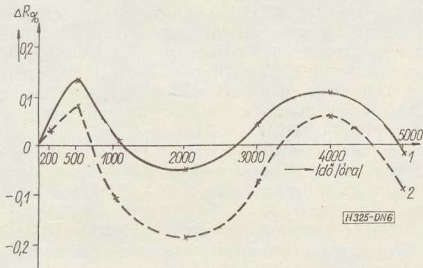
6. ábra. Alkáliionszegény és közönséges porcelántestekre készült kristályosszén ellenállás raktározási stabilitása az idő függvényében (0,25 W, 1/400 KΩ). 1 — alkáliionszegény porcelán, 2 — közönséges porcelán
