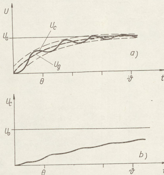
5. ábra. A generátorfeszültség exponenciális homlokú, 5a esetén \vartheta = 4\Theta , ( \Theta = 12,6 ), T = \Theta . 5b esetén: \vartheta = 4\Theta , ( Q = 12,6 ), T = \vartheta . Jelölések: \Theta a rezgőkör saját periódusideje, \vartheta a rezgőkör csillapítási időállandója, T a generátorfeszültség időállandója
