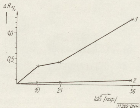
4. ábra. Alkáliionszegény és közönséges porcelántestekre készült kristályosszén ellenállás IEC szerinti nedves terhelési stabilitása. 1 — közönséges porcelán, 2 — alkáliionszegény porcelán
