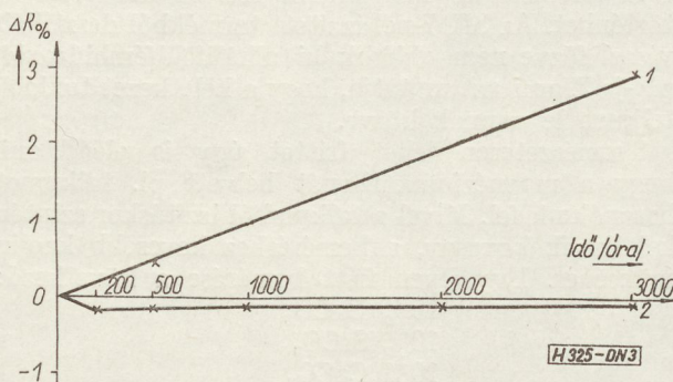
3. ábra. Az alkáliionszegény és közönséges porcelántestekre készült kristályosszén ellenállás (0,25 W, 1/4000 KΩ) egyenáramú terhelési stabilitása az idő függvényében. 1 közönséges porcelán, 2 alkáliionszegény porcelán
