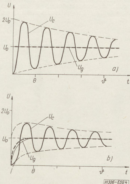
4. ábra. 4a esetén a generátorfeszültség ugrásfüggvény, \vartheta = 4\Theta ( Q = 12,6 ). 4b esetén a generátorfeszültség exponenciális homlokú, \vartheta = 4\Theta , ( Q = 2,6 ), T = 0,2 \Theta . Jelölések: \Theta a rezgőkör saját periódusideje, \vartheta a rezgőkör csillapítási időállandója, T a generátorfeszültség időállandója
