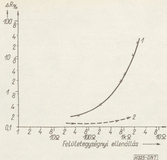
7. ábra. Alkáliionszegény és közönséges porcelántestekre készült kristályosszén ellenállás egyenáramú terhelési stabilitása ( \Delta R\% , 5000 óra) a felületegységnyi ellenállás függvényében. 1 — közönséges porcelán, 2 — alkáliionszegény porcelán
