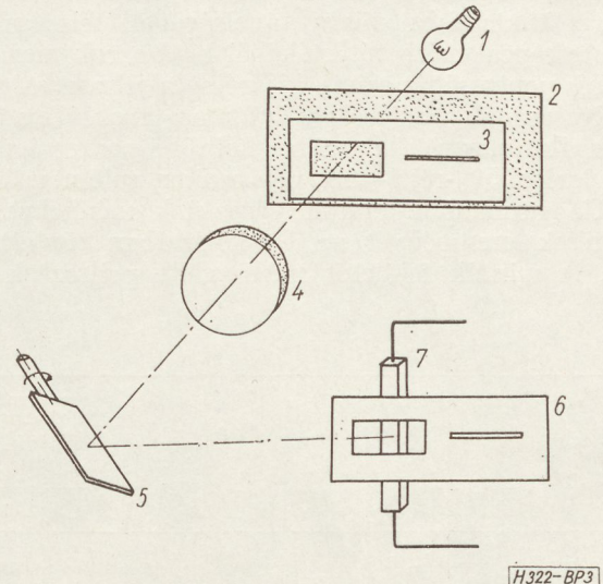
3. ábra. A mérés elrendezésének sematikus rajza. 1 — fényforrás, 2 — homályos üveg, 3 — tolóablak, 4 — optika, 5 — forgó tükör, 6 — tolóablak, 7 — fémvetet minta
