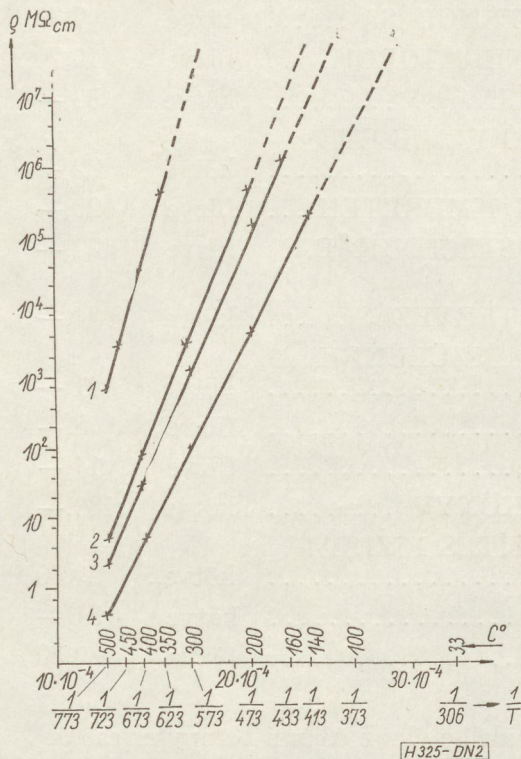
1. ábra. Különbő porcelánok fajlagos ellenállása, összehasonlítva a kvarcéval, a hőmérséklet függvényében. 1 kvarc-rúd, 2 stromciummentes alkáliionszegény porcelán, 3 alkáliionszegény porcelán, 4 közönséges porcelán
