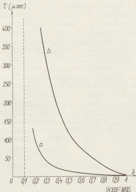
2. ábra. A mérés kiértékeléséhez szükséges grafikonok. a görbe: t_1 = 12 \mu s ; t_2 = 120 \mu s , b görbe: t_1 = 96 \mu s ; t_2 = 960 \mu s
