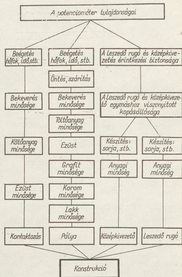
1. ábra. A potenciométer tulajdonságainak függése a konstrukciótól és a gyártástechnológiától
