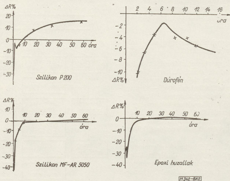
2. ábra. A terhelés hatására bekövetkező ellenállásváltozás a beégetési idő függvényében
