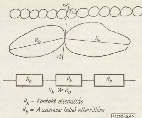
4. ábra. Koromszemcsék kontakt és „belső ellenállása”
