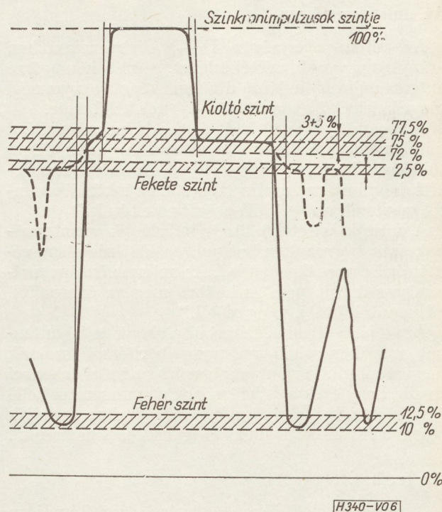
6. ábra. Képadó kimenő jelének térértékei
