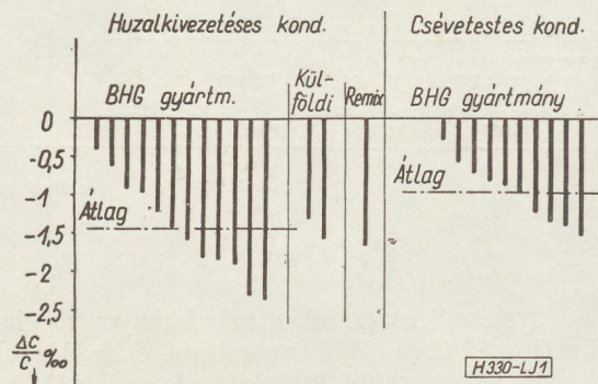
1. ábra. Három hőciklus utáni maradó kapacitásváltozás
