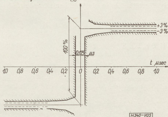
5. ábra. Térértékek a magasfrekvenciás (100–250 kHz) ismétlődési frekvenciájú négyszögimpulzus torzulásának kiértékeléséhez
