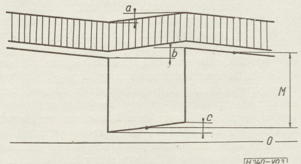
3. ábra. Torzított 50 Hz-es négyzetimpulzus vázlatos rajza a kiértékeléshez használt betűjelölésekkel
