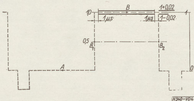
4. ábra. Térértékek a sorfrekvenciás ismétlődési frekvenciájú felsor időtartamú négyszögimpulzus torzulásának kiértékeléséhez
