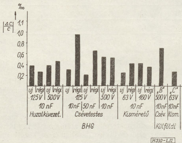
2. ábra. 1 éves tárolás alatt bekövetkező kapacitás változás
