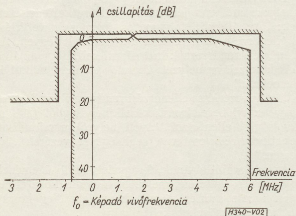
2. ábra. Képadó amplitúdó — frekvencia karakterisztikájának tűrései
