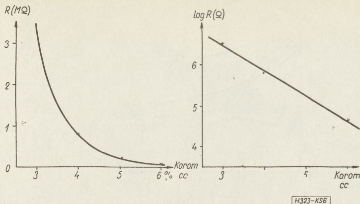
6. ábra. a) Az ellenállás alapérték és koromkoncentráció közötti összefüggés. b) Az ellenállás alapérték logaritmus és a koromkoncentráció közötti összefüggés előkezeletlen (A) és előkezelt (B) korom esetében
