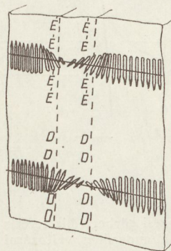
8. ábra. Mágneses nyomatékvektorok elrendeződése a doménfalban
