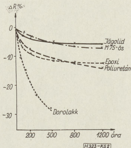
2. ábra. Különböző lakkokból készült ellenállások terhelési stabilitása
