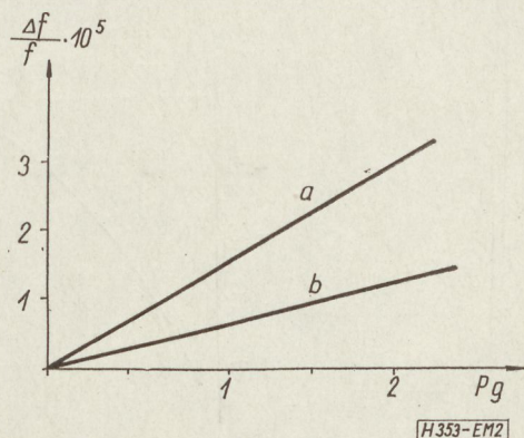
2. ábra. 4 KHz-es kristályok erő-frekvencia jelleggörbéje a) hosszirányú húzóerő, b) keresztirányú nyomóerő
