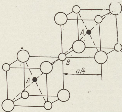
1. ábra. A szoros illeszkedésű köbös térrács elrendezése
