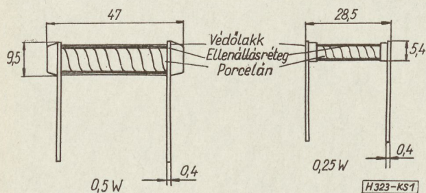
1. ábra. A nagy ohmértékű lakkrétegellenállások mérete és külalakjai
