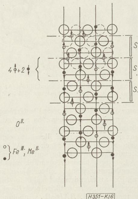
6. ábra. A köbös térrács (111) tengelyével párhuzamos metszet ion-elrendezése
