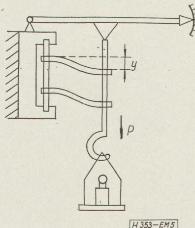
5. ábra. A foszforbronz tartóhuzalok rugalmasságának kimérése
