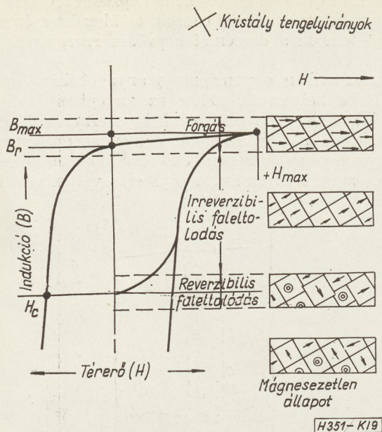
9. ábra. A mágnesezési görbe, a hiszterézis görbe és a domén-elrendeződés változásai
