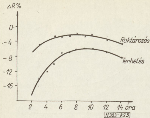
5. ábra. Epoxizsír-savészter lakkal készült ellenállások terhelési és raktározási stabilitása a beégetési idő függvényében
