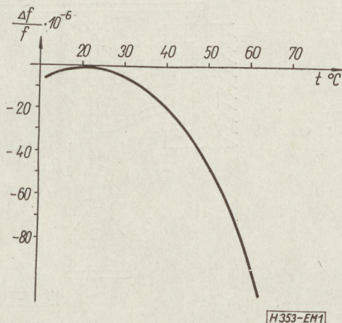
1. ábra. 4 KHz-es kristály hőfok-frekvencia jelleggörbéje kompenzálás nélkül
