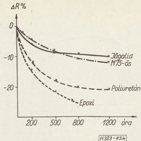
4. ábra. Különböző lakkokból készült ellenállások értékváltozása 100 °C-os tárolás alatt
