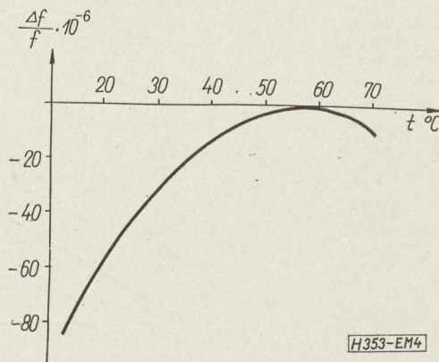
4. ábra. 4 KHz-es horgany állvánnyal kompenzált kristály hőfok-frekvencia jelleggörbéje
