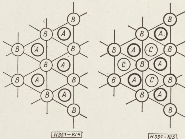
4. ábra. A hexagonális térrácsréteg elrendezése
