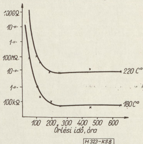
8. ábra. Azonos koromkoncentrációjú lakkrétegek ellenállásváltozása az ellenállásmassza golyósmalmozási idejének függvényében 180^\circ\text{C} -on és 220^\circ\text{C} -on előkezelt koromok esetén
