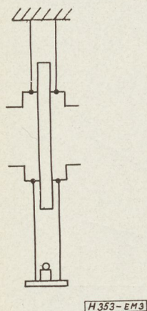
3. ábra. A hosszirányú húzóerő hatásának kimérése
