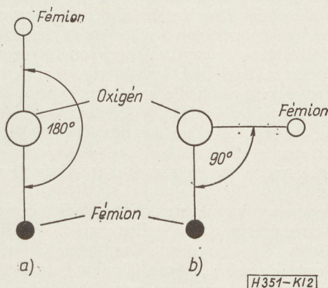
2. ábra. A közvetett kölcsönhatás vázlata
