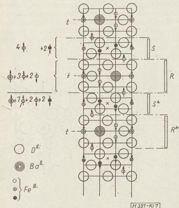
7. ábra. A báriumferrit kristály szerkezetének ion-elrendezése
