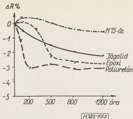
3. ábra. Különböző lakkokból készült ellenállások raktározási stabilitása
