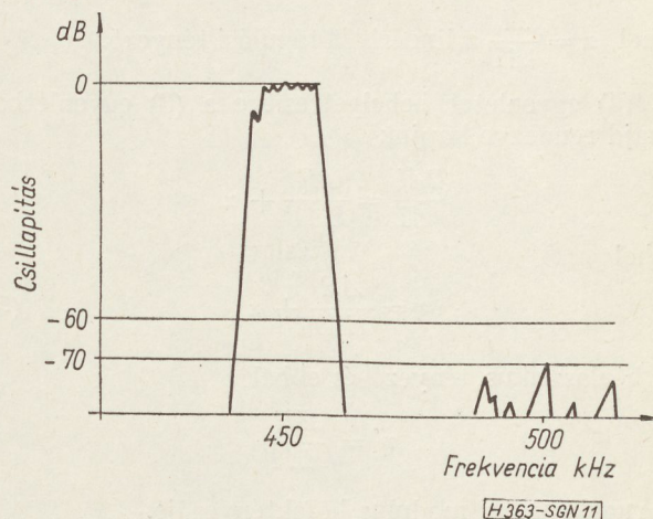
11. ábra. Mechanikus szűrő átviteli karakterisztikája és parazita frekvenciák
