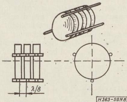
8. ábra. Tárcsarezonátorokból felépített huzalcsatolású szűrőtest
