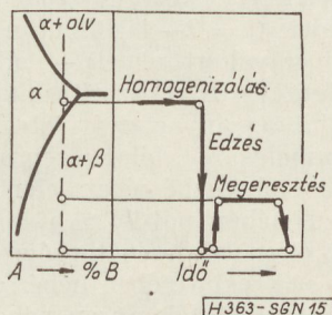
15. ábra. Szegregációs nemesítés hőmérséklet-idő diagramja (Verő)
