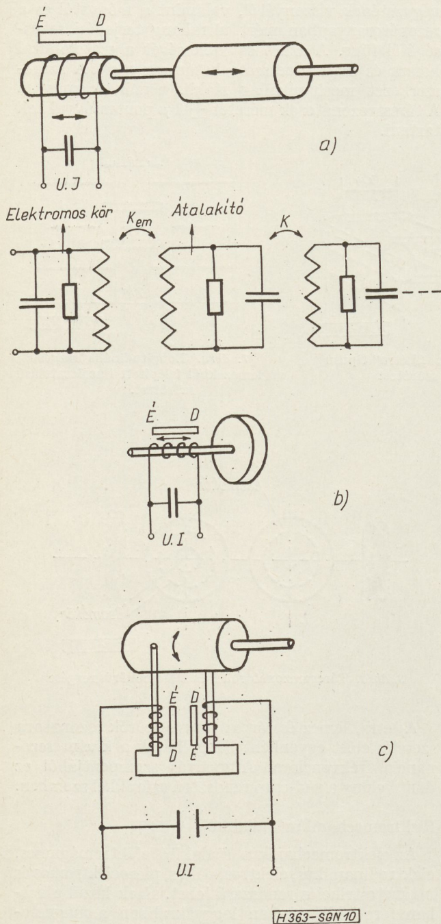
10. ábra. Különböző magnetostrikciós átalakítók a) longitudinálisan rezgő rezonátor meghajtása magnetostrikciós ferrittel b) tárcsarezonátor meghajtása magnetostrikciós fémhuzallal c) torziósan rezgő fémrezonátor meghajtása magnetostrikciós fémhuzallal
