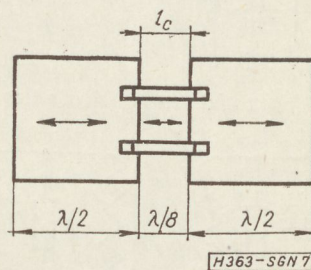
7. ábra. Longitudinális rezgésű lemezekből felépített huzalcsatolású szűrőtest.
