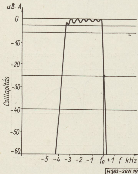
19. ábra. Egyoldalsávú alkalmazási célra előállított mechanikus szűrő átviteli karakterisztikája
