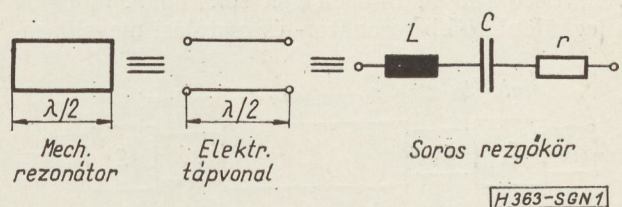
1. ábra. Félhullámhosszúságú mechanikus rezonátor elektromos megfelelői
