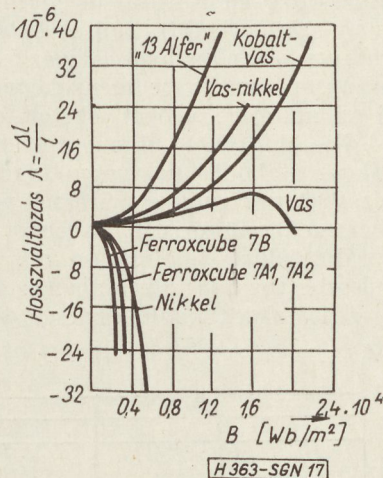
17. ábra. Különböző anyagok magnetostrikciója (Burgt)
