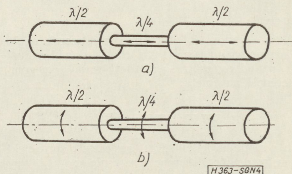
4. ábra. Rúdrezonátoros csapcsatolású mechanikus szűrőtest a) longitudinálisan rezgő, b) torziósan rezgő
