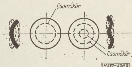
9. ábra. Tárcsarezonátorok 1 és 2 csomókörös rezgése
