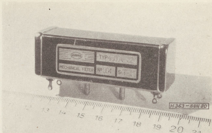
20. ábra. Gamma Műveknél egyoldalsávú alkalmazási célra előállított mechanikus szűrő
