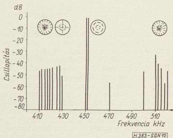
12. ábra. Tárcsarezonátor különböző módusú rezonáns frekvenciái
