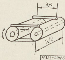
6. ábra. „Létra” típusú szűrőtest
