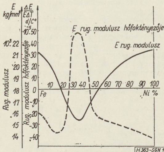
13. ábra. Az E rugalmassági modulusz és hőfoktényezőjének változása Fe-Ni ötvözetnél a Ni tartalom függvényében (Guillaume)
