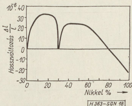
18. ábra. Fe-Ni ötvözetek magnetostrikciója a Ni tartalom változásával (Bozorth)
