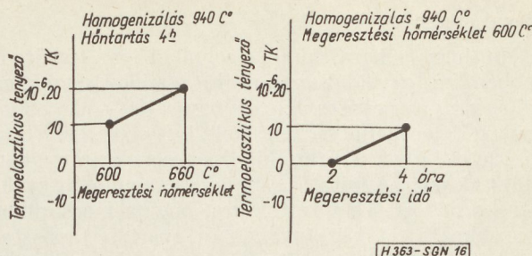
16. ábra. A megeresztési hőmérséklet és idő befolyása adott összetételű Ni-Span C anyag hőfoktényezőjére [24]
