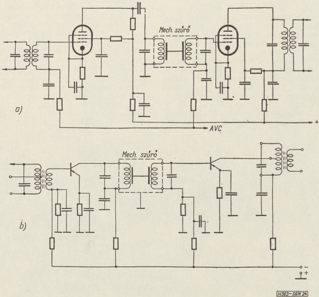
24. ábra. Mechanikus szűrők alkalmazása elektroncsöves és tranzisztoros KF fokozatokban
