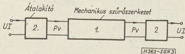
3. ábra. Mechanikus szűrő blokkismája
