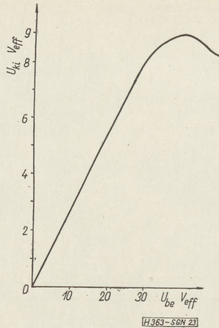
23. ábra. Mechanikus szűrő U_{be}U_{ki} karakterisztikája
