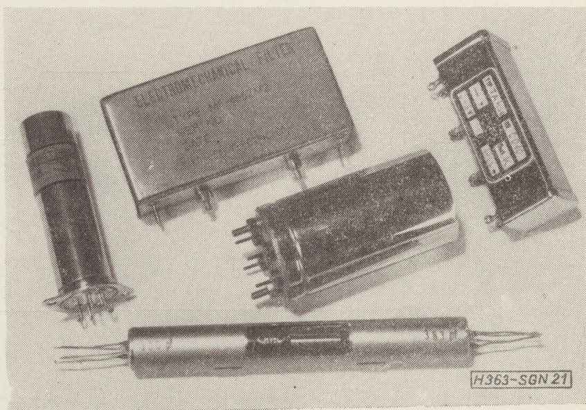
21. ábra. Különböző külföldi és Gamma gyártású mechanikus szűrők
