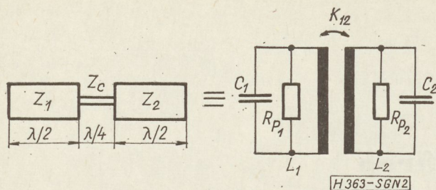
2. ábra. Mechanikus csatolt kör elektromos megfelelője
