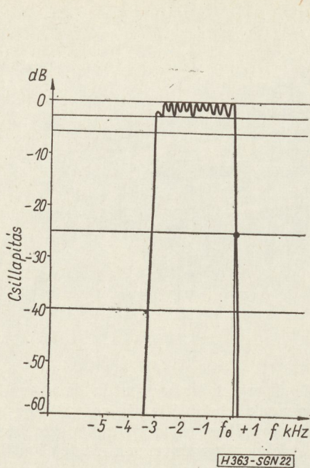
22. ábra. 12 rezonátoros mechanikus szűrő karakterisztikája
