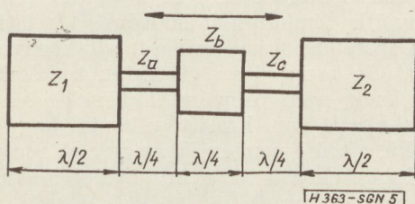
5. ábra. Rúdrezonátoros \frac{3}{4} \lambda hosszúságú csatolócsapos szűrőtest
