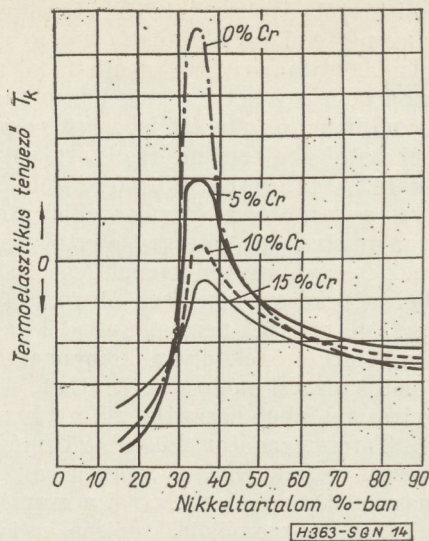
14. ábra. Az E rugalmassági modulusz hőfoktényezőjének változása Fe-Ni ötvözetnél a Cr tartalomtól függően (P. Chevenard)
