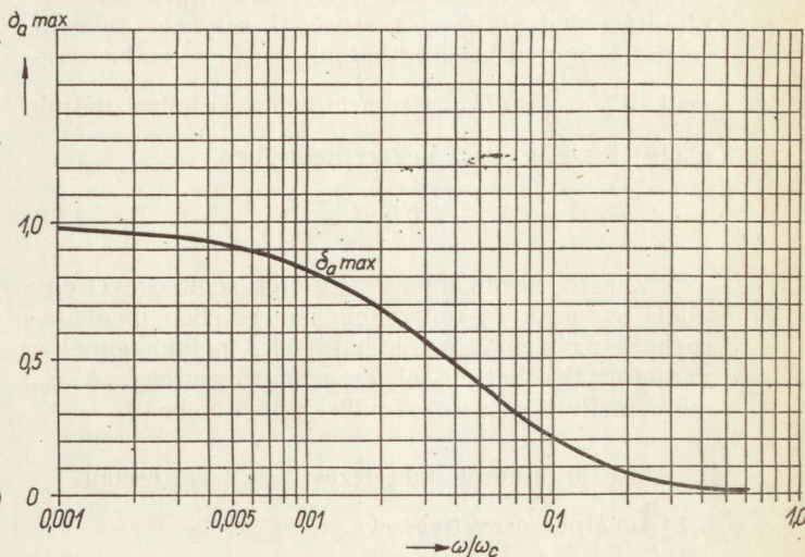
7. ábra. Frekvenciaduplázó maximális átalakítás hatásfoka függvényben az \frac{\omega}{\omega_c}
