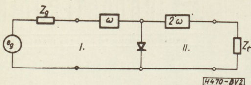
2. ábra. Frekvenciaduplázó áramkör ekvivalens kapcsolása
