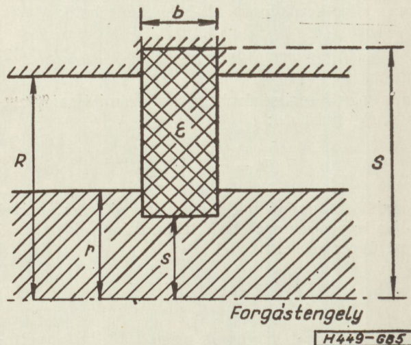
5. ábra. Kitámasztó koaxiális vezetékben
