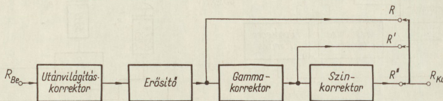
3. ábra. A fő erősítő egy csatornájának (R) elvi felépítése
