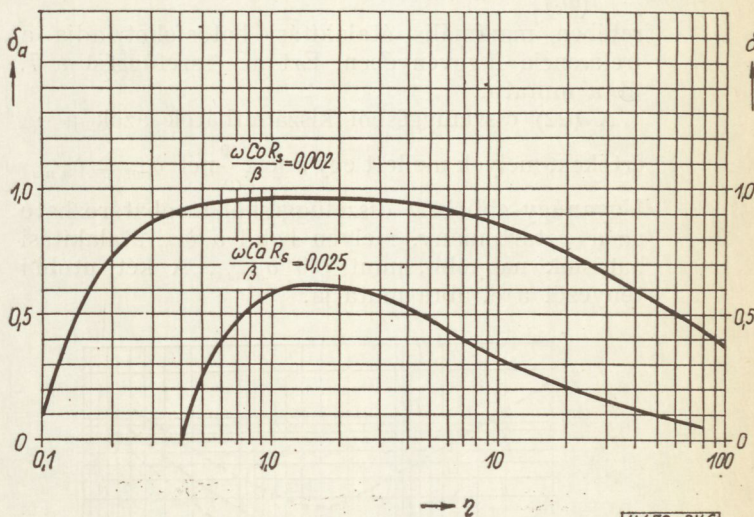
6. ábra. Frekvenciaduplázó átalakítás hatásfoka az \eta áramtényező függvényében két különböző \frac{\omega C_0 R_s}{\beta} paraméter esetén
