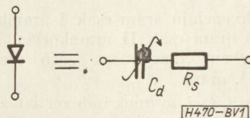
1. ábra. Varactort helyettesítő soros ekvivalens kapcsolás
