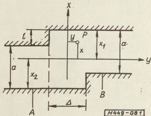
1. ábra. Ugráshely sík vezetékben
