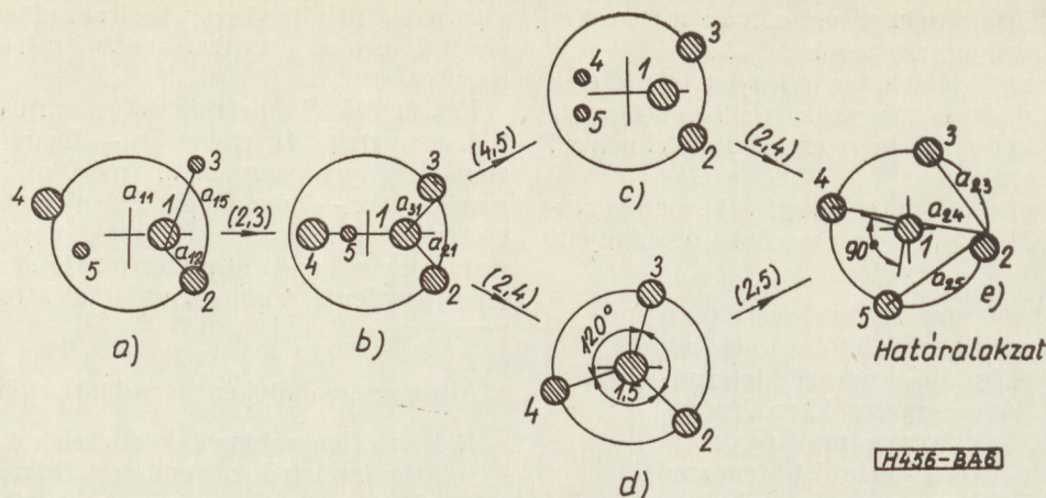
6. ábra. Az ábra a szimmetriafeltételek geometriai jelentésének és a redukció végrehajtásával kapcsolatos geometriai tevékenység szemléltetése. Az ábrák az elektródarendszer w síkú képei. A rajzok léptéke olyan, hogy a bejelölt távolságok a_{xy} -nal egyenlők és az anódhenger a centrumtól távol van.
