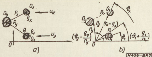
3. ábra. a) P -k optimális hálózata D_{JK}^Y számításához. b) Az optimális hálózat megközelítése, P_x = P_1 -et r_1 sugarú kör és q_1 kerület P_x = P_x - t r_x sugarú és q_x kerület metszéspontjával határozzuk meg
