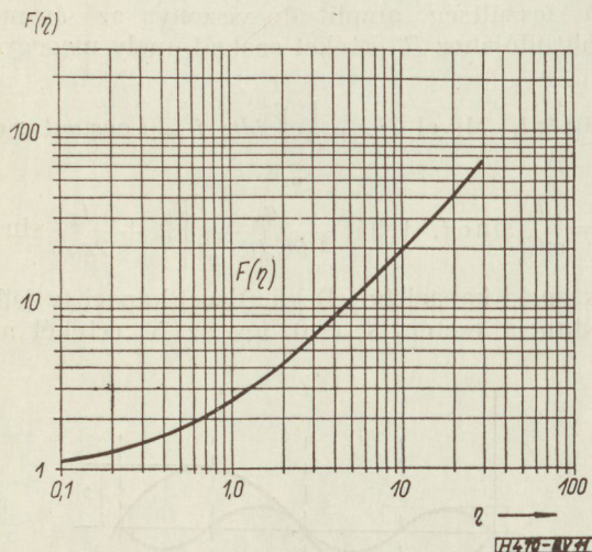
11. ábra. F(\eta) -függvény
