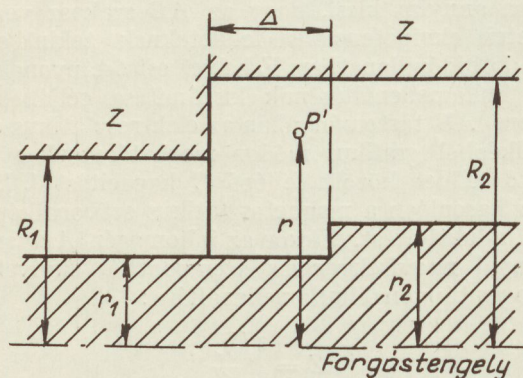
2. ábra. Ugráshely koaxiális vezetékben
