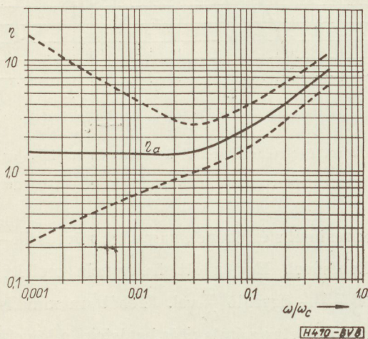
8. ábra. Maximális átalakítás hatásfokához tartozó \eta_a áramtényező \frac{\omega}{\omega_c} függvényében
