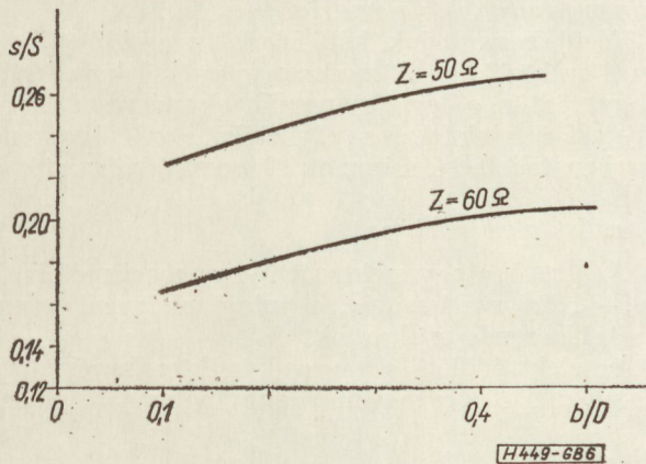
6. ábra. Reflexiómentes teflon kitámasztóra vonatkozó görbék. Az 50 ohmos görbe számítással adódott a 60 ohmosból
