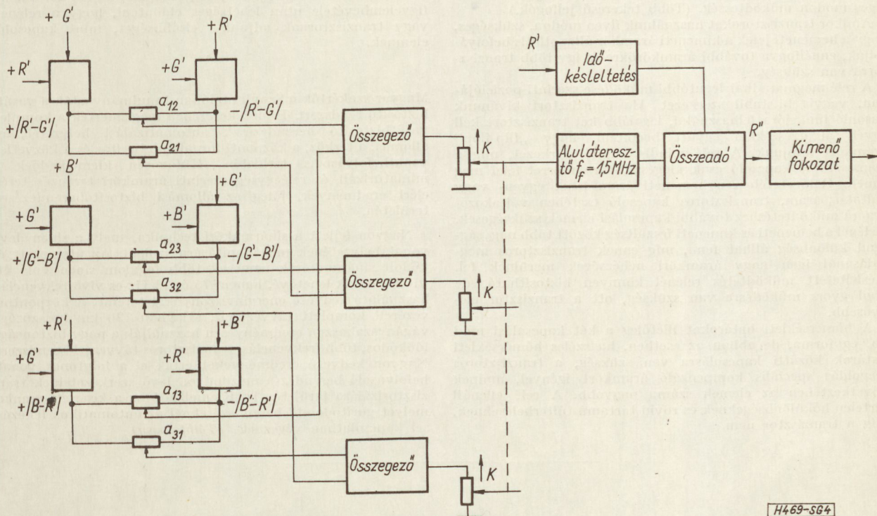
4. ábra. Színekorrektor elvi felépítése (A legsó G' helyesen B' )
