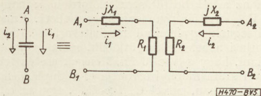
5. ábra. Ideális varactor ekvivalens kapcsolása abban az esetben, amikor varactoron keresztül csak \omega és 2\omega frekvenciájú áramok folynak
