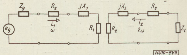
9. ábra. Frekvenciaduplázó teljes helyettesítési rajza
