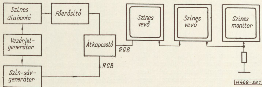
1. ábra. A bemutató elvi elrendezése
