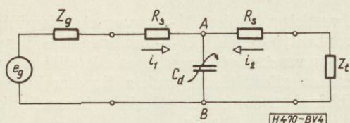
4. ábra. Frekvenciaduplázó áramkör ekvivalens kapcsolása
