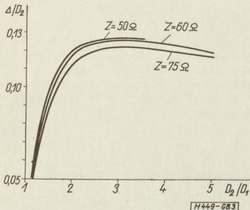
3. ábra. Reflexiómentes ugrásra vonatkozó görbék. Az 50 és 75 ohmos görbe számításával adódott a 60 ohmos görbéből
