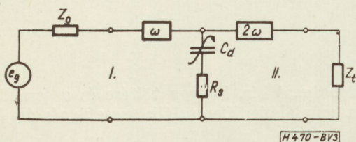
3. ábra. Frekvenciaduplázó áramkör ekvivalens kapcsolása
