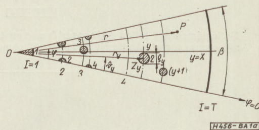
1a ábra. A vonatkoztatási rendszer. P = P(r, \varphi) a szektor egy pontja. z_y az y -ik bot tengelyének helyvektora. Feltüntettük a bevezetett indexeket és az elektródák leszámolását
