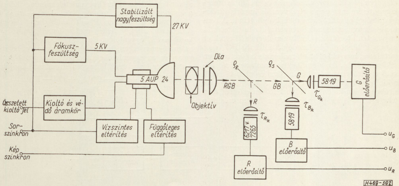
2. ábra. Színes dia-bontó elvi felépítése
