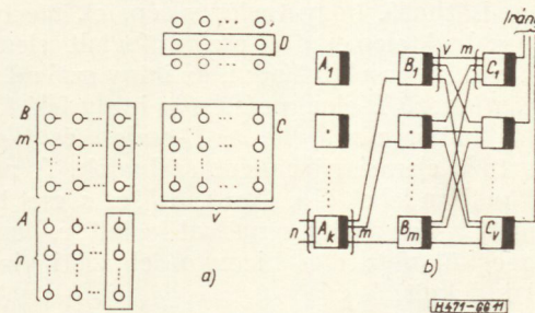
11. ábra. Egyszerű háromfokozatú csatolóutas rendszer
