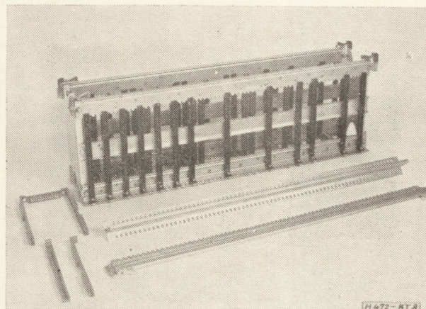
8. ábra. Szekrényfiók a középső pótmerevítéssel
