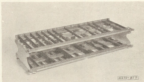
7. ábra. Választó sínek szekrényen kívüli összeszerelése
