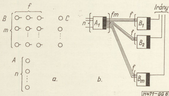
8. ábra. Nem teljes csatolóutas rendszer, f < 1
