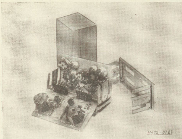
2. ábra. „B” jelű nyomtatott áramköri lap elhelyezésének példája
