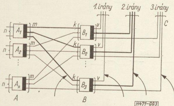
3. ábra. Kétfokozatú csatolóútas rendszer keresztrudas kapcsológépekkel
