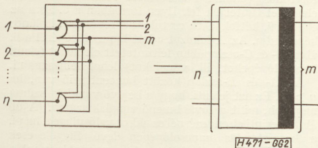
2. ábra. Keresztrudas kapcsológép ábrázolása
