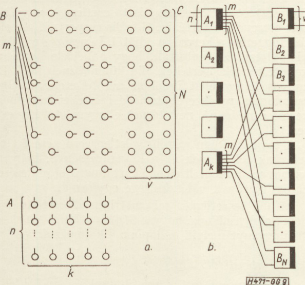
9. ábra. Lépcsőzött csatolóutas rendszer
