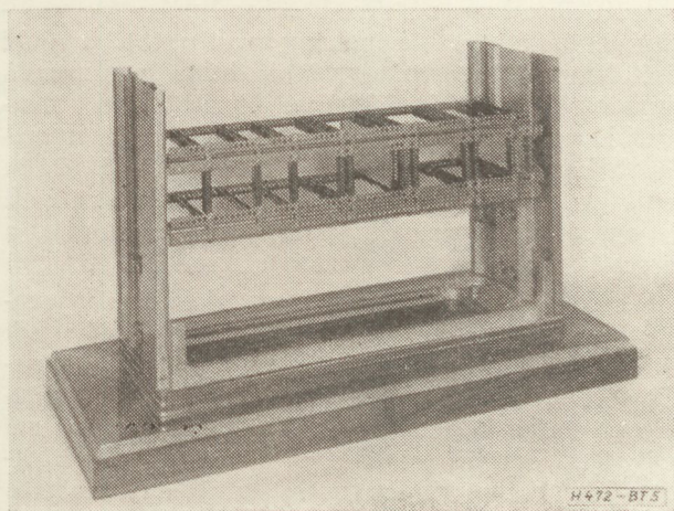
5. ábra. Szekrény-keresztmetszet hátulnézetben az alumínium öntvényekkel
