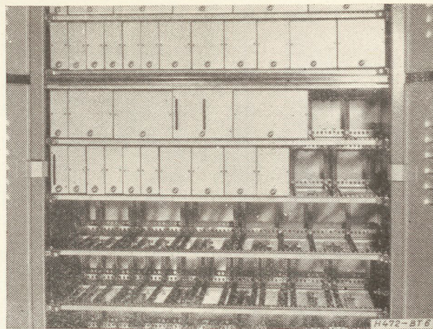
6. ábra. Szekrény részlet a különböző méretű egységekkel
