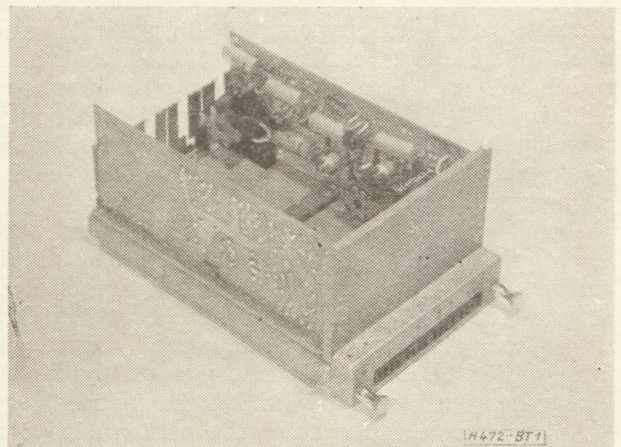
1. ábra. „A” jelű nyomtatott áramköri lapok elhelyezésének példája
