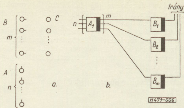
6. ábra. Egyszerű kétfokozatú csatolóútas rendszer
