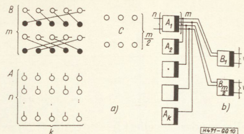
10. ábra. Belsőleg lépcsőzött csatolóutas rendszer
