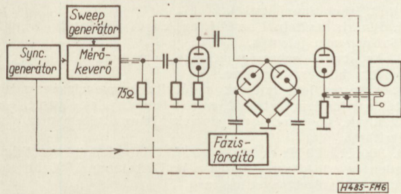
6. ábra. Vezérelt szinthehelyreállító kapcsolással ellátott erősítő-fokozat szórt kapacitásának mérési elve
