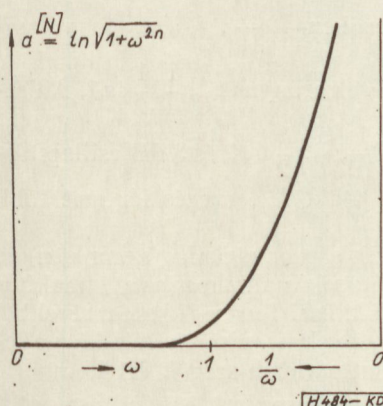
1. ábra. Maximális laposságú vagy Butterworth típusú közelítés
