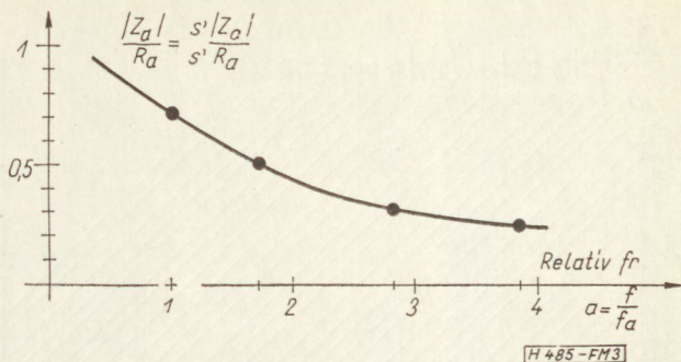
3. ábra. Párhuzamosan csatolt RC tag impedanciájának abszolút értéke a relatív frekvencia függvényében
