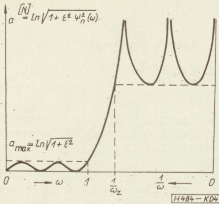
4. ábra. Elliptikus vagy Cauer közelítés ( \psi \dots az n -ed rendű elliptikus függvény)
