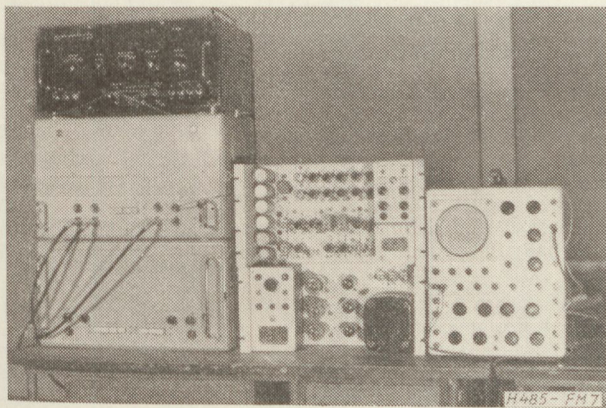
7. ábra. Vezérelt szinthehelyreállító kapcsolással ellátott erősítő fokozat mérési összeállítása
