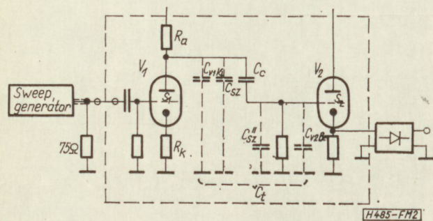
2. ábra. Szórt kapacitások mérése sweep-generátorral A mérés elve
