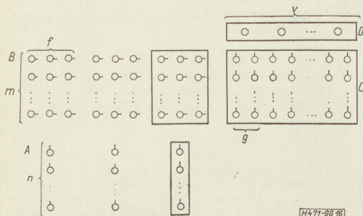
16. ábra. Háromfokozatú nem teljes csatolótás rendszer
