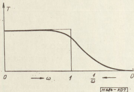
7. ábra. Maximális laposságú futási idő karakterisztika
