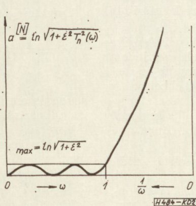
2. ábra. Egyenletes vagy Csebisev közelítés ( T_n ... az n -edfokú Csebisev polinom)
