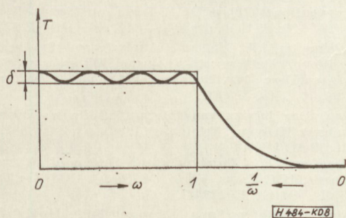
8. ábra. Csebishev típusú futási idő karakterisztika
