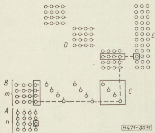
17. ábra. Négyfokozatú csatolótás rendszer (egyéni kereséssel)
