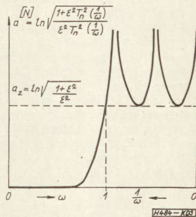
3. ábra. Inverz Csebisev közelítés
