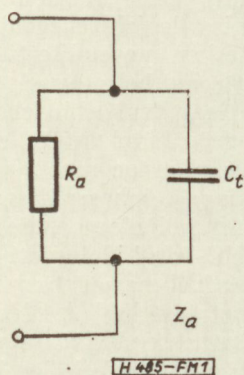
1. ábra. Szélessávú erősítők anódimpedanciája kompenzálás nélkül
