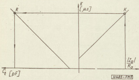
5. ábra. A szórt kapacitás meghatározására szolgáló nomogram használata
