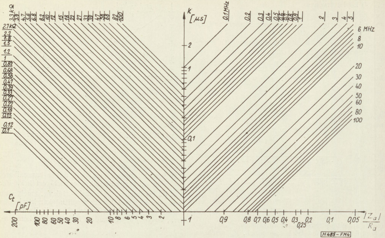
4. ábra. Szórt kapacitások meghatározására szolgáló nomogram
