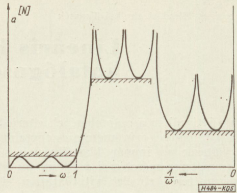
5. ábra. Általános szűrő-karakterisztika approximációja
