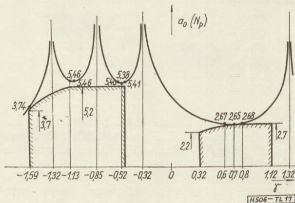
17. ábra. Póluselrendezés a \gamma -síkon (2. példa)
