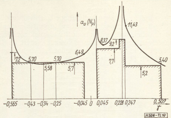
10. ábra. Póluselrendezés a \gamma -síkon (1. példa)
