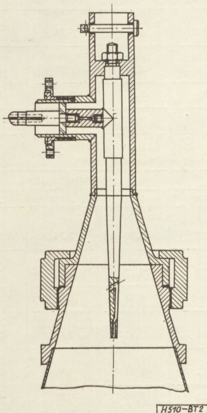
2. ábra. A gerjesztő tölcser keresztmetszete
