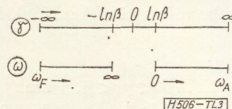
3. ábra. Sávszűrő \gamma -transzformáció
