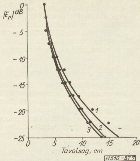
7. ábra. A sugárirányú elektromos térerősség-összetevő eloszlása 2000 MHz (1), 3000 MHz (2) és 3670 MHz (3) frekvencián, zománcszigetelésű rézhuzalos felületi hullámvezető esetén
