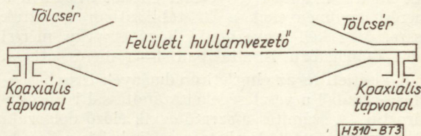
3. ábra. Felületi hullámú tápvonal
