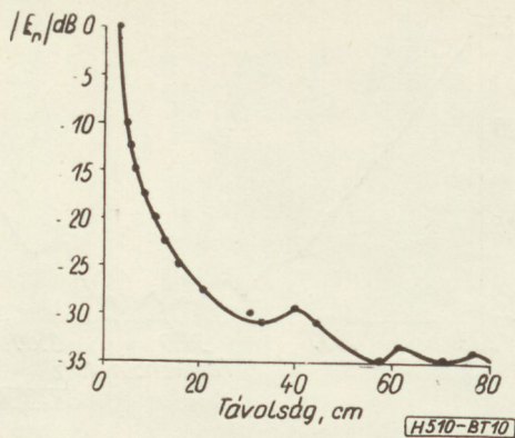
10. ábra. A sugárirányú elektromos térerősség-összetevő változása a huzaltól való távolság függvényében csupasz rézhuzalos felületi hullámvezető esetén
