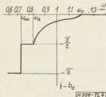
4. ábra. Ia típusú L-tag hullámforgatása
