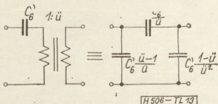
13. ábra. Kapacitív transzformáció
