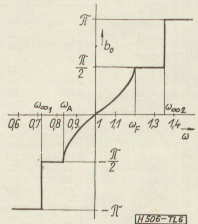
6. ábra. II. típusú L-tag ( m_1 = m_2^{-1} ) hullámforgatása
