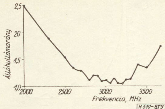
9. ábra. Csupasz rézhuzalos tápvonal állóhullámaránya a frekvencia függvényében
