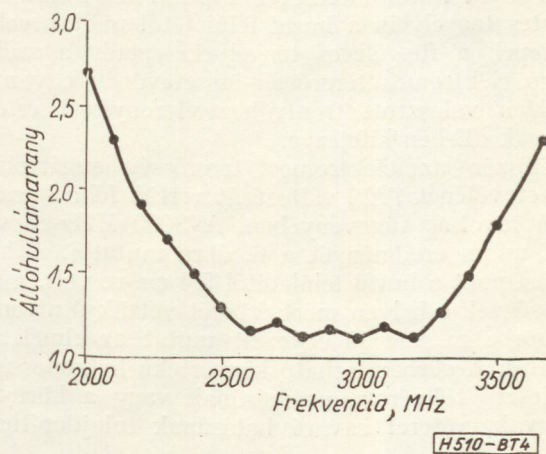
4. ábra. A kis tölcserrel gerjesztett hosszú zománcszigetelésű rézhuzaos tápvonal állóhullámaránya
