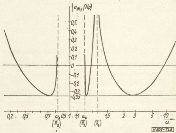
8. ábra. Primer ütközési csillapítás 5 típusú hullámimpedancia esetén
