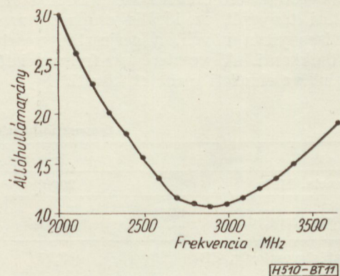
11. ábra. Polietilén-bevonatú rézsodrony tápvonal állóhullámaránya a frekvencia függvényében
