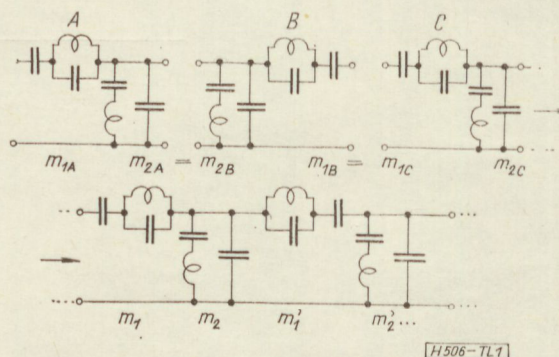
1. ábra. Cikkcakk szűrőláncalkotás
