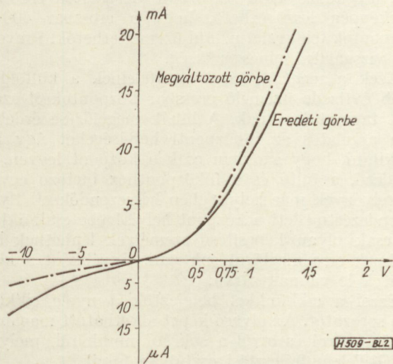
2. ábra. A 24. sz. OA 1154 Q dióda karakterisztikájának időbeli változása
