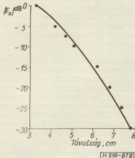
8. ábra. A tengelyirányú elektromos térerősség-összetevő csökkenése sugárirányban zománcszigetelésű rézhuzalos felületi hullámvezető esetén
