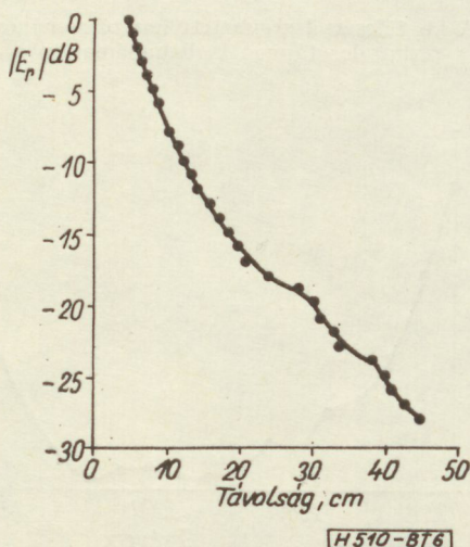
6. ábra. A sugárirányú elektromos térerősség-összetevő változása a huzaltól való távolság függvényében zománcszigetelésű rézhuzalos felületi hullámvezető esetén
