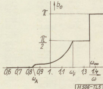
5. ábra. Ib típusú L-tag hullámforgatása
