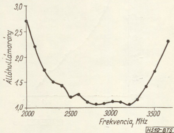
5. ábra. A nagy tölcserrel gerjesztett hosszú zománcszigetelésű rézhuzaos tápvonal állóhullámaránya
