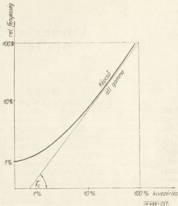
7. ábra. Tipikus képcső gamma-görbe
