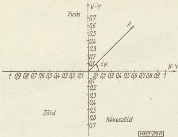
11. ábra. Az NTSC-re jellemző segédvívó fázis és amplitúdó moduláció
