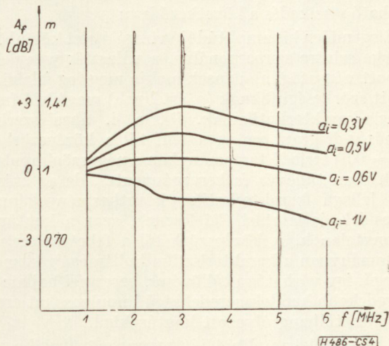
4. ábra. Dinamikus nonlinearitás görbék
