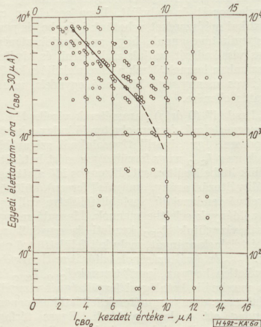
6a ábra. Összefüggés IC_{BO} kezdeti értéke és az IC_{BO} > 30 \mu A élettartam-véggponttal definiált egyedi élettartam közt, kisteljesítményű ötvözött germánium pnp tranzisztor-nál (600 darabból 8000 óra alatt). A korreláció nagyon laza. A berajzolt vonal az egyes időpontokhoz tartozó kiesések IC_{BO_0} értékeiből alkotott mediánok durva összekötéséből származik. Az IC_{BO} kezdeti értéke és az élettartam közt nem szabad egyértelmű összefüggést feltételezni
