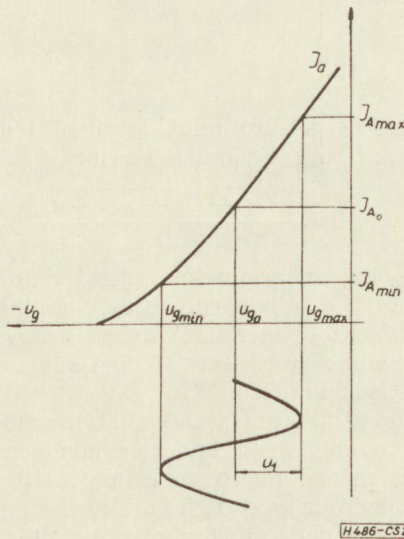
2. ábra. Torzítások másodfokú karakterisztika esetén
