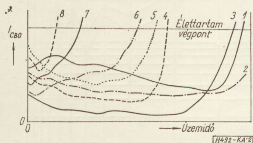
2. ábra. Erősen heterogén minőségű egyedek IC_{BO} időfüggvénye, elektromos tartóterhelés esetén ( Ge pnp ötvöztött tranzistoroknál). 1, 2, 3, : hosszú; 4, 5, 6, közepes; 7, 8 nagyon rövid élettartam. 1, 6: lassú; 2, 3, 4, 5 gyors „bestabilizálódás” \mu A . A vonalkázott területnek megfelelő példányok estek ki. Megfigyelhető, hogy a magas IC_{BO} -jú példányok közül relatíve magasabb a kiesés, de a különbség nem pregnáns. A IC_{BO} kezdeti értéke és a megbízhatóság közt szoros összefüggés tehát nincs; az alacsonyabb kezdeti IC_{BO} érték egy szükséges, de nem elégséges feltétele a fokozott megbízhatóságnak
