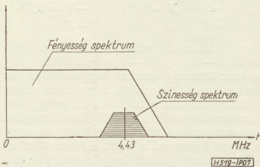
7. ábra. Összetett színes televíziójel videospektruma
