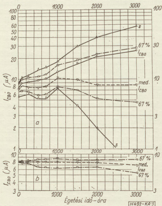
5. ábra. A „válogatási” eljárás eredményének illusztrációja 400 db kisteljesítményű ötvözött germánium pnp tranzisztor-nál (standard, szórakoztató ipari minőség)
