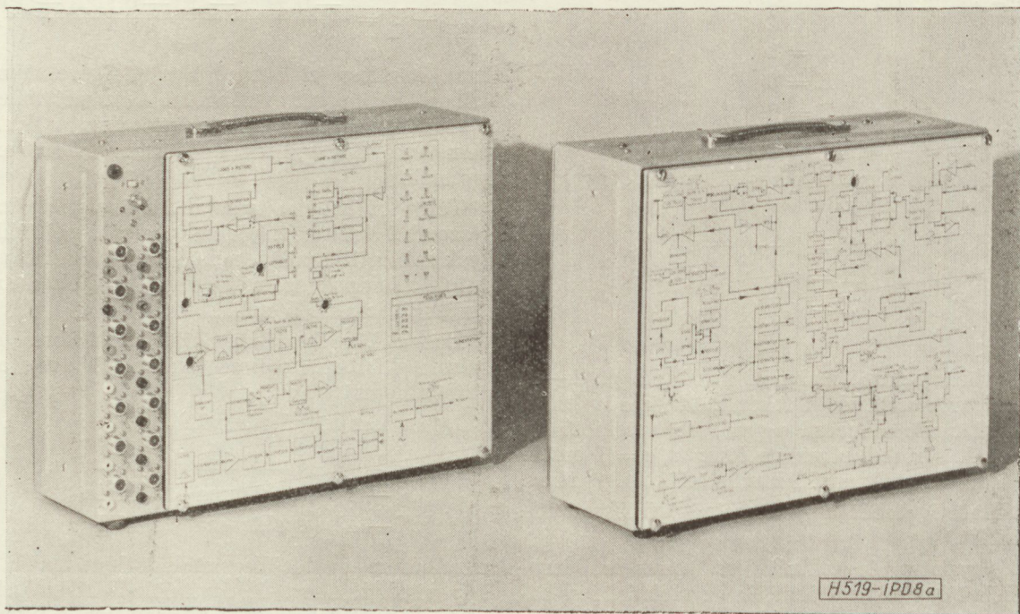
8a ábra. Secam kódoló elől — hátulnézet
