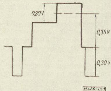
5. ábra. A kis ugrás jelalakja
