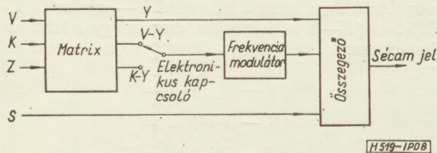
8. ábra. Secam típusú kódoló
