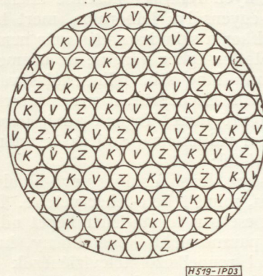
3. ábra. Katódsugárcső mozaikja. Képernyő előlnézete
