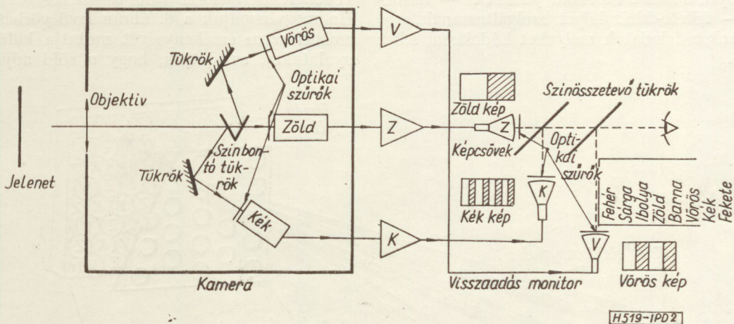
2. ábra. Háromcsatornás átvitel
