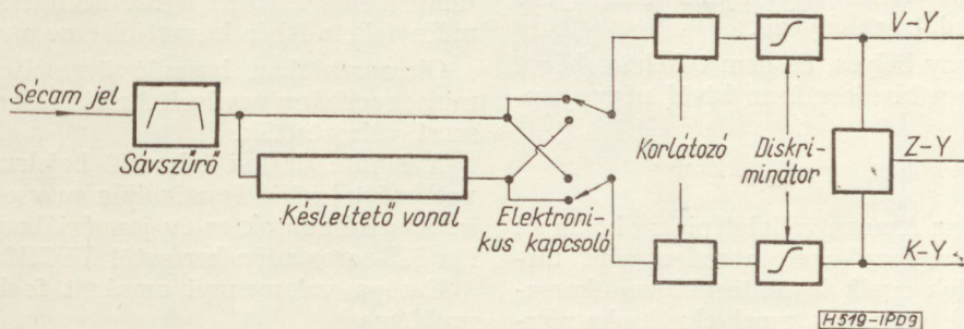
9. ábra. Dekódoló tömbvázlata
