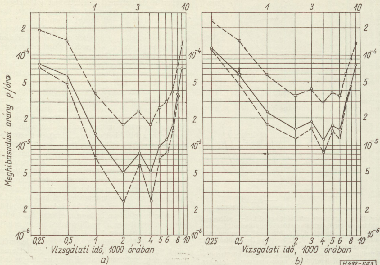
3. ábra. A hibásodási faktor időfüggése 600 db standarú minőségű kisteljesítményű ötvözött germánium pnp tranzistor statikus tartóségetésénél
