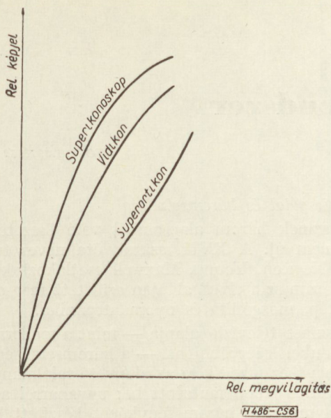
6. ábra. A képfelvevőcsövek gamma értékei
