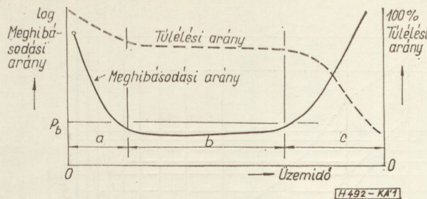
1. ábra. A meghibásodási arány (folytonos vonal) és a túlélési arányának (szaggatott vonal) időfüggvénye kellően homogén minőségű, elhasználódást mutató termék esetén
