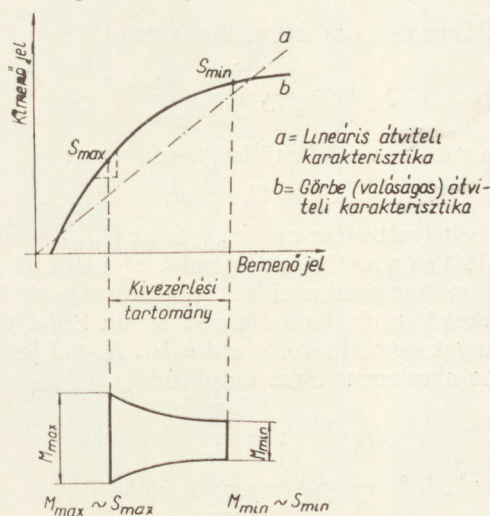
1. ábra. A nonlinearitás definíciója
