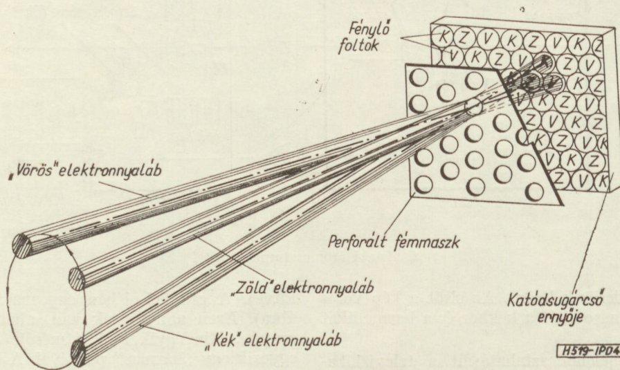
4. ábra. Perforált fémmaszkos cső működési elve
