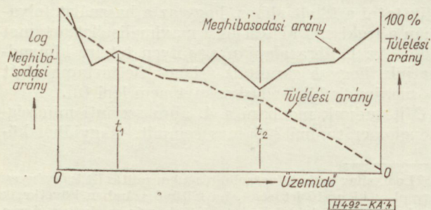
4. ábra. Heterogén minőségű termék meghibásodási arányának (folytonos vonal) és túlélési arányának (szaggatott vonal) időfüggvénye
