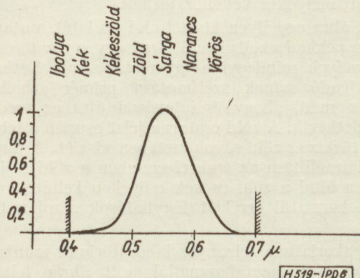
6. ábra. A szem érzékenysége
