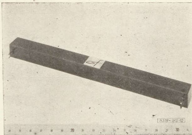
10. ábra. Késleltető művonal
