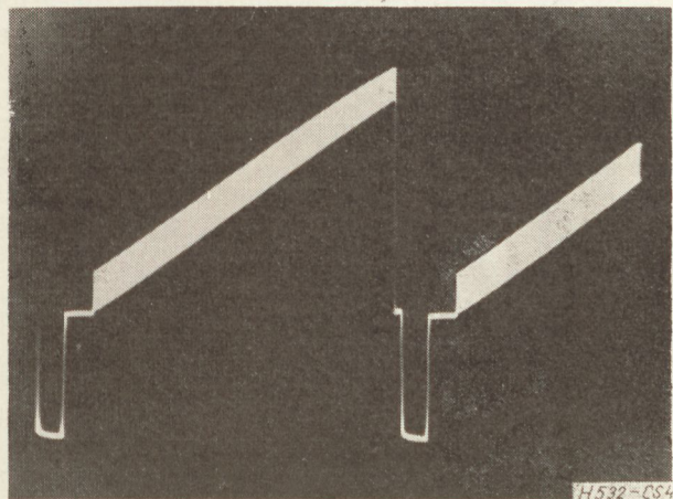
4. ábra. Solfrekvenciás fűrészel, szuperponált nagyfrekvenciával
