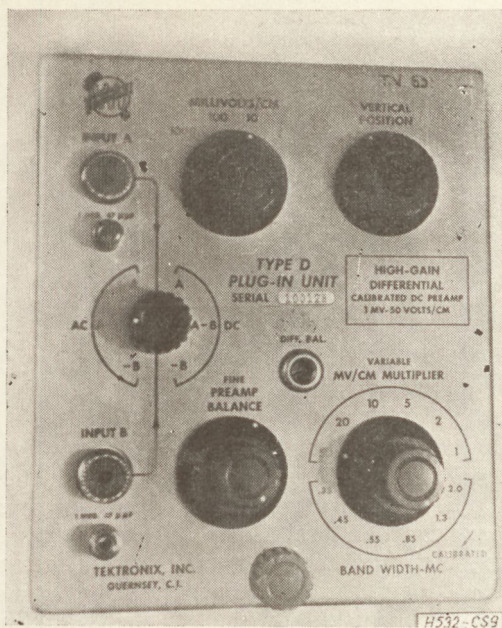
9. ábra. Differenciál erősítő
