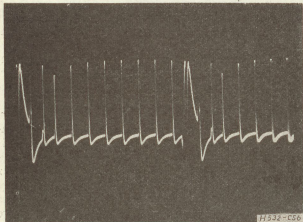
6. ábra. Lépcsőjelet linearitás-szűrő után
