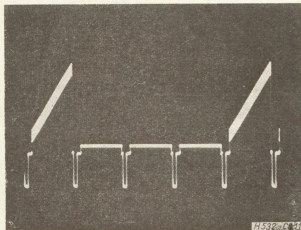
11. ábra. Sorfrekvenciás fűrészjel, változó egyenáramú középértékkel (fűrészjelek közt fekete sorok)
