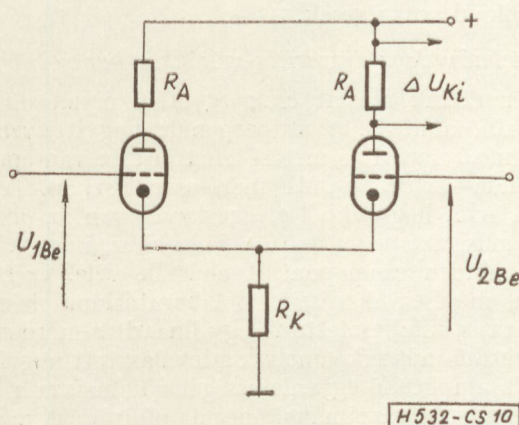
10. ábra. Differenciál erősítő alapkapcsolása
