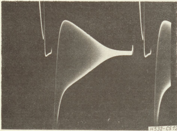
12. ábra. Határolt jel leválasztott nagyfrekvenciás jele
