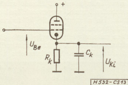
13. ábra. Katódkövető kapcsolás
