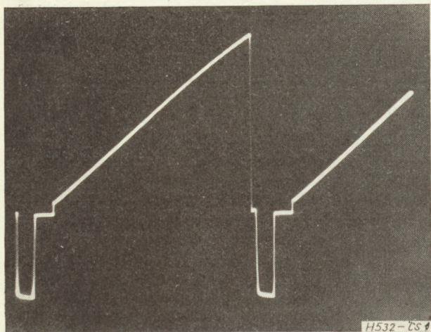
1. ábra. Sorfrekvenciás fűrészellet
