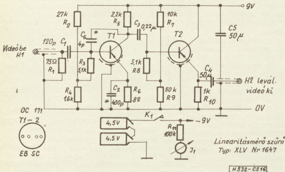
16. ábra. Az EMV XLV típusú linearitás-szűrő kapcsolási rajza
