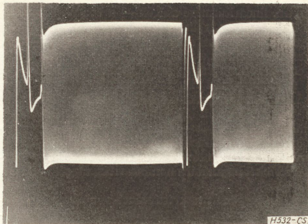
5. ábra. Leválasztott nagyfrekvencia (vízszintes eltérítés: solfrequentia)
