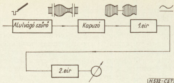
7. ábra. Közvetlenül mutató linearitás-mérő vázlata
