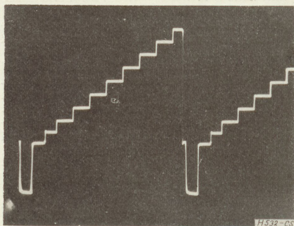
3. ábra. Sorfrekvenciás lépcsőjel
