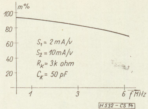
14. ábra. A katódkövető frekvencia függősége
