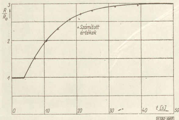
9. ábra. A termisztor ellenállása az idő függvényében a fűtés megszűntetése után
