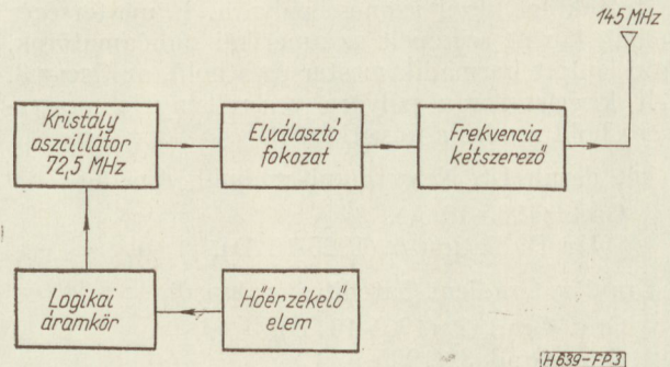
3. ábra. Az Oscar 1 és 2 elvi felépítése
