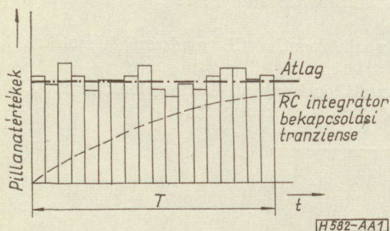
1. ábra. A mintavételi elv alkalmazása sávkorlátozott zaj mérésére
