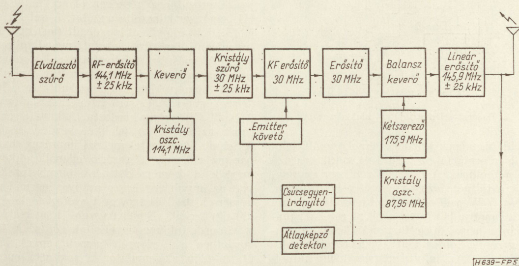
5. ábra. Az Oscar 3 hírátviteli rendszerének blokkdiagramja
