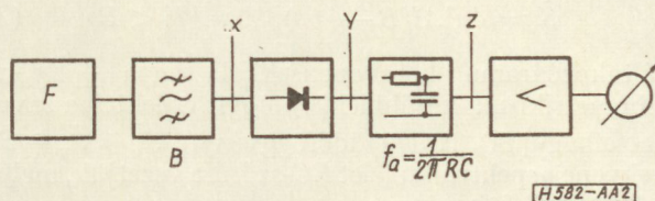
2. ábra. Közvetlen leolvasású zajmérő bloksémája
