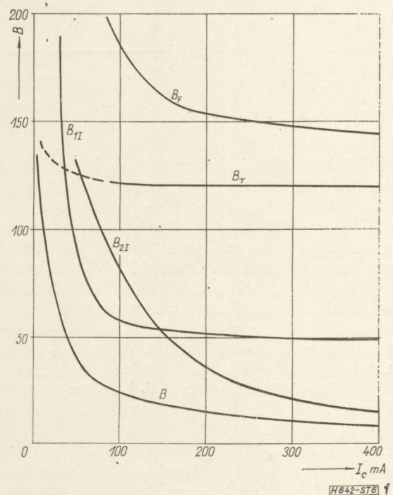
6. ábra. Az I. struktúránál K_e = 4,5 \cdot 10^{13} \frac{1}{cm^4 s} , a = 1000 cm/s, \tau_0 = 3 \mu s adatokkal számított B(I_c) függvény komponensei
