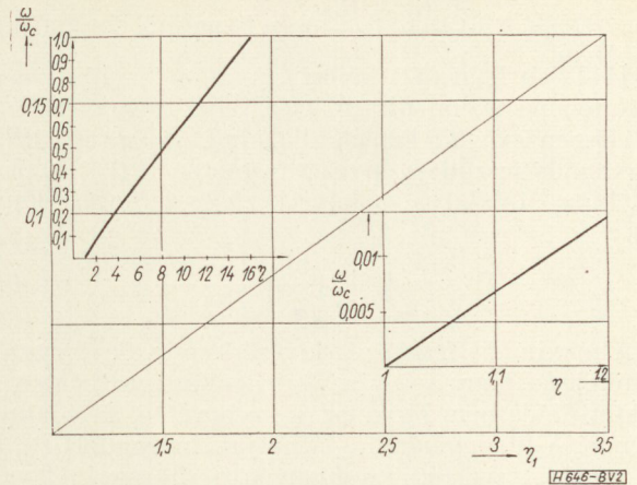
2. ábra. \frac{\omega}{\omega_c} az \eta_1 -függvényében
