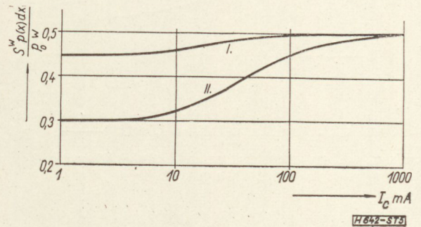
5. ábra. A_2 = \int_0^w p(x) dx ; T(I_c) görbék az I. és II. eloszlásnál a 2. és 3. ábrák alapján
