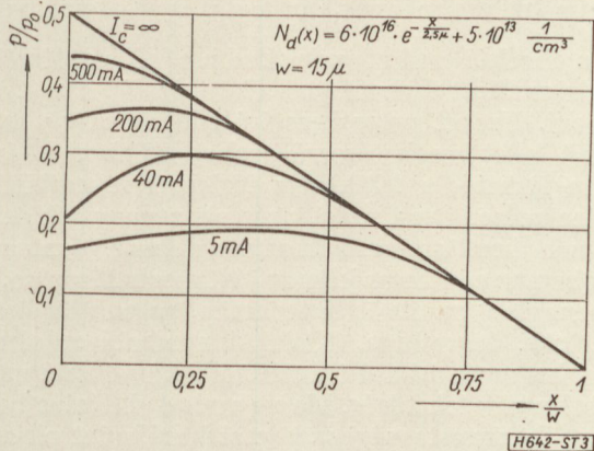
3. ábra. Az injektált lyukkonzentrációk a II. eloszlású bázisban a kollektoráram, mint paraméter mellett
