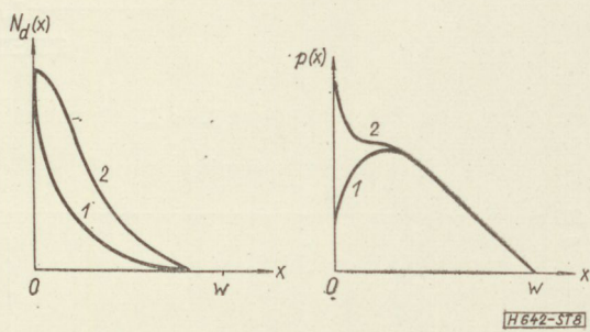
8. ábra. A donoreloszlás hatása az injektált töltéshordozó eloszlásra
