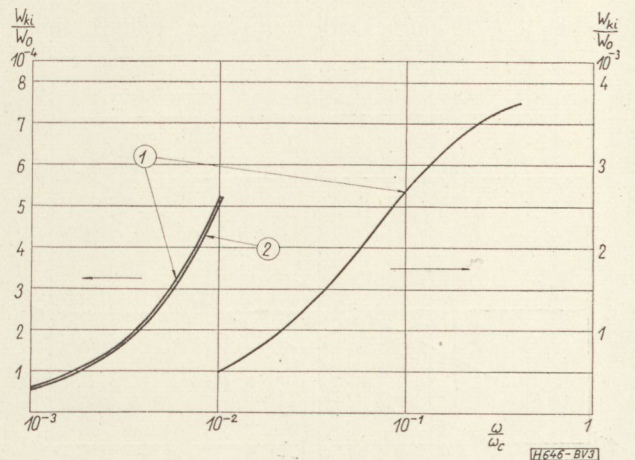
3. ábra. Normalizált kimenő teljesítmény \frac{\omega}{\omega_c} -függvényében. 1 — maximális normalizált teljesítmény teljes kivezérlés esetén; 2 — legnagyobb hatásfokhoz tartozó normálizált teljesítmény
