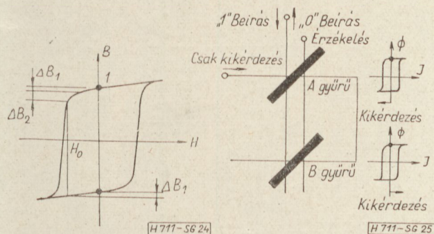
24. ábra. A reverzibilis indukciótörölés
