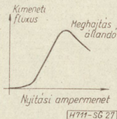
27. ábra. Transzfluxor karakterisztikája
