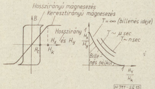
15. ábra. Mágneses vékonyréteg karakterisztikái
