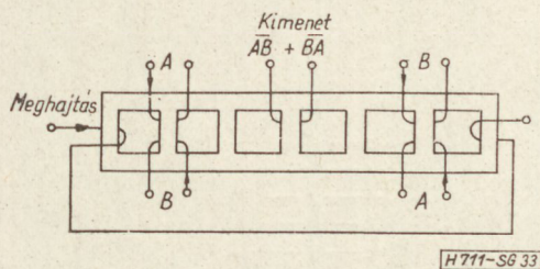
33. ábra. Kizárólagos vagy kapcsolás
