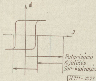
23. ábra. Négyszöghiszterézisgörbéjű ferritgyűrű működtetése állandó tárolóban
