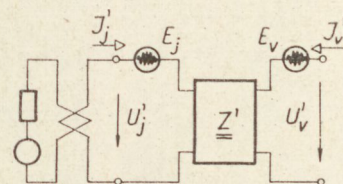
10. ábra. Áramkörü modell a zajtényező számításához
