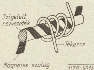
13. ábra. Twistor memóriaelem
