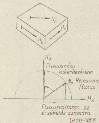
9. ábra. A biax működése
