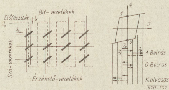
2. ábra. Szószervezésű memóriaelrendezés
