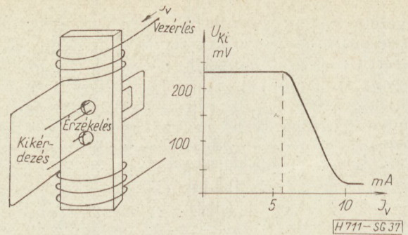
37. ábra. Ferrod-elem és karakterisztikája
