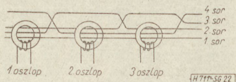
22. ábra. Átszámláló áramkör lineáris transzformátorokkal
