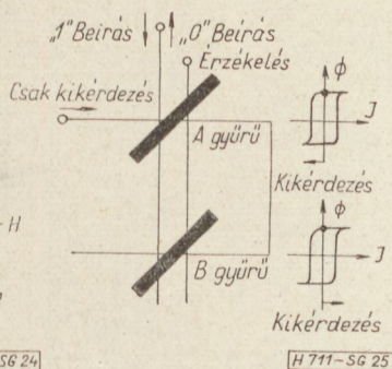
25. ábra. Elrendezés nem-törölő kiolvasáshoz
