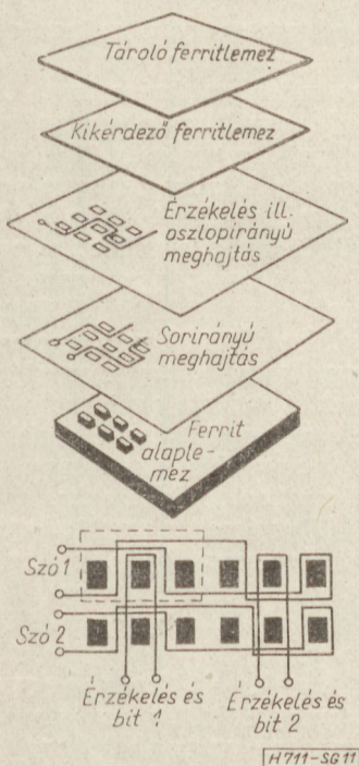
11. ábra. Ferritrács memóriafelépítése
