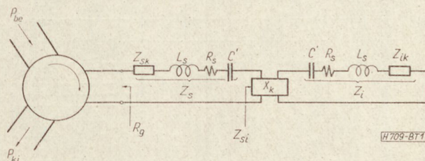
1. ábra. Parametrikus erősítő helyettesítő képe
