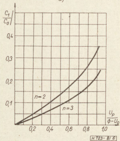
6. ábra. Dióda átlagos kapacitás és az ún. modulációs tényező függése a pump kivezérés mértékétől
