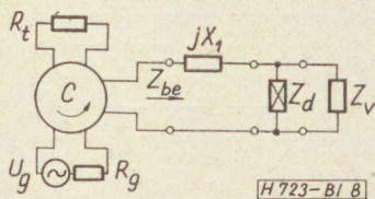
8. ábra. Negatív ellenállású, reflexiós erősítő áramkörti modellje
