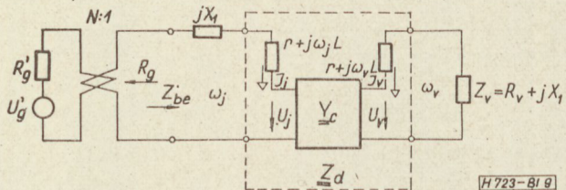
9. ábra. Az erősítő számításánál használt koncentrált paraméterű áramkörti modell ( Z_v = R_v + jX_v )
