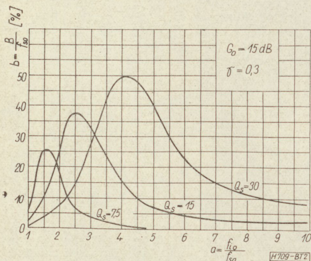
2. ábra. Relatív sávzélesség a különbségi frekvencia-jelfrekvencia hányados függvényében
