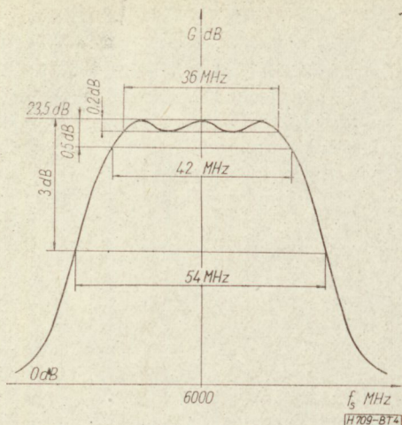
4. ábra. Kivitelezett parametrikus erősítő erősítés-frekvencia karakterisztikája
