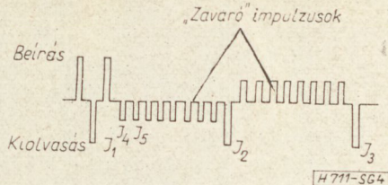
4. ábra. Impulzusprogram ferritgyűrűk vizsgálatához
